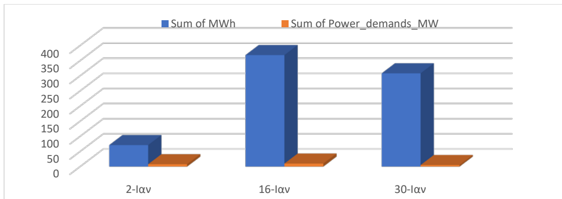
Διάγραμμα 3.4 : Αποτελέσματα Ιανουαρίου
