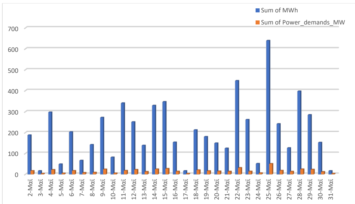
Διάγραμμα 3.8 : Αποτελέσματα Μαΐου
