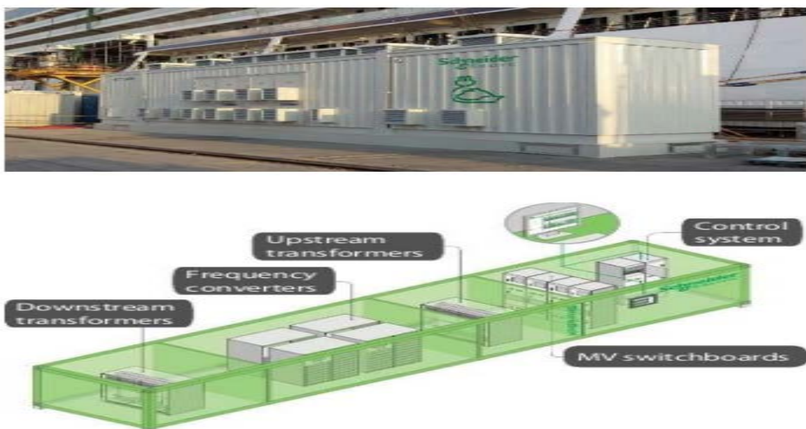
Εικόνα 2.4 : Προκατασκευασμένος υποσταθμός συστήματος OPS, πηγή [11]
