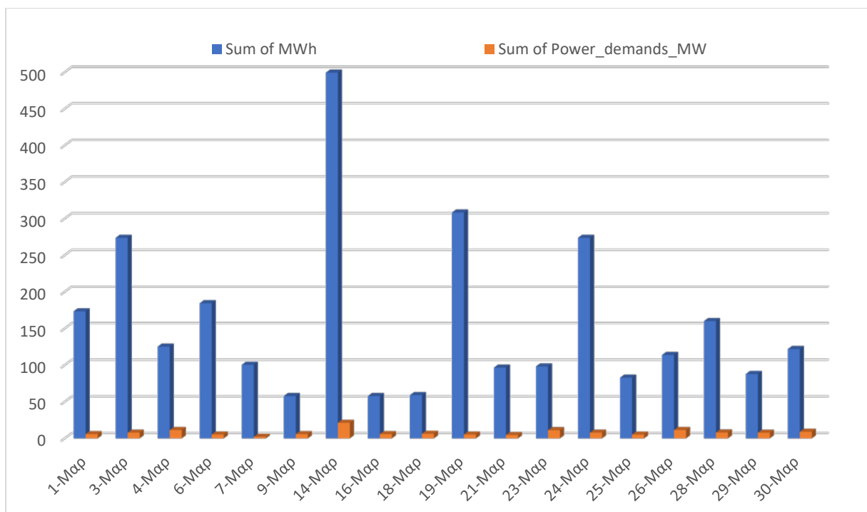
Διάγραμμα 3.6 : Αποτελέσματα Μαρτίου
