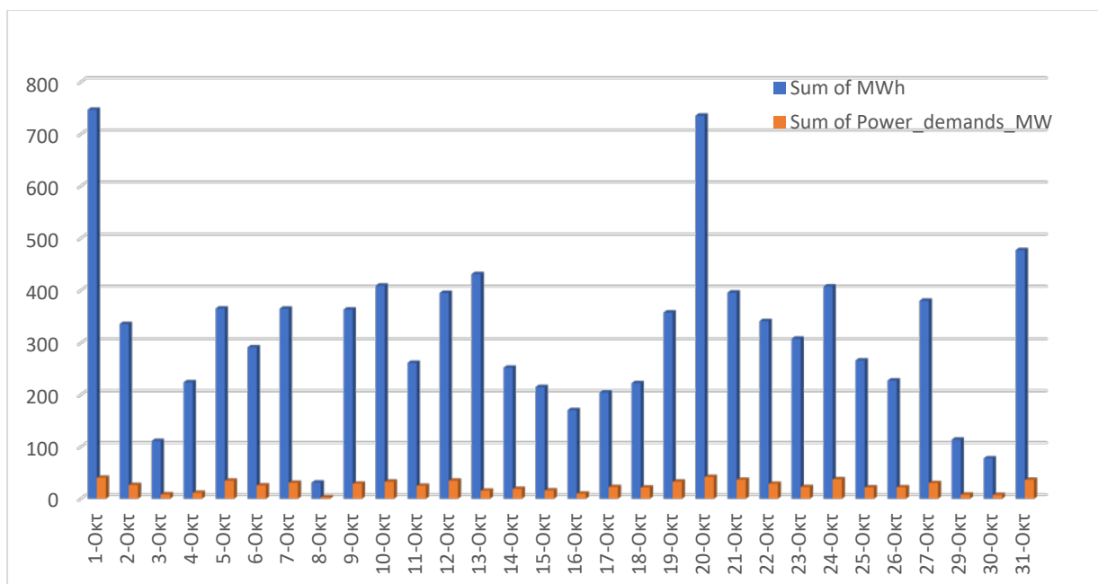
Διάγραμμα 3.13 : Αποτελέσματα Οκτωβρίου
