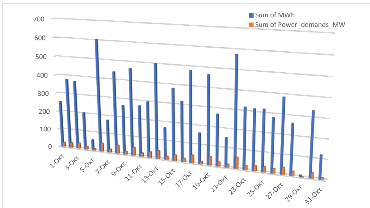
Διάγραμμα 3.23 : Αποτελέσματα Οκτωβρίου
