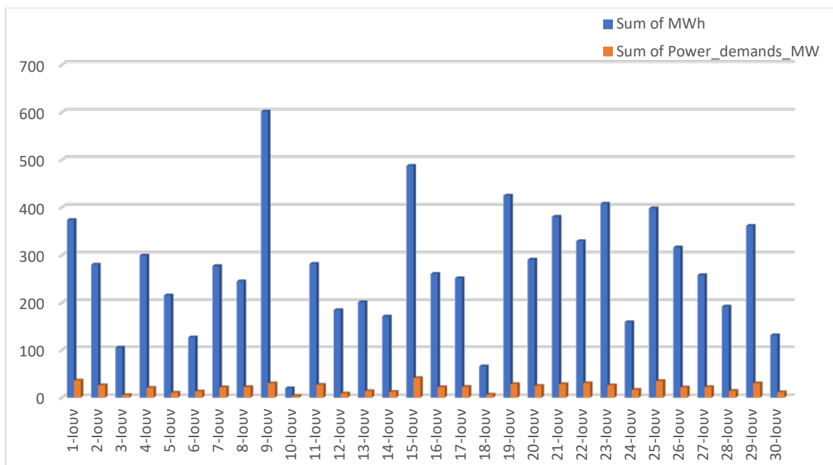
Διάγραμμα 3.9 : Αποτελέσματα Ιουνίου
