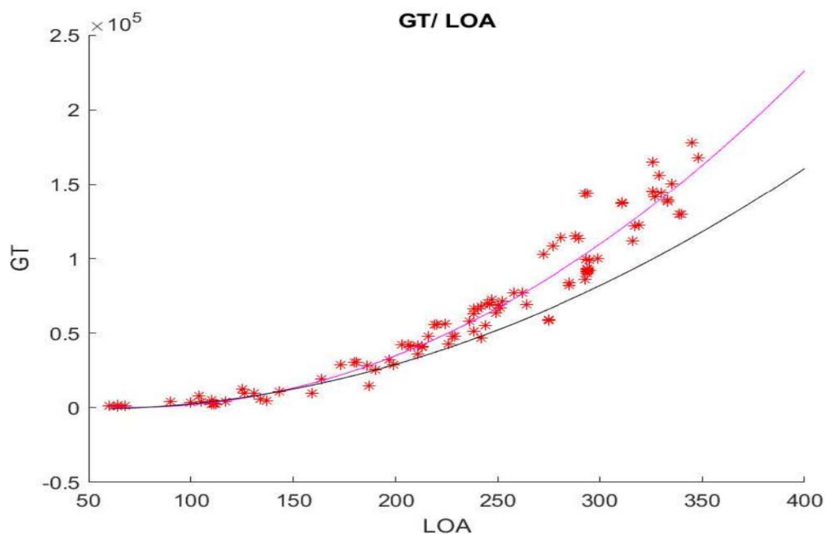
Διάγραμμα 3.1 : Gross Tonnage-Μήκος
