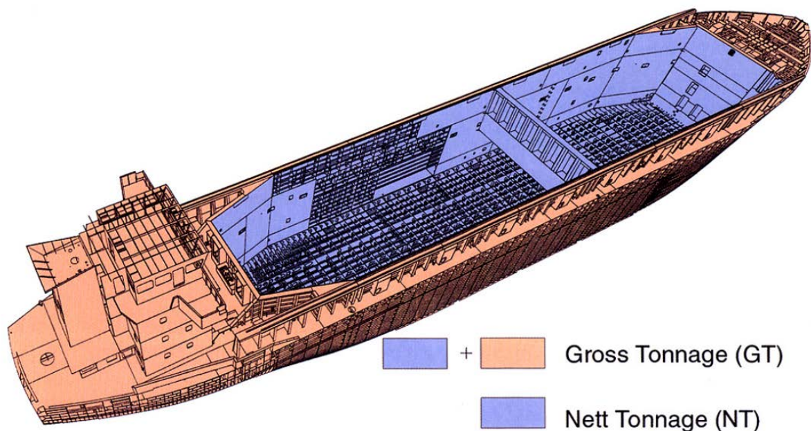
Εικόνα 1.1 : Η έννοια του Tonnage, πηγή [2]
