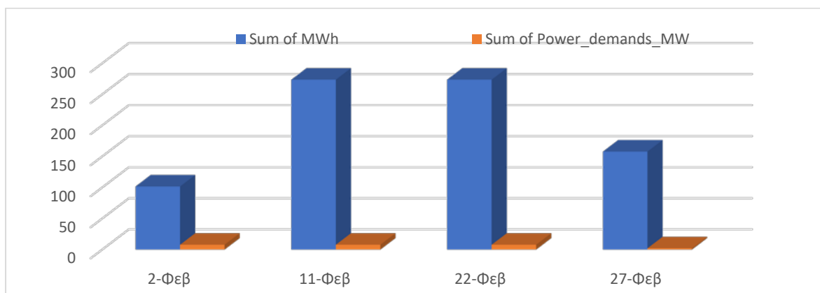
Διάγραμμα 3.5 : Αποτελέσματα Φεβρουαρίου
