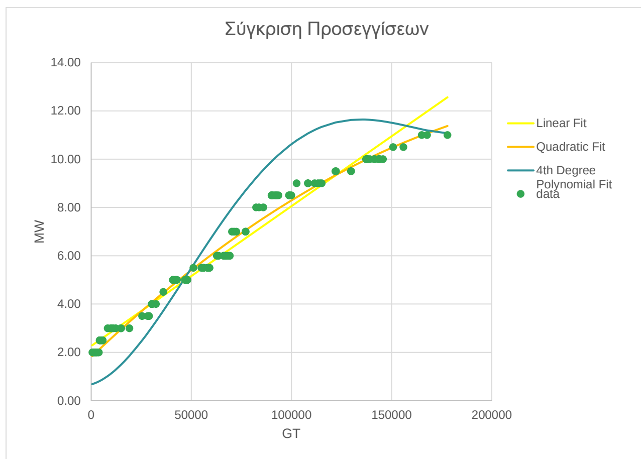
Διάγραμμα 3.3 : P-Gross Tonnage
