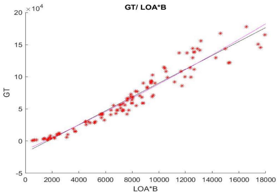
Διάγραμμα 3.2 : Gross Tonnage-Μήκος επί πλάτος
