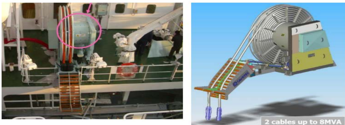
Εικόνα 2.11 : Εγκατάσταση πάνω στο πλοίο , πηγή [10]
