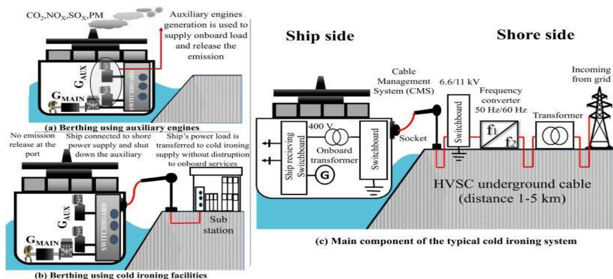
Εικόνα 2.1 : Προτεινόμενη διάταξη, πηγή [4]
