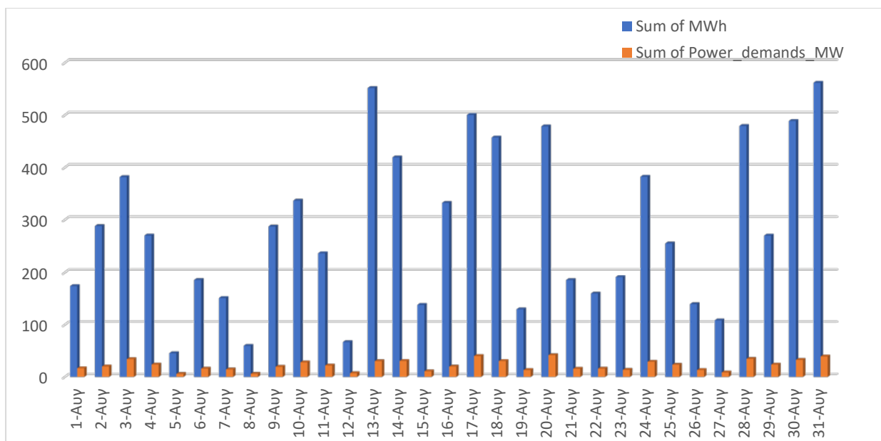
Διάγραμμα 3.11 : Αποτελέσματα Αυγούστου
