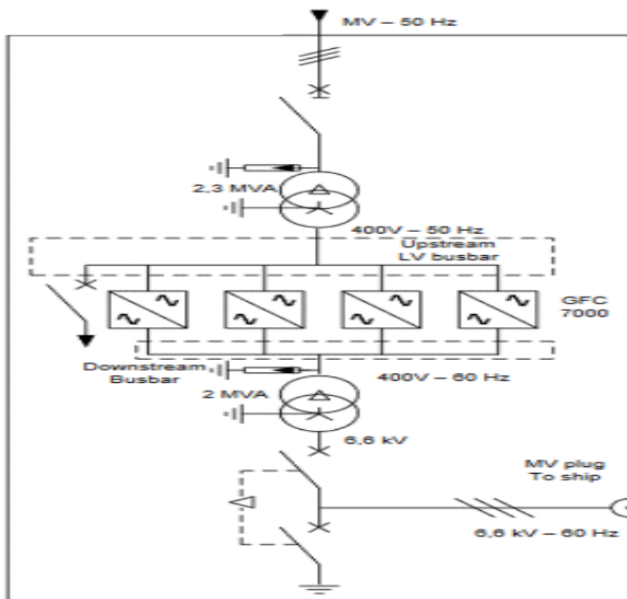
Εικόνα 2.5 : Μονογραμμικό διάγραμμα, πηγή [12]
