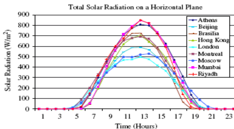
Διάγραμμα 14: 24ωρο προφίλ της ολικής ηλιακής ακτινοβολίας σε οριζόντιο επίπεδο, για το ζεστότερο μήνα κάθε πόλης [82]
