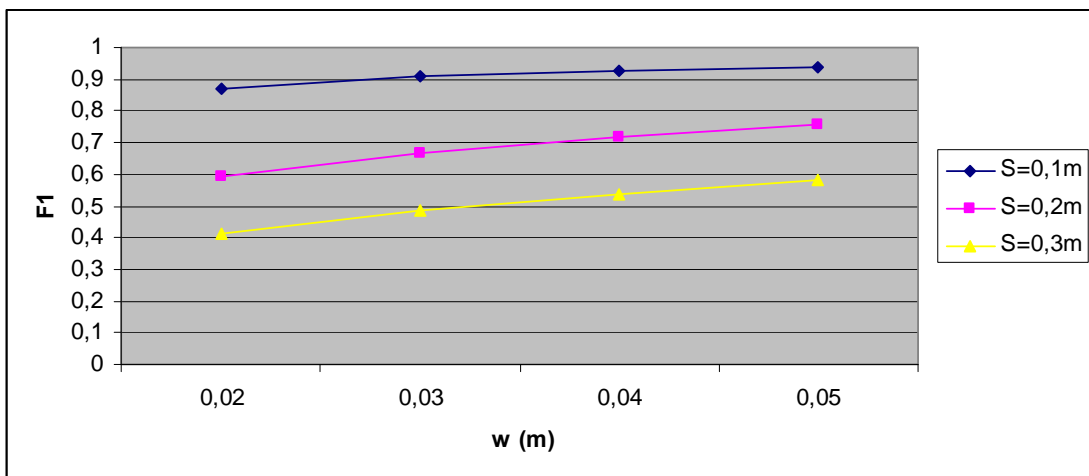
Διάγραμμα 35: Εξάρτηση του παράγοντα απόδοσης F_1 από το πάχος του πάνελ w , με παράμετρο την απόσταση των αγωγών S , για h = 10 \text{ W m}^{-2} \text{ } ^\circ\text{C}^{-1} , διαμέτρους D_o = 0,02 \text{ m} , D_i = 0,018 \text{ m} , συντελεστή
