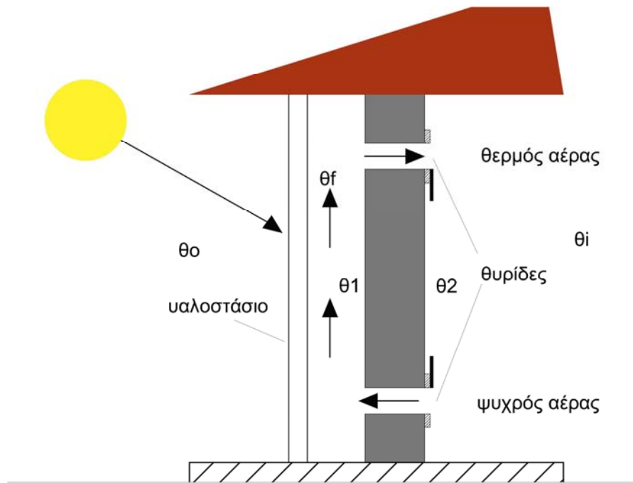
Εικόνα 22: Τοίχος Trombe
