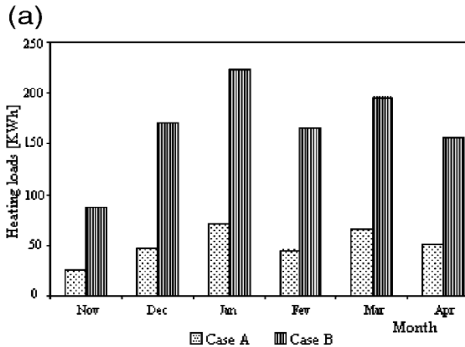
Διάγραμμα 12: Μηνιαία φορτία για θέρμανση για την περίπτωση του συνδυασμού τοίχου BC-βοηθητική συσκευή θέρμανσης (Περίπτωση A) και για ένα συμβατικό σύστημα θέρμανσης (Περίπτωση B) [64]
