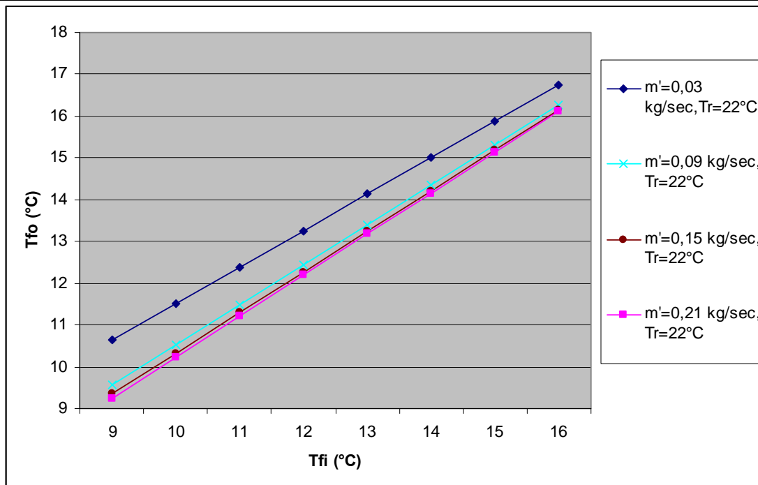
Διάγραμμα 40: Η θερμοκρασία εξόδου T_{f_o} του ρευστού από το σωλήνα, σε συνάρτηση με την θερμοκρασία εισόδου του T_{f_i} , για διαφορετικές παροχές μάζας m' (Πίνακας 50) και θερμοκρασία T_r=22^\circ\text{C} του εσωτερικού αέρα, για c_p=4184\text{ J/kg}^\circ\text{C} , n=4 αγωγοί, μήκους L=3\text{m} , απόσταση S=0,2\text{m} , h=10\text{ W m}^{-2}\text{ }^\circ\text{C}^{-1} , διαμέτρους D_o=0,016\text{ m} , D_i=0,014\text{ m} , w=0,04\text{m} και F_1=0,702827 (από εξίσωση 9.2.5.6.).
