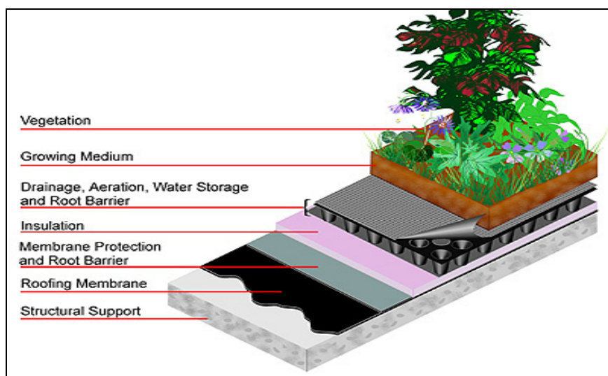
Εικόνα 63: Διαστρωμάτωση φυτεμένου δώματος [80]
