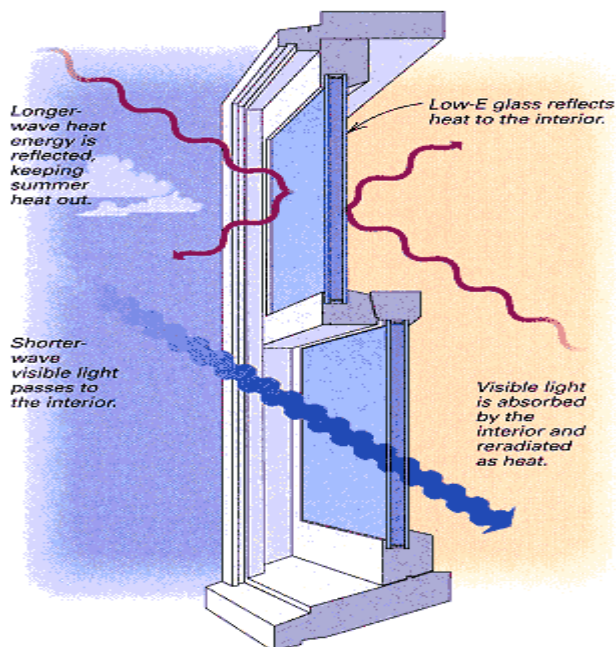
Εικόνα 51: Τα κρύσταλλα χαμηλής εκπομπής αντανακλούν τη θερμική ενέργεια, ενώ επιτρέπουν τη διέλευση του ορατού φωτός. Έτσι, το καλοκαίρι αποφεύγεται η υπερθέρμανση του χώρου, ενώ το χειμώνα, η ηλιακή ορατή ακτινοβολία, που σχηματίζει χαμηλότερη γωνία, εισέρχεται στο εσωτερικό και απορροφάται ως θερμότητα [71]
