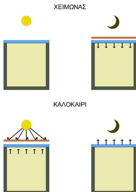
Εικόνα 31: Ηλιακή Λίμνη.
