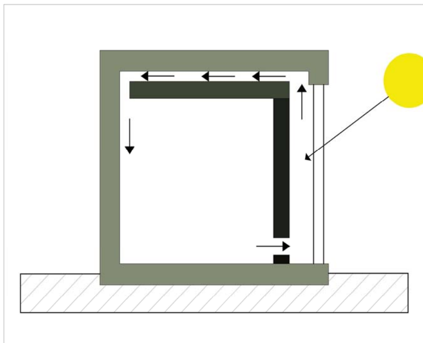
Εικόνα 29: Τοίχος Barra-Constantini
