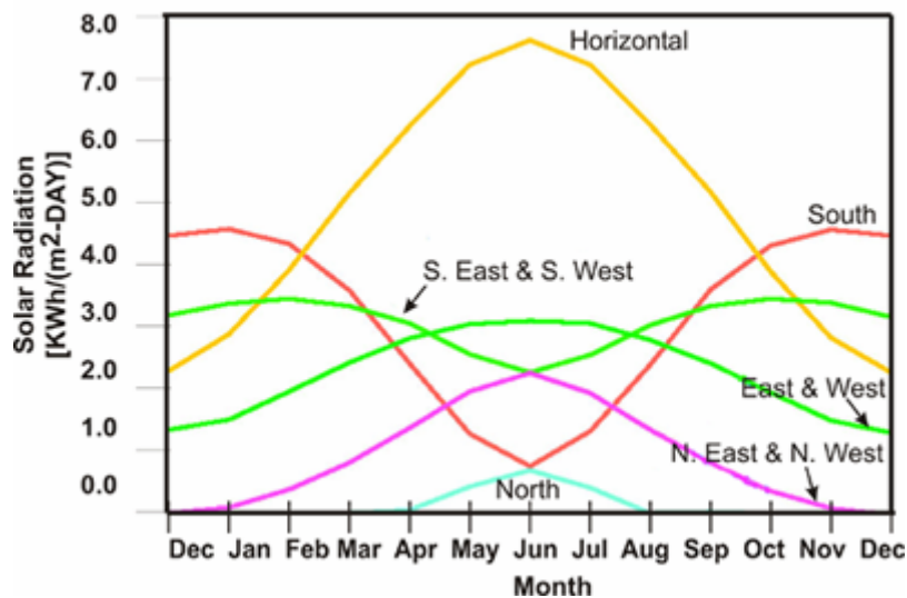
Διάγραμμα 13: Ηλιακή Ακτινοβολία για διάφορους προσανατολισμούς [22]
