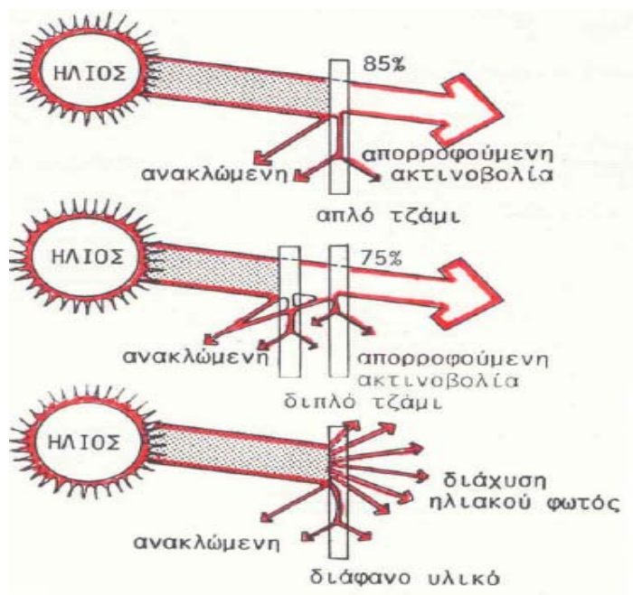
Εικόνα 13: Είσοδος της ηλιακής ακτινοβολίας μέσα από τζάμι [20]
