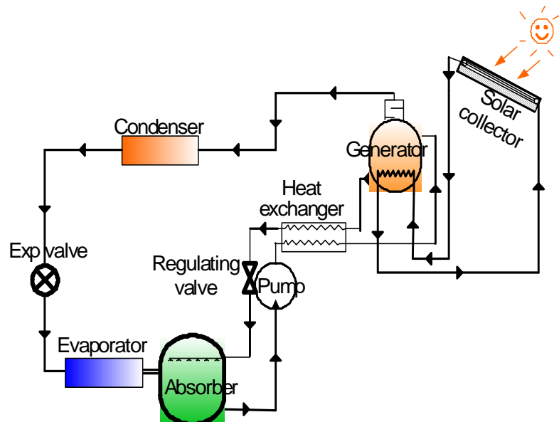
Εικόνα 102: Διαδικασία ηλιακού κλιματισμού με απορρόφηση. Αποτελείται από το ηλιακό συλλέκτη, τον συμπυκνωτή, την εκτονωτική βαλβίδα, τον ατμοποιητή και τη μονάδα απορρόφησης, η οποία μαζί με τη γεννήτρια (αναγεννητής) και ένα σύστημα που συνίσταται από τον εναλλάκτη, μια αντλία και τη ρυθμιστική βαλβίδα, παίζει το ρόλο του συμπιεστή [106].
