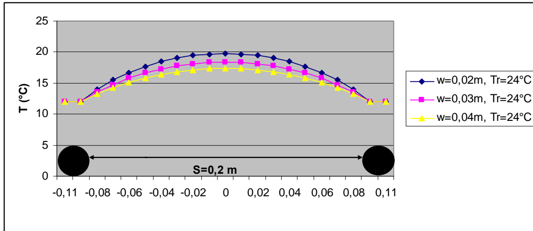
Διάγραμμα 26: Κατανομή θερμοκρασίας μεταξύ των σωλήνων για θερμοκρασίες χώρου T_r=24\text{ }^\circ\text{C} , S=0,2\text{m} , w=0,02\text{m} , 0,03\text{m} , 0,04\text{m} , h=10\text{ W m}^{-2}\text{ }^\circ\text{C}^{-1} , k=1,4\text{ W m}^{-1}\text{ }^\circ\text{C}^{-1} , T_o=12\text{ }^\circ\text{C} , D_o=0,02\text{ m} . Θεωρώ x=0 , το μέσο της απόστασης των αξόνων των δύο σωλήνων. (οι αρνητικές τιμές προκύπτουν συμβολικά, επειδή θεωρώ ως 0 το μέσο της απόστασης των αγωγών )
