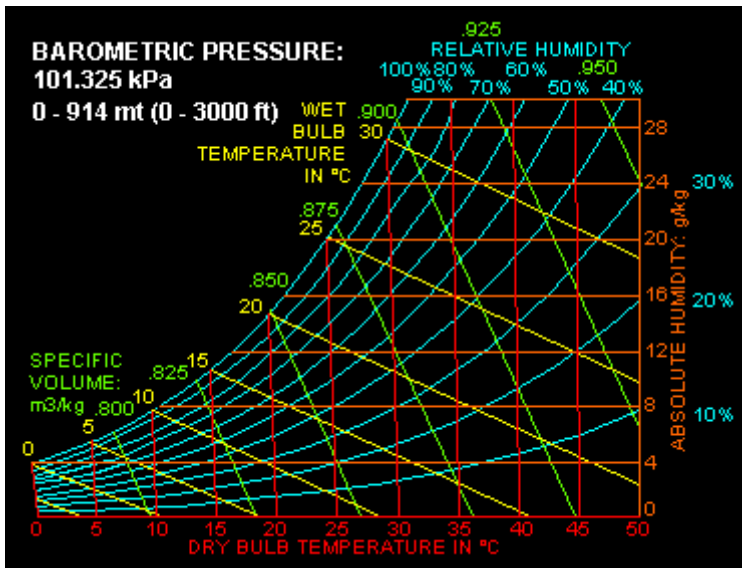
Διάγραμμα 1: Ψυχομετρικό Διάγραμμα [17]
