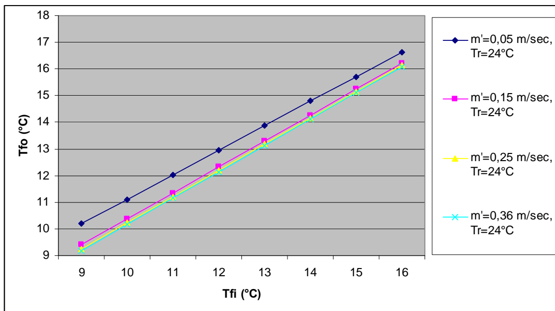
Διάγραμμα 37: Η θερμοκρασία εξόδου T_{f,o} του ρευστού από το σωλήνα, σε συνάρτηση με την θερμοκρασία εισόδου του T_{f,i} , για διαφορετικές παροχές μάζας m' και θερμοκρασία T_r=24^\circ\text{C} του εσωτερικού αέρα, για c_p=4184\text{ J/kg }^\circ\text{C} , n=4 αγωγοί, μήκους L=3\text{m} , απόσταση S=0,2\text{m} , h=10\text{ W m}^{-2}\text{ }^\circ\text{C}^{-1} , k=1,4\text{ W m}^{-1}\text{ }^\circ\text{C}^{-1} , διαμέτρους D_o=0,02\text{ m} , D_i=0,018\text{ m} , w=0,04\text{m} και F_1=0,718321 (από Πίνακα 43).
