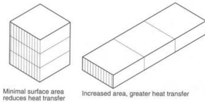
Εικόνα 39: Σχήμα κτηρίου και μεταφορά θερμότητας [22]
