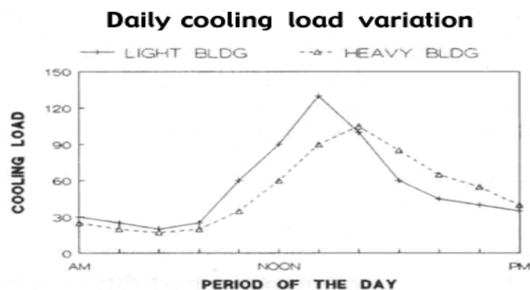
Διάγραμμα 4: Διακόμανση του ψυκτικού φορτίου κατά τη διάρκεια της ημέρας για μικρή και μεγάλη θερμική μάζα [22]
