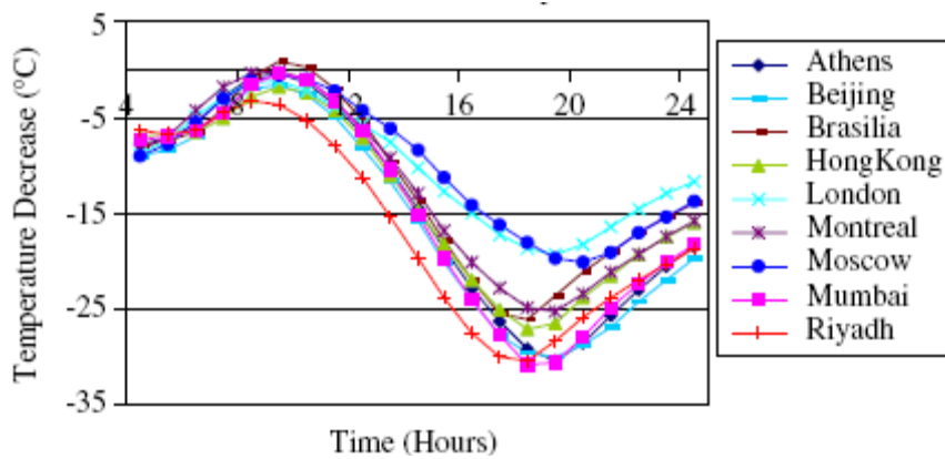
Διάγραμμα 16 : Πτώση της θερμοκρασίας της επιφάνειας της στέγης όταν καλύπτεται με βλάστηση, για διάφορες πόλεις
