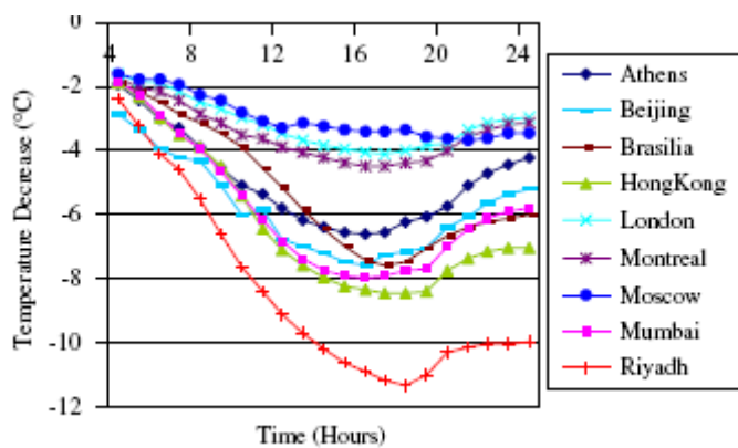
Διάγραμμα 17: Η μείωση της θερμοκρασίας μέσα στο «αστικό φαράγγι» όταν καλύπτονται με βλάστηση τόσο οι στέγες, όσο και οι τοίχοι, για διάφορες κλιματικές ζώνες.
