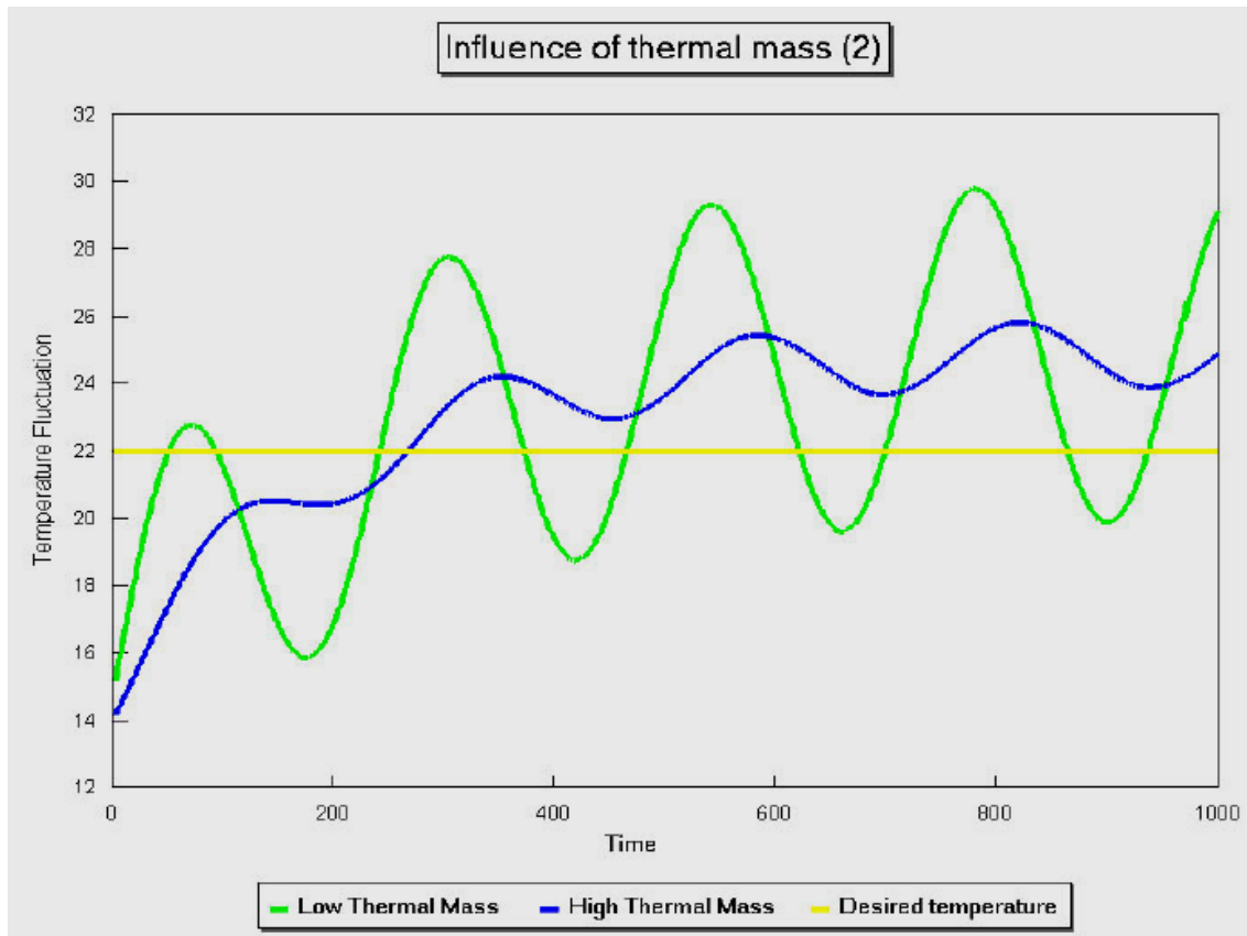
Διάγραμμα 6: Επίδραση της θερμικής μάζας [22].
