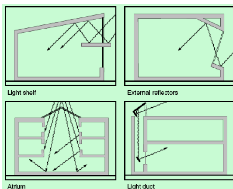
Εικόνα 80: Μερικά από τα συστήματα φυσικού φωτισμού. Πάνω σειρά από αριστερά:ράφια φωτισμού, εξωτερικοί ανακλαστής. Κάτω σειρά από αριστερά: αίθριο, φωταγωγός [26]
