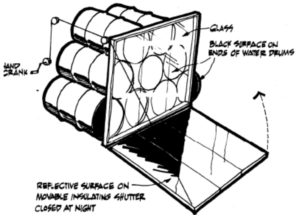
Εικόνα 28: Τοίχος νερού [23]
