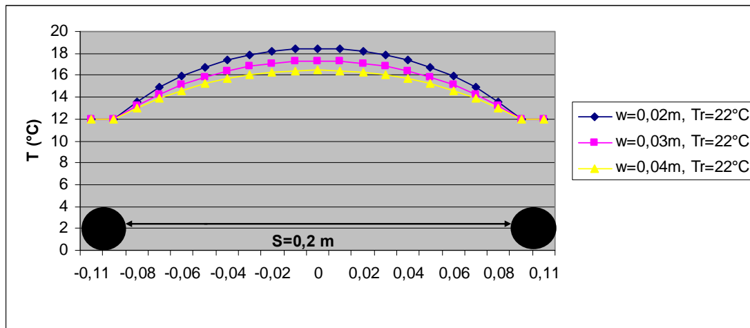
Διάγραμμα 25: Κατανομή θερμοκρασίας μεταξύ των σωλήνων για θερμοκρασίες χώρου T_r=22\text{ }^\circ\text{C} , S=0,2\text{m} , w=0,02\text{m} , 0,03\text{m} , 0,04\text{m} , h=10\text{ W m}^{-2}\text{ }^\circ\text{C}^{-1} , k=1,4\text{ W m}^{-1}\text{ }^\circ\text{C}^{-1} , T_o=12\text{ }^\circ\text{C} , D_o=0,02\text{ m} . Θεωρώ x=0 , το μέσο της απόστασης των αξόνων των δύο σωλήνων.. (οι αρνητικές τιμές προκύπτουν συμβολικά, επειδή θεωρώ ως 0 το μέσο της απόστασης των αγωγών )
