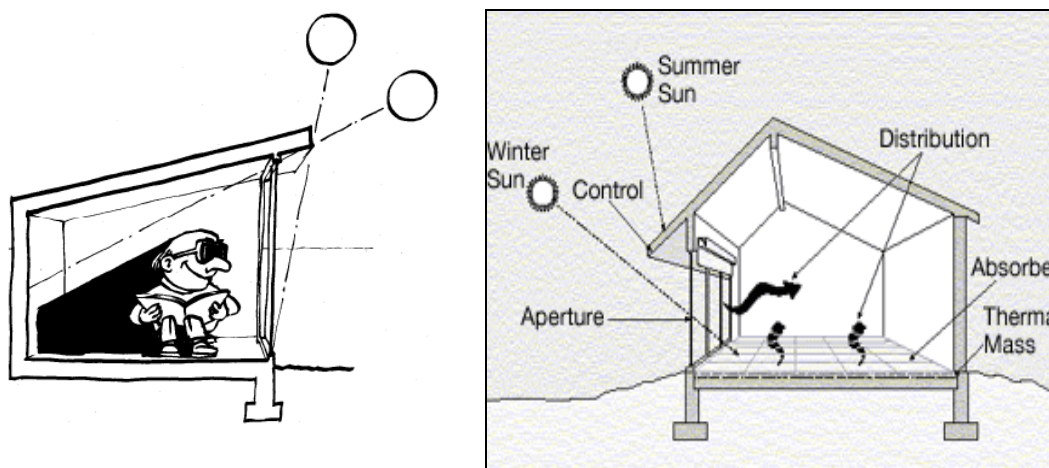
Εικόνα 6: Συστήματα άμεσου κέρδους [21]
