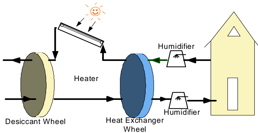
Εικόνα 104: Ηλιακός κλιματισμός με αφύγρανση [106]
