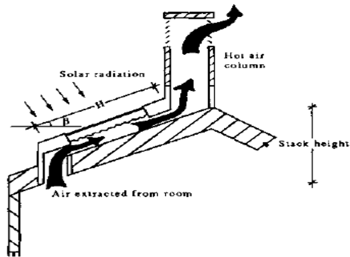
Εικόνα 72: Ηλιακή Καμινάδα
