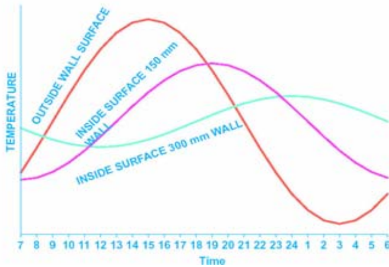
Διάγραμμα 8: Διακύμανση της θερμοκρασίας του τοίχου, λόγω χρονικής υστέρησης [22]
