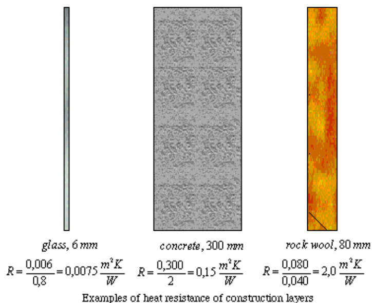
Εικόνα 10: Παραδείγματα θερμικής αντίστασης στρωμάτων της τοιχοποιίας [22]
