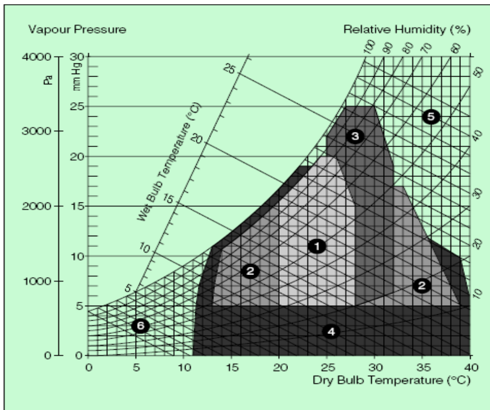
Διάγραμμα 2: Ένδειξης θερμικής άνεσης σε συνθήκες εσωτερικού χώρου. 1. Ζώνη Θερμικής Άνεσης, 2. Ζώνη εφαρμογής παθητικών συστημάτων θέρμανσης 3. Ζώνη Ανάγκης Αερισμού, 4. Ζώνη επίδρασης στους χρήστες 5. Ζώνη ανάγκης μηχανικής ψύξης, 6. Ζώνη Ανάγκης Θέρμανσης [26]
