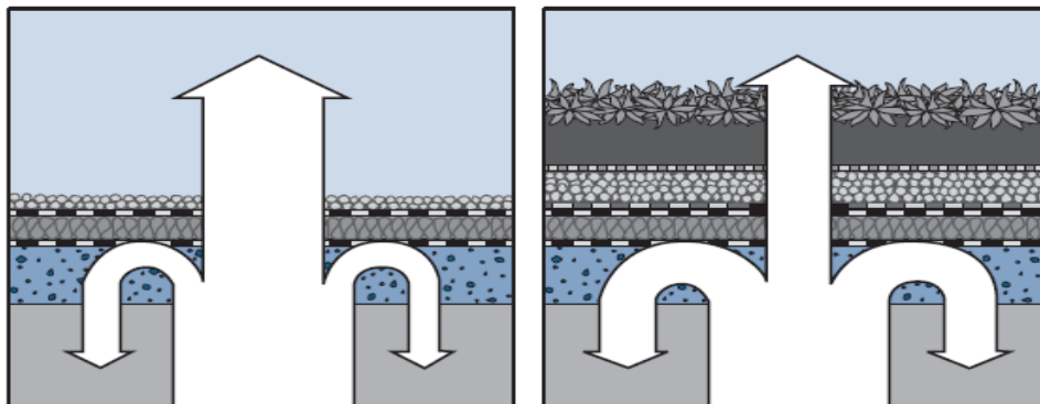
Εικόνα 65: Ροή θερμότητας δια μέσου, στέγης χαλικοστρωμένης και «πράσινης» οροφής. Στη δεύτερη περίπτωση η θερμική μάζα του φυτεμένου δώματος αποτρέπει ένα μεγάλο ποσό θερμότητας να διαφύγει [44]
