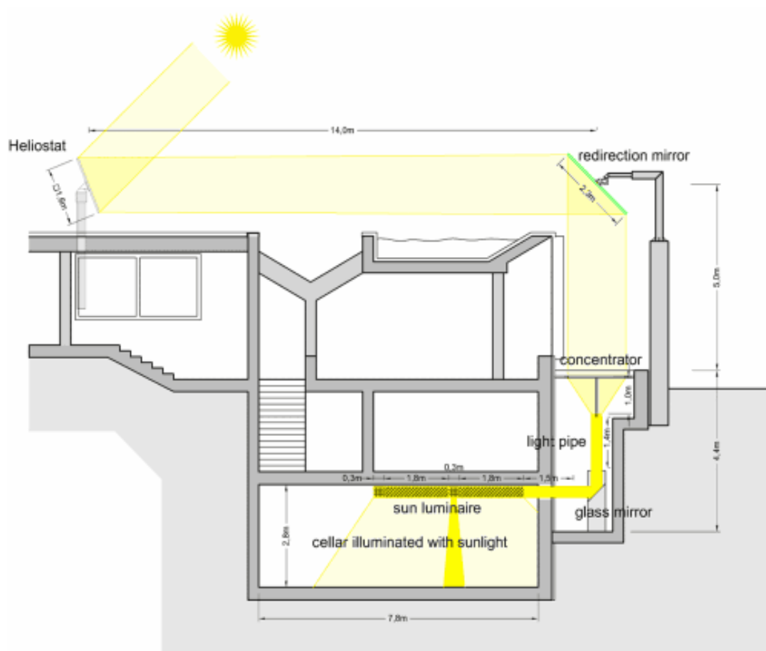
Εικόνα 83: Χρήση ηλιοστασίων για φυσικό φωτισμό [22]
