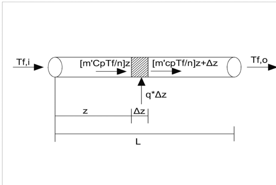
Εικόνα 112: Ενεργειακή ισορροπία σε ένα στοιχείο \Delta z του ψυκτικού ρευστού.
