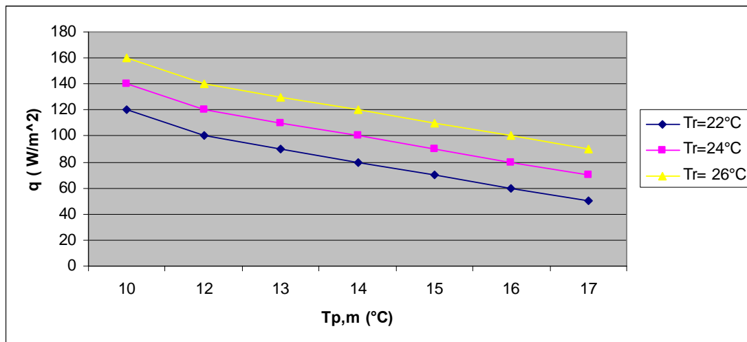
Διάγραμμα 47: Η θερμότητα q που απορροφάται ανά μονάδα επιφάνειας του πάνελ, σε σχέση με τη μέση θερμοκρασία του πάνελ T_{p,m} , για διάφορες θερμοκρασίες εσωτερικού αέρα T_r
