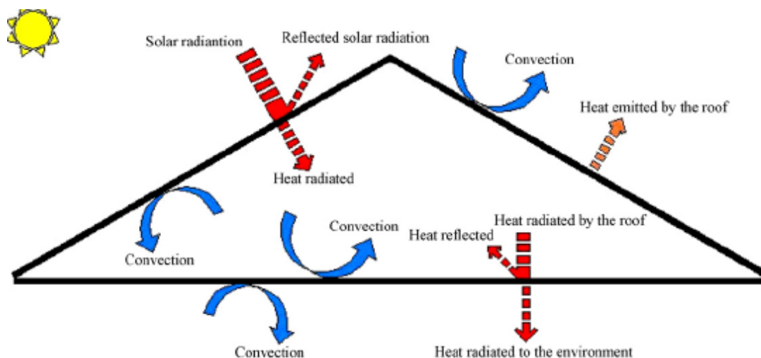
Εικόνα 55: Μετάδοση θερμότητας προς την στέγη κτηρίου [76]
