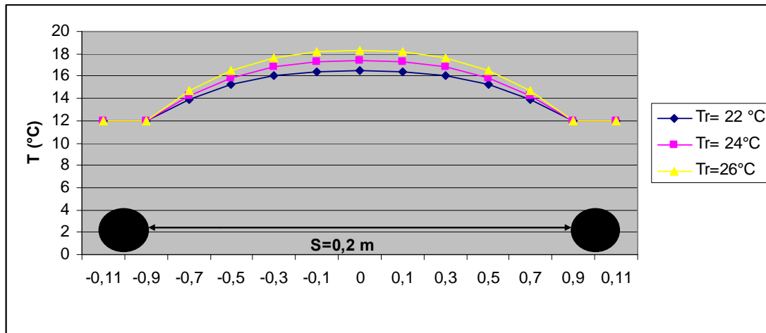
Διάγραμμα 23: Κατανομή της θερμοκρασίας μεταξύ των σωλήνων του πάνελ για S=0,2m , w=0,04m , h=10W m^{-2} °C^{-1} , k=1,4W m^{-1} °C^{-1} , T_o=12°C , D_o=0,02m , για T_r=22°C, 24°C, 26°C . (οι αρνητικές τιμές προκύπτουν συμβολικά, επειδή θεωρώ ως 0 το μέσο της απόστασης των αγωγών )
