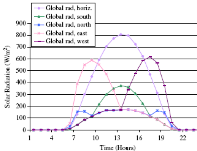
Διάγραμμα 15: Πρόσπτωση της ηλιακής ακτινοβολίας σε οριζόντιο επίπεδο και κατακόρυφο επίπεδο για νότιο, βόριο, ανατολικό και δυτικό προσανατολισμό για το μήνα Ιούλιο [82]
