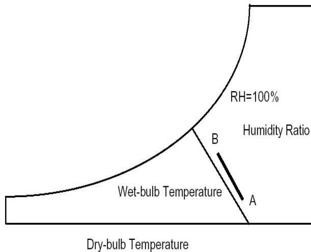
Διάγραμμα 18: Άμεσος δροσισμός από εξάτμιση. Ο αέρας που πρόκειται να ψυχθεί βρίσκεται αρχικά στο σημείο A, ενώ λόγω της άμεσης εξάτμισης, ψύχεται και φτάνει στο σημείο B. Η διαδικασία γίνεται υπό σταθερή θερμοκρασία υγρής σφαίρας, δηλαδή έχουμε πτώση της θερμοκρασίας του αέρα, με παράλληλη αύξηση της υγρασίας του [22]
