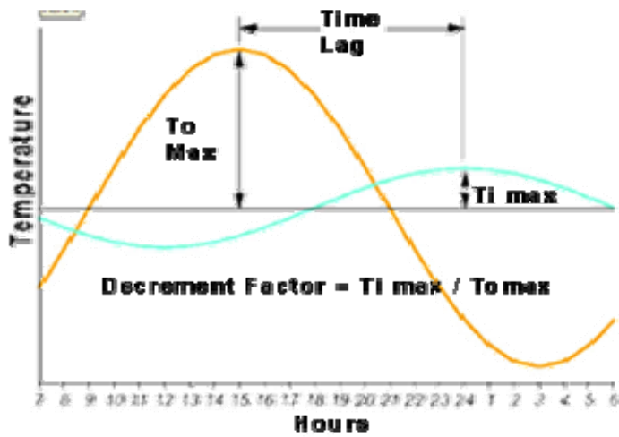
Διάγραμμα 9: Χρονική Υστέρηση. Ο παράγων μείωσης είναι ίσος με T_{i\max}/T_{o\max} (Decrement Factor) [22].
