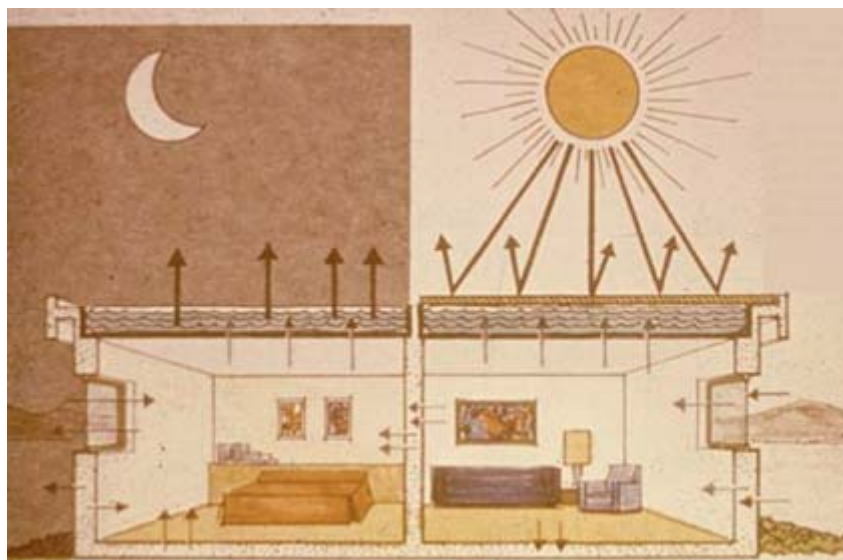
Εικόνα 30: Λειτουργία ηλιακής λίμνης το καλοκαίρι [65]
