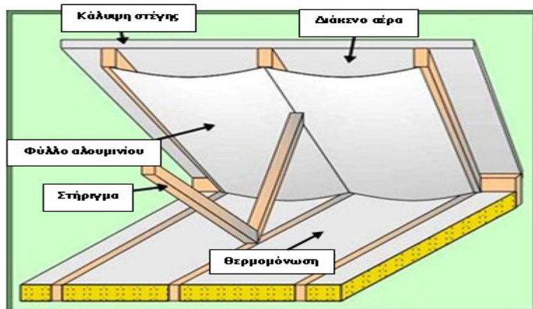
Εικόνα 57: Φράγμα Ακτινοβολίας [22]
