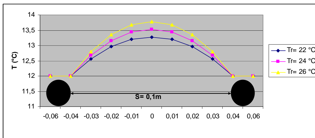
Διάγραμμα 22: Κατανομή της θερμοκρασίας μεταξύ των σωλήνων του πάνελ για S=0,1\text{m} , w=0,04\text{ m} , h=10\text{ W m}^{-2}\text{ }^\circ\text{C}^{-1} , k=1,4\text{ W m}^{-1}\text{ }^\circ\text{C}^{-1} , T_o=12\text{ }^\circ\text{C} , D_o=0,02\text{ m} , για T_r=22\text{ }^\circ\text{C} , 24\text{ }^\circ\text{C} , 26\text{ }^\circ\text{C} . (οι αρνητικές τιμές προκύπτουν συμβολικά, επειδή θεωρώ ως 0 το μέσο της απόστασης των αγωγών)
