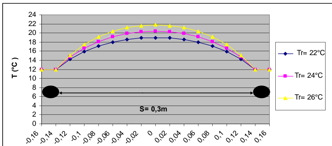
Διάγραμμα 24: Κατανομή της θερμοκρασίας μεταξύ των σωλήνων του πάνελ για S=0,3m , w=0,04m , h=10Wm^{-2}^{\circ}C^{-1} , k=1,4Wm^{-1}^{\circ}C^{-1} , T_o=12^{\circ}C , D_o=0,02m , για T_r=22^{\circ}C , 24^{\circ}C , 26^{\circ}C . (οι αρνητικές τιμές προκύπτουν συμβολικά, επειδή θεωρώ ως 0 το μέσο της απόστασης των αγωγών)
