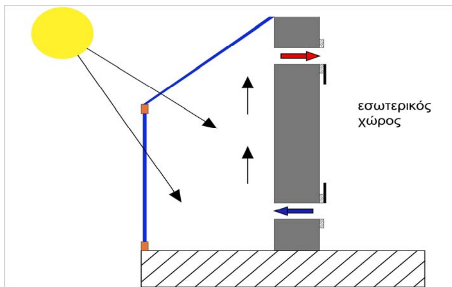
Εικόνα 32: Λειτουργία Θερμοκηπίου
