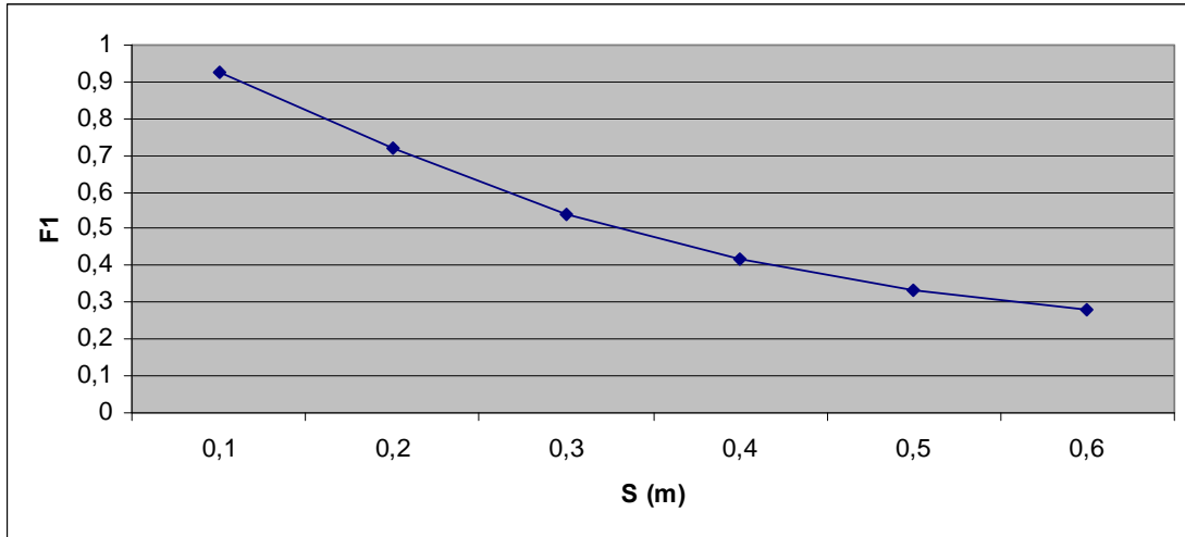
Διάγραμμα 34 Εξάρτηση του παράγοντα απόδοσης F_1 από την απόσταση των αγωγών S , για h = 10 \text{ W m}^{-2} \text{ } ^\circ\text{C}^{-1} , διαμέτρους D_o = 0,02 \text{ m} , D_i = 0,018 \text{ m} και συντελεστή μεταφοράς θερμότητας της εσωτερικής επιφάνειας του σωλήνα h_i = 3000 \text{ W m}^{-2} \text{ } ^\circ\text{C}^{-1} , με k = 1,4 \text{ W m}^{-1} \text{ } ^\circ\text{C}^{-1} και w = 0,04 \text{ m}
