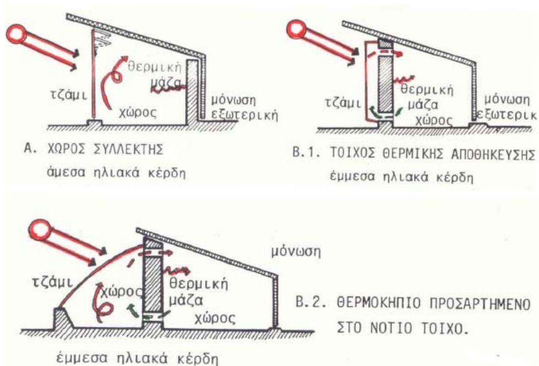
Εικόνα 5: Ηλιακά Παθητικά Συστήματα [20]
