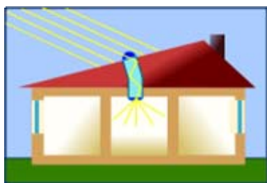
Εικόνα 85: Φωτοσωλήνας
