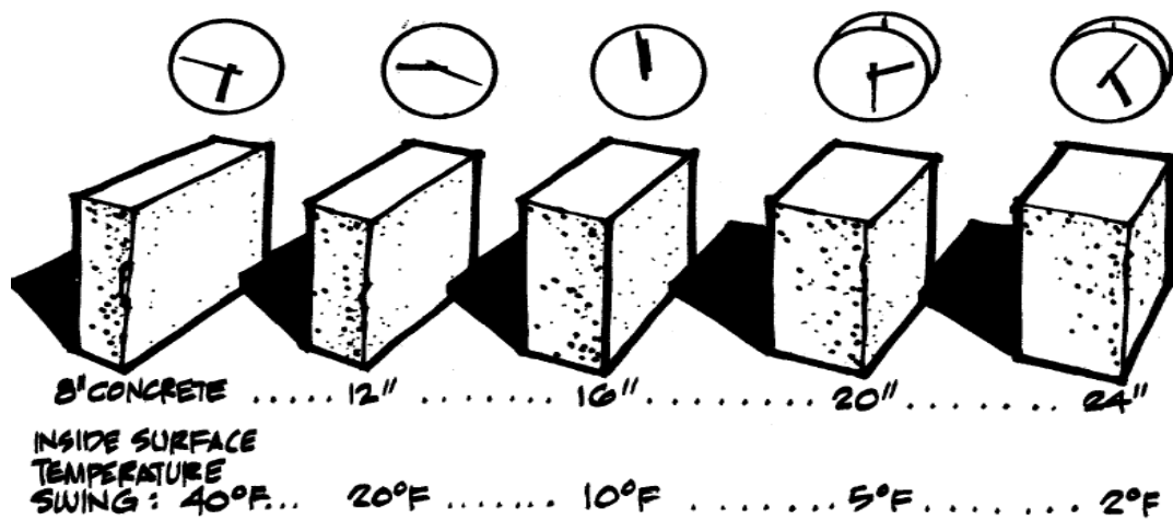
Διάγραμμα 9: Χρονική Υστέρηση. Ο παράγων μείωσης είναι ίσος με T_{i\max}/T_{o\max} (Decrement Factor) [22].
