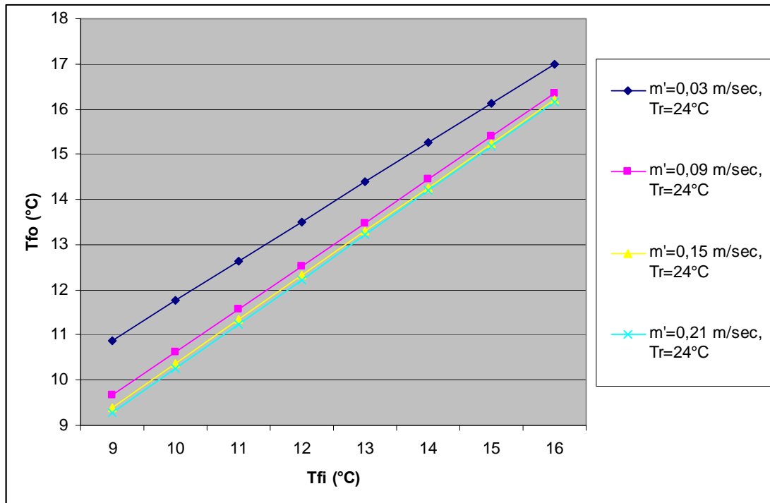
Διάγραμμα 41: Η θερμοκρασία εξόδου T_{f,o} του ρευστού από το σωλήνα, σε συνάρτηση με την θερμοκρασία εισόδου του T_{f,i} , για διαφορετικές παροχές μάζας m' (Πίνακας 49) και θερμοκρασία T_r=24^\circ\text{C} του εσωτερικού αέρα, για c_p=4184\text{ J/kg}^\circ\text{C} , n=4 αγωγοί, μήκους L=3\text{m} , απόσταση S=0,2\text{m} , h=10\text{ W m}^{-2}\text{ }^\circ\text{C}^{-1} , k=1,4\text{ W m}^{-1}\text{ }^\circ\text{C}^{-1} , διαμέτρους D_o=0,016\text{ m} , D_i=0,014\text{ m} , w=0,04\text{m} και F_1=0,702827 (από εξίσωση 9.2.5.6.).
