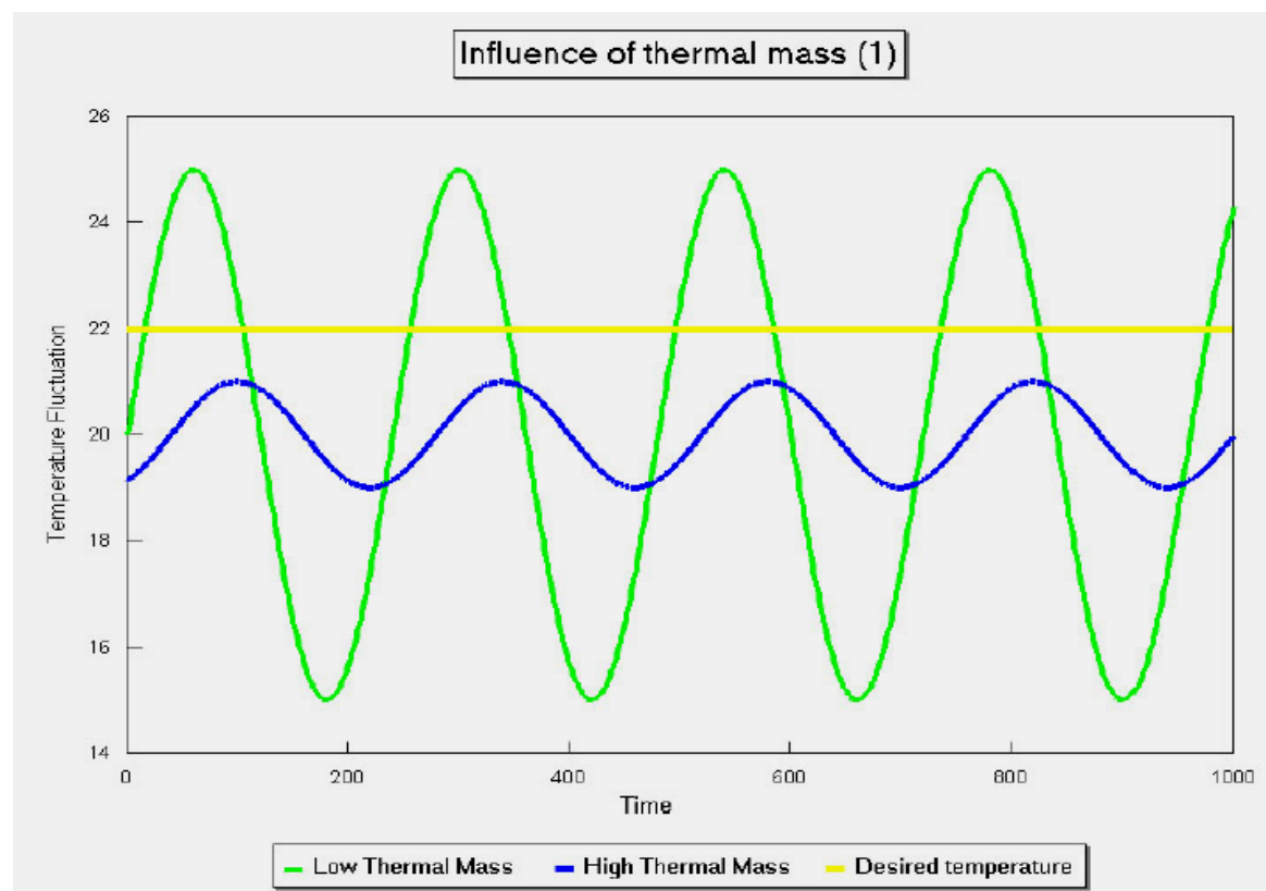
Διάγραμμα 5: Επίδραση της θερμικής μάζας [22].
