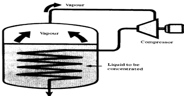
Σχήμα 1: Μηχανικός συμπιεστής ατμού [109]
