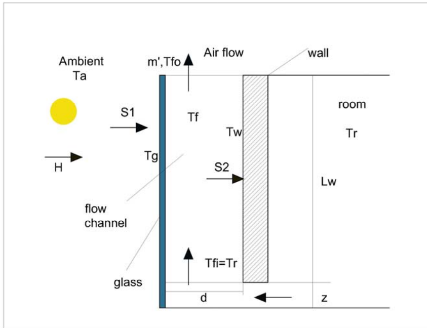
Εικόνα 73: Λειτουργία Ηλιακής καμινάδας
