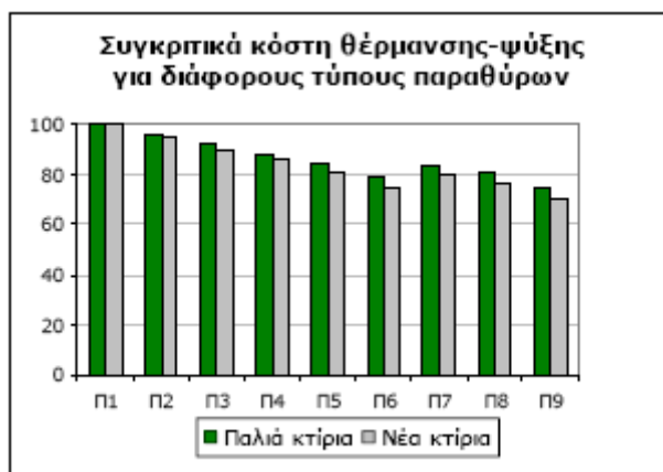
Εικόνα 18: Συγκριτικά κόστη θέρμανσης-ψύξης για διάφορους τύπους παραθύρων [25].
