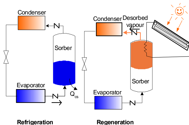
Εικόνα 103: . Διαδικασία ηλιακού κλιματισμού με προσρόφηση [106].
