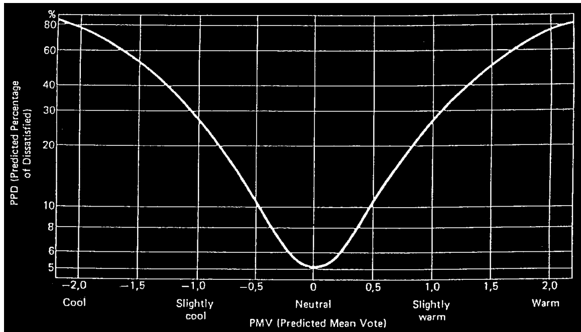
Διάγραμμα 3: Δείκτες PMV, PPD [18]
