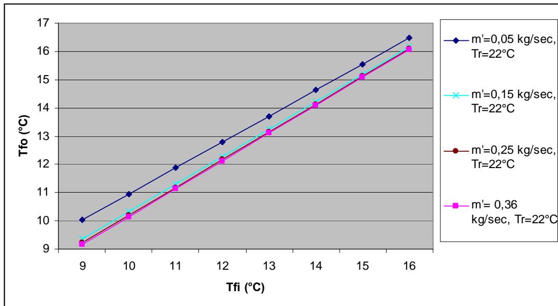
Διάγραμμα 36: Η θερμοκρασία εξόδου T_{f,o} του ρευστού από το σωλήνα, σε συνάρτηση με την θερμοκρασία εισόδου του T_{f,i} , για διαφορετικές παροχές μάζας m' και θερμοκρασία T_r=22^\circ\text{C} του εσωτερικού αέρα, για c_p=4184\text{ J/kg }^\circ\text{C} , n=4 αγωγοί, μήκους L=3\text{m} , απόσταση S=0,2\text{m} , h=10\text{ W m}^{-2}\text{ }^\circ\text{C}^{-1} , k=1,4\text{ W m}^{-1}\text{ }^\circ\text{C}^{-1} , διαμέτρους D_o=0,02\text{ m} , D_i=0,018\text{ m} , w=0,04\text{m} και F_1=0,718321 (από Πίνακα 43).
