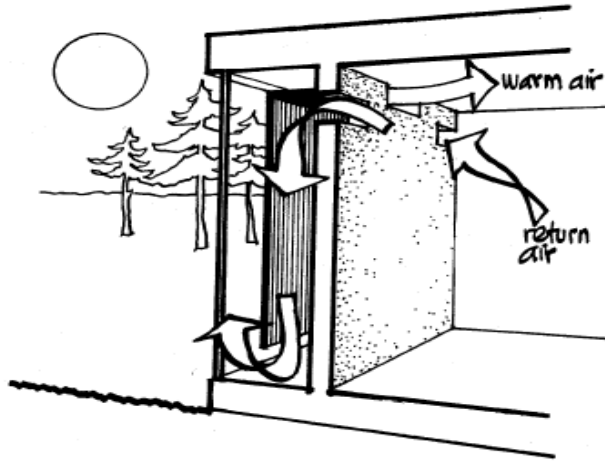
Εικόνα 23: Τοίχος Trombe [23].
