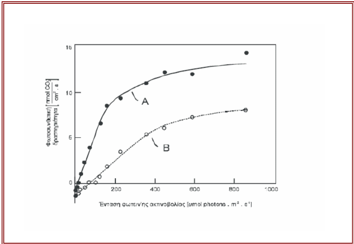
Εικόνα 3.7: φωτοαναστολή της φωτοσύνθεσης. Ρυθμός φωτοσύνθεσης φύλλων πριν (καμπύλη A) και μετά (καμπύλη B) την έκθεση σε συνθήκες καταπόνησης υπερβολικής ακτινοβολίας.
