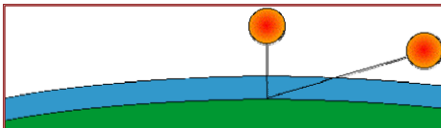
Εικόνα 2.7: σε χαμηλότερο ηλιακό υψόμετρο η ακτίνα διανύει μεγαλύτερη απόσταση στην ατμόσφαιρα
