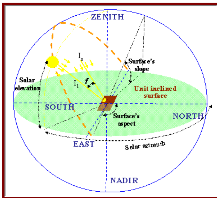
Εικόνα 2.13: παράγοντες που υπεισέρχονται στον υπολογισμό της εισερχόμενης δυναμικής ακτινοβολίας.
