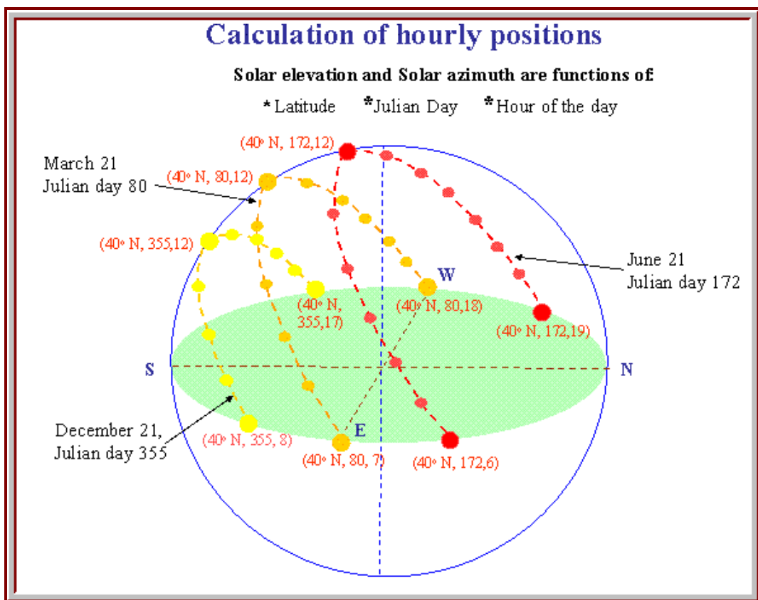
Εικόνα 2.10: παράγοντες που υπεισέρχονται στον υπολογισμό της εισερχόμενης ακτινοβολίας ανά ώρα
