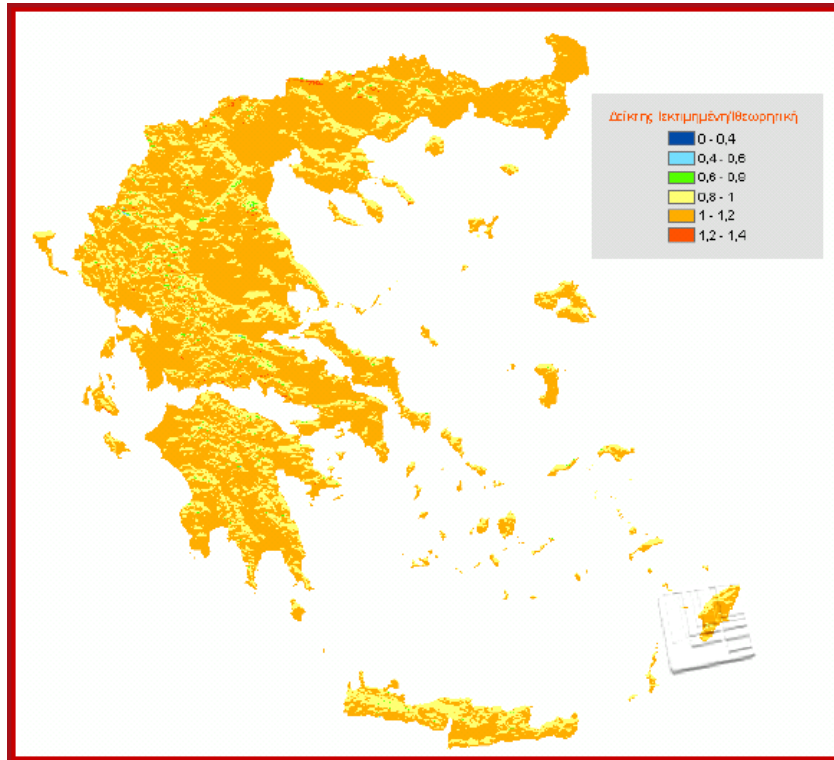
Εικόνα 4.3: δείκτης I_{\text{εκτιμημένη}} / I_{\text{θεωρητική}} ακτινοβολία στον Ελλαδικό χώρο.
