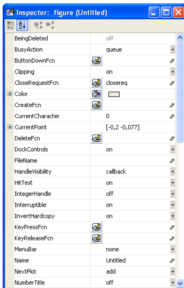
Σχήμα 5.4: Property inspector
