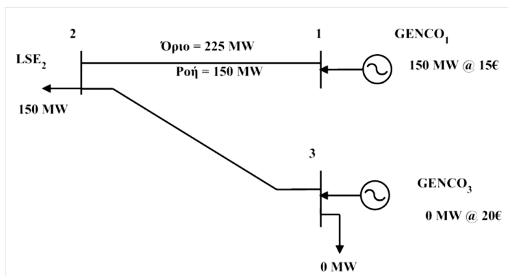
Σχήμα Π1. Σύστημα Χωρίς Συμφόρηση.
