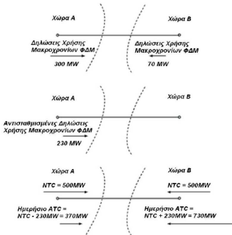
Σχήμα 6. Διαδικασία Κατά τον Υπολογισμό της Διαθέσιμης Ισχύος για Βραχυχρόνια Εκχώρηση Δικαιωμάτων Μεταφοράς από τις Δύο Πλευρές της Διασύνδεσης.
