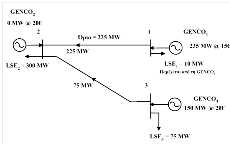
Σχήμα Π3. Απεικόνιση Συστήματος Όπου το FTR Αποφέρει Ζημία.
