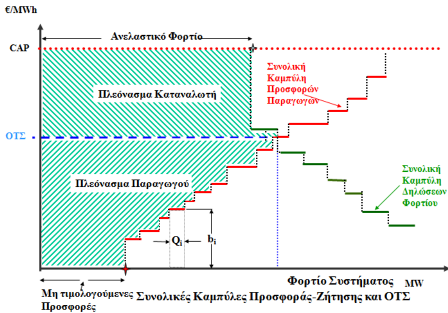
Σχήμα 2. Προσδιορισμός OTS στον ΗΕΠ από τις Καμπύλες Προσφοράς και Ζήτησης.
