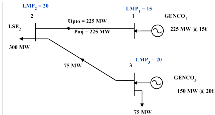
Σχήμα Π2. Σύστημα με Συμφόρηση.
