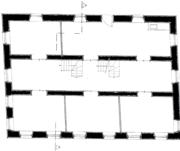
Κάτοψη και τομή τυπολογίας Β, της οικίας Δανιλούλη
