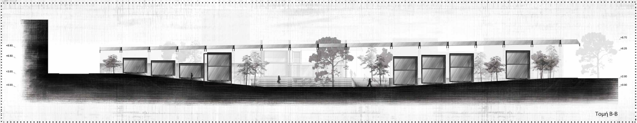
Τομή Α-Α
