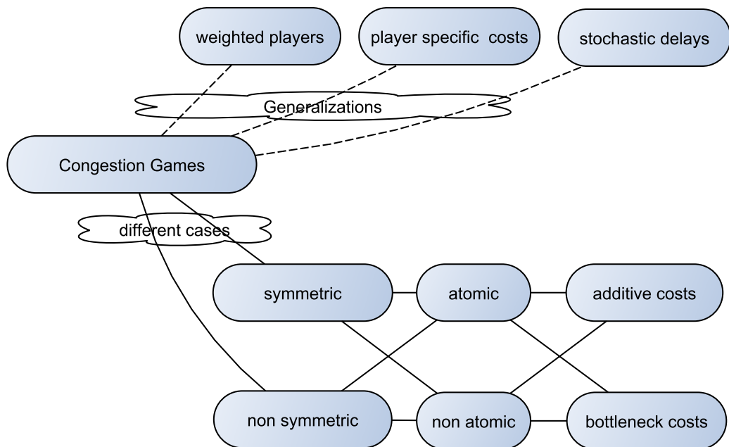
Σχήμα 1.1: Χάρτης (μικρός) δικτυακών παιγνίων συμφόρησης. Αναπαρίστανται στο πάνω μέρος οι επικρατούσες γενικεύσεις των ΠΣ. Το κάτω μέρος αναπαριστά τις διαφορετικές περιπτώσεις που προκύπτουν εξετάζοντας τις παραδοχές σχετικά με το χώρο στρατηγικών των παικτών, τους τύπους των παικτών και του κόστους των στρατηγικών των παικτών.
