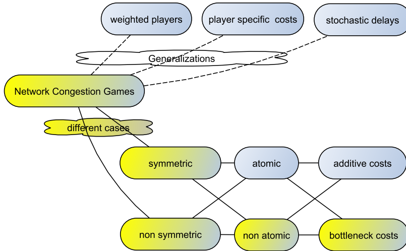
Σχήμα 2.1: Το κεντρικό αποτέλεσμα που ισχύει τόσο σε συμμετρικά όσο και σε μη συμμετρικά παίγνια με ακμές συγκέντρωσης.
