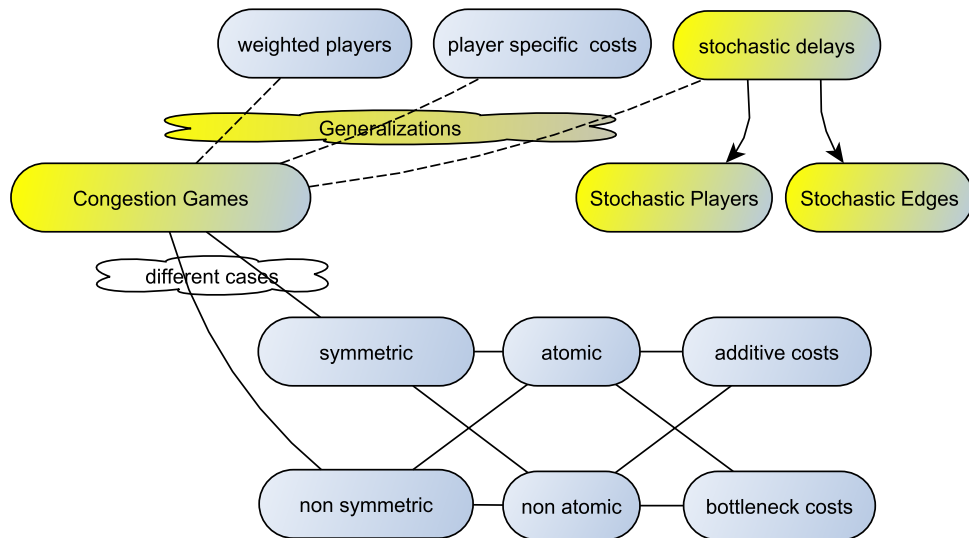
Σχήμα 2.3: Τα εισηγμένα μοντέλα και η τοποθέτησή τους στο Χάρτη.
