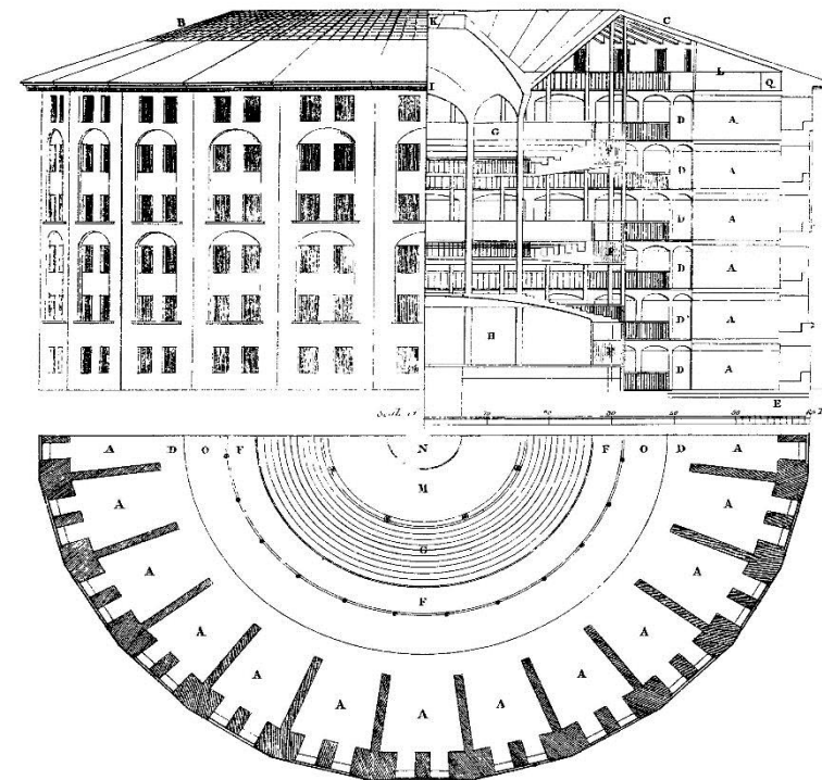
Σχέδιο του Πανοπτικών, πηγή: Τα έργα του Jeremy Bentham, vol. IV, 172-3, 1843 (αρχικά το 1791), http://tr.wikipedia.org/wiki/Dosya:Panopticon.jpg
