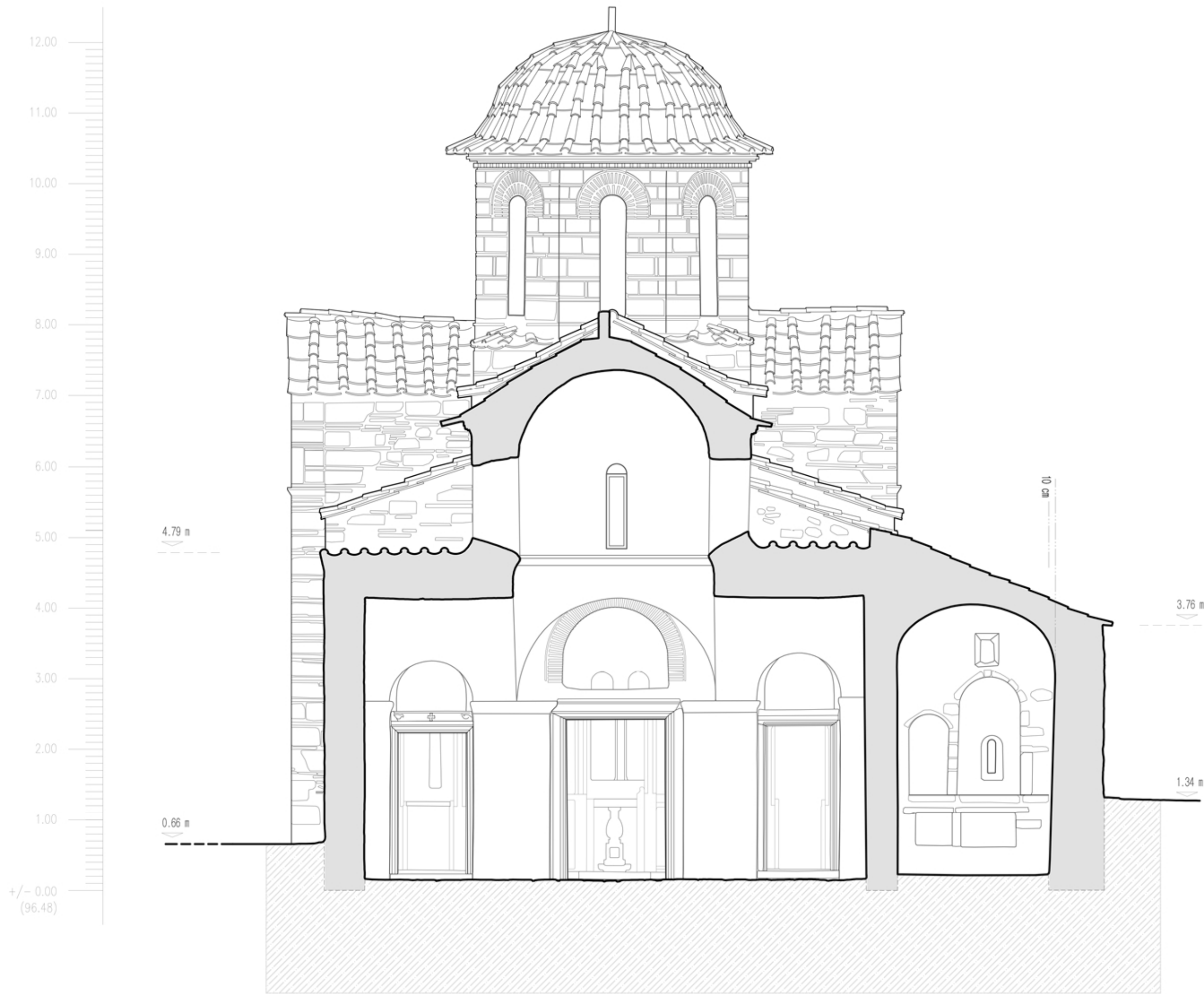
ΚΑΤΑ ΠΛΑΤΟΣ ΤΟΜΗ
