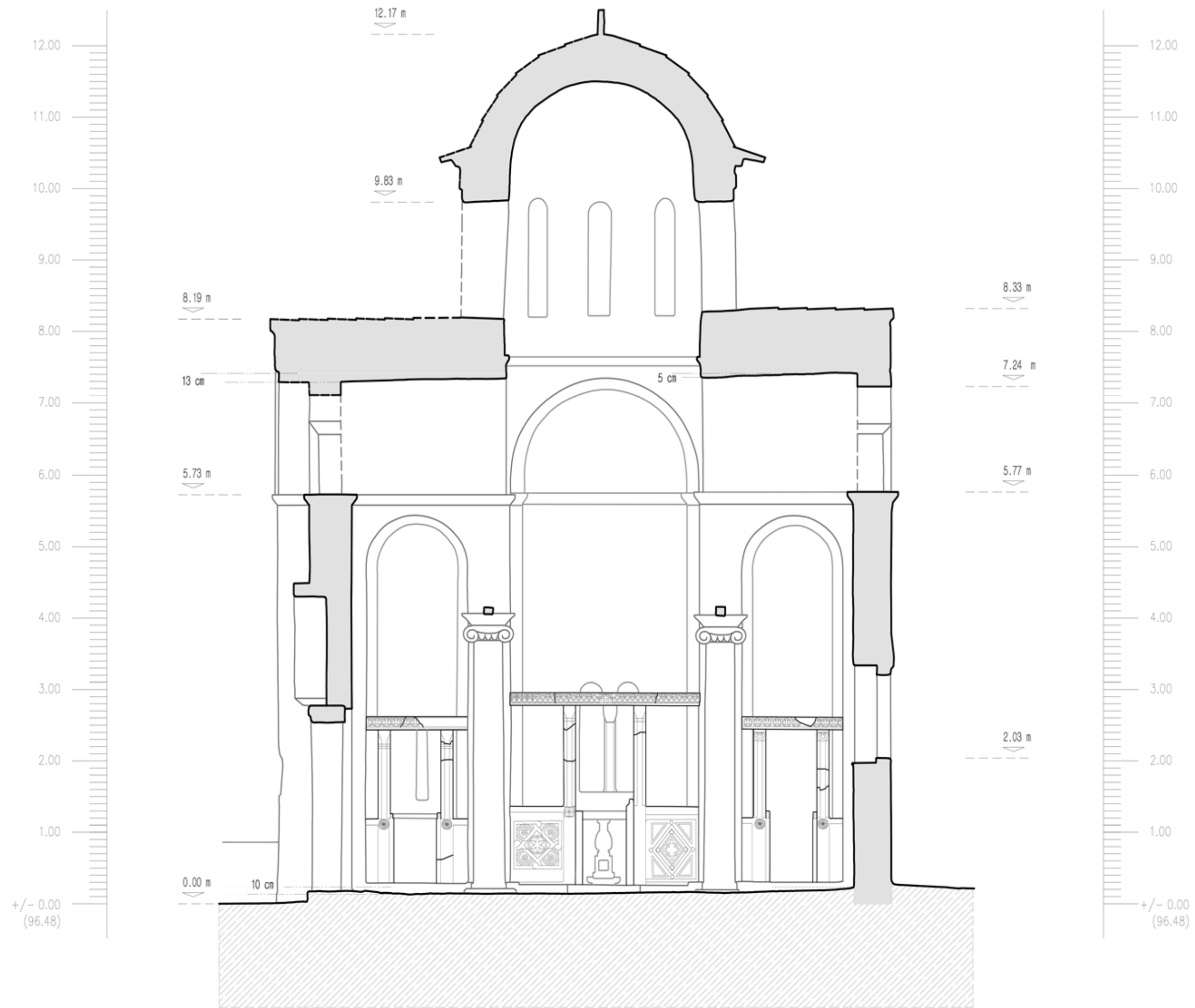
ΚΑΤΑ ΠΛΑΤΟΣ ΤΟΜΗ Β--Β'
