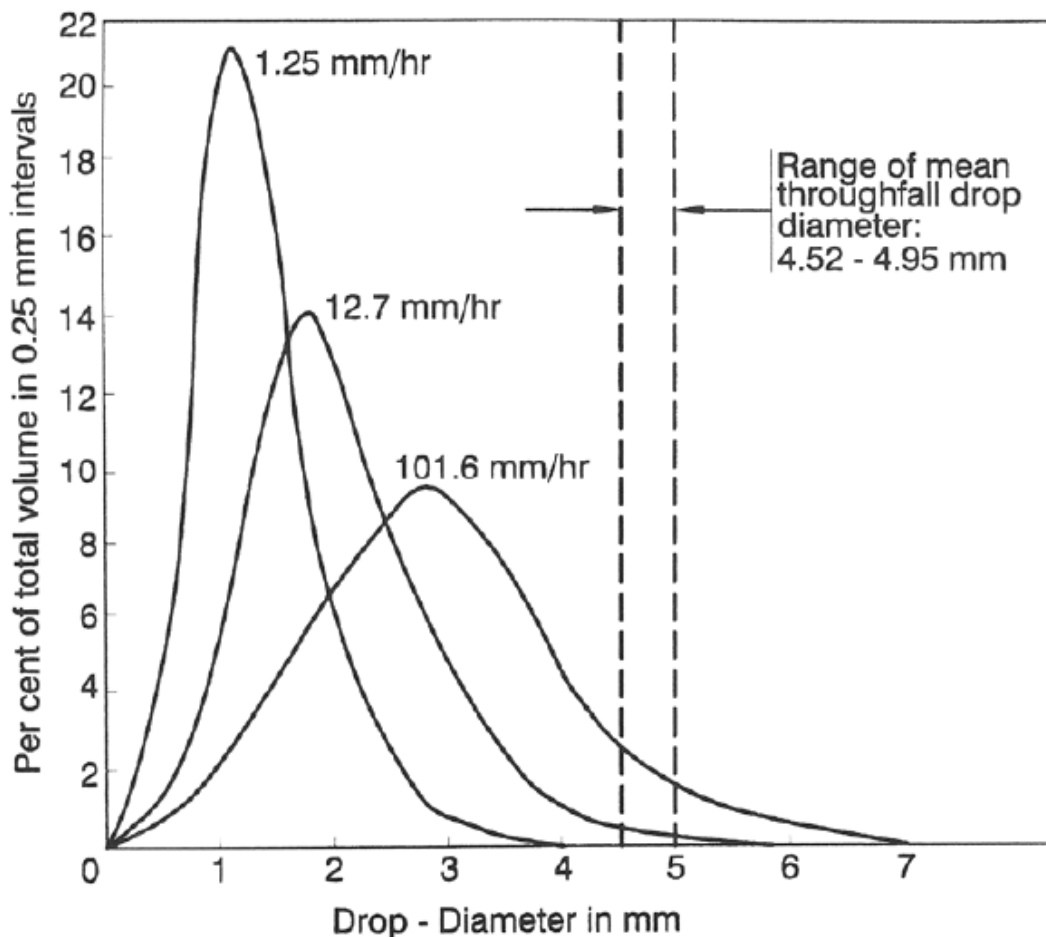
Σχήμα 2.1 Ποσοστό του συνολικού όγκου των σταγόνων σε συνάρτηση της διαμέτρου τους για τρεις διαφορετικές τιμές σφοδρότητας βροχοπτώσης (Lars and Parsons, 1943). Σύγκριση με το εύρος του μέσου μεγέθους της σταγόνας (Brandt, 1990).
