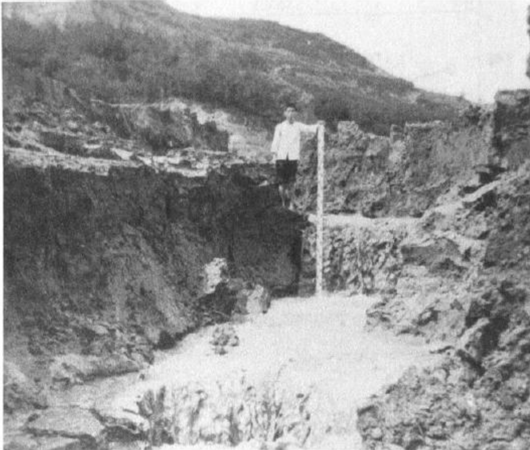
Εικόνα 3.14 Σημείο απότομης αλλαγής κλίσης παλινδρομικής διάβρωσης, ταμιευτήρας Heisonglin, της Κίνας (Morris and Fan, 1998).
