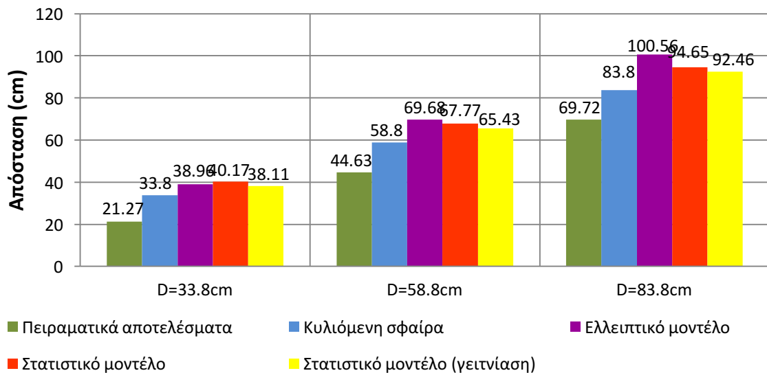
Σχήμα 4.54: Συγκριτικό διάγραμμα των αποστάσεων πρόσκρουσης ανά απόσταση φορτισμένης ράβδου-πλάκας, όπου D μετρημένο από το επίπεδο του καταστρώματος. Αρνητική πολικότητα
