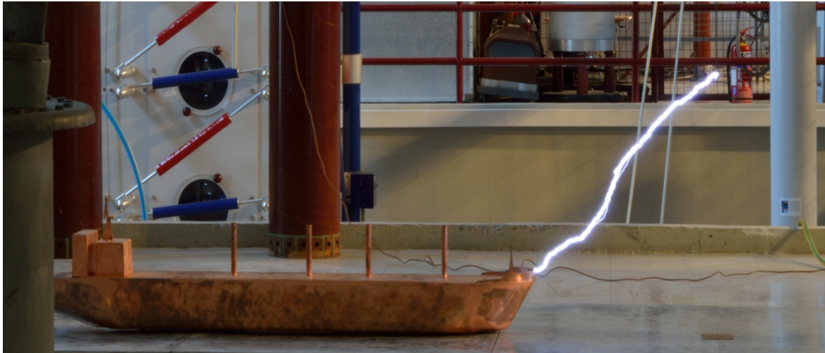
D=75cm Αστοχία
