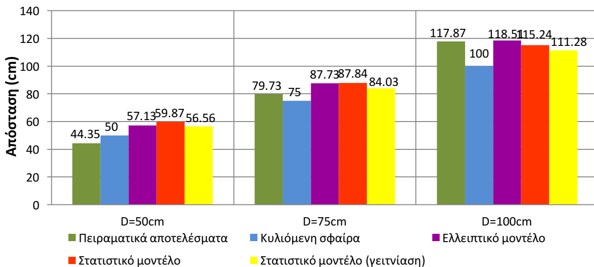
Σχήμα 4.16: Συγκριτικό διάγραμμα των αποστάσεων πρόσκρουσης ανά απόσταση φορτισμένης ράβδου-πλάκας, όπου D μετρημένο από το επίπεδο της γειωμένης πλάκας. Αρνητική πολικότητα
