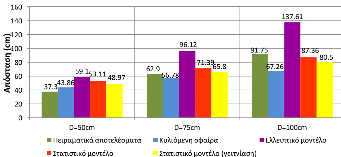
Σχήμα 4.15: Συγκριτικό διάγραμμα των ακτίνων σύλληψης ανά απόσταση φορτισμένης ράβδου-πλάκας, όπου D μετρημένο από το επίπεδο της γειωμένης πλάκας. Αρνητική πολικότητα
