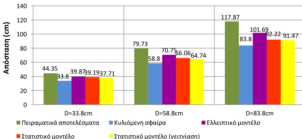
Σχήμα 4.18: Συγκριτικό διάγραμμα των αποστάσεων πρόσκρουσης ανά απόσταση φορτισμένης ράβδου-πλάκας, όπου D μετρημένο από το επίπεδο του καταστρώματος. Αρνητική πολικότητα
