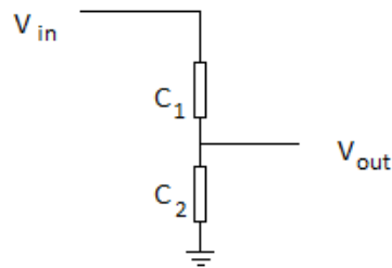
Σχήμα 4.4:Χωρητικός καταμεριστής
