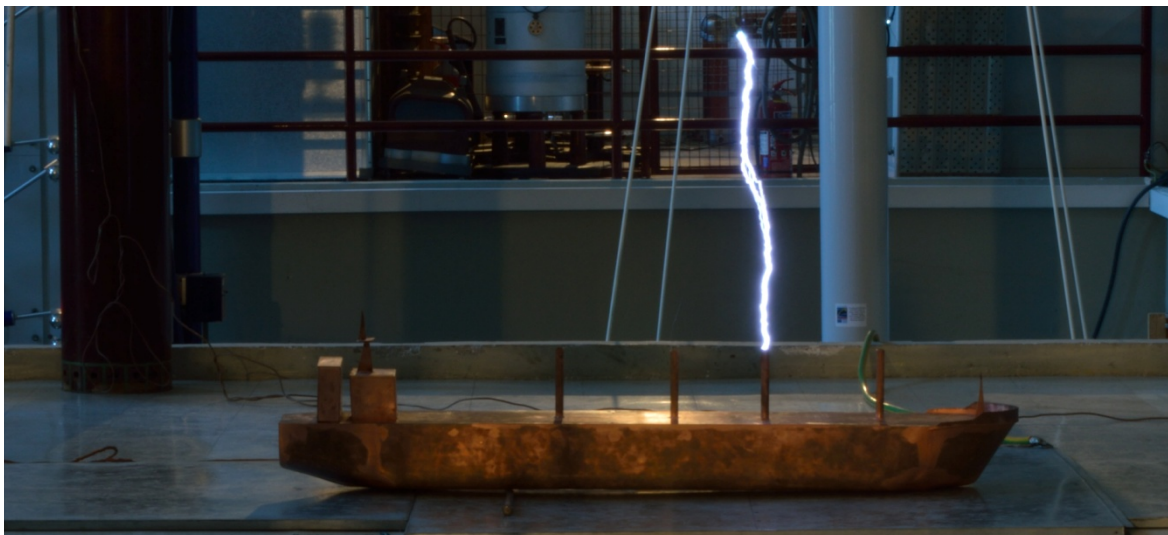
D=100cm Σύλληψη
