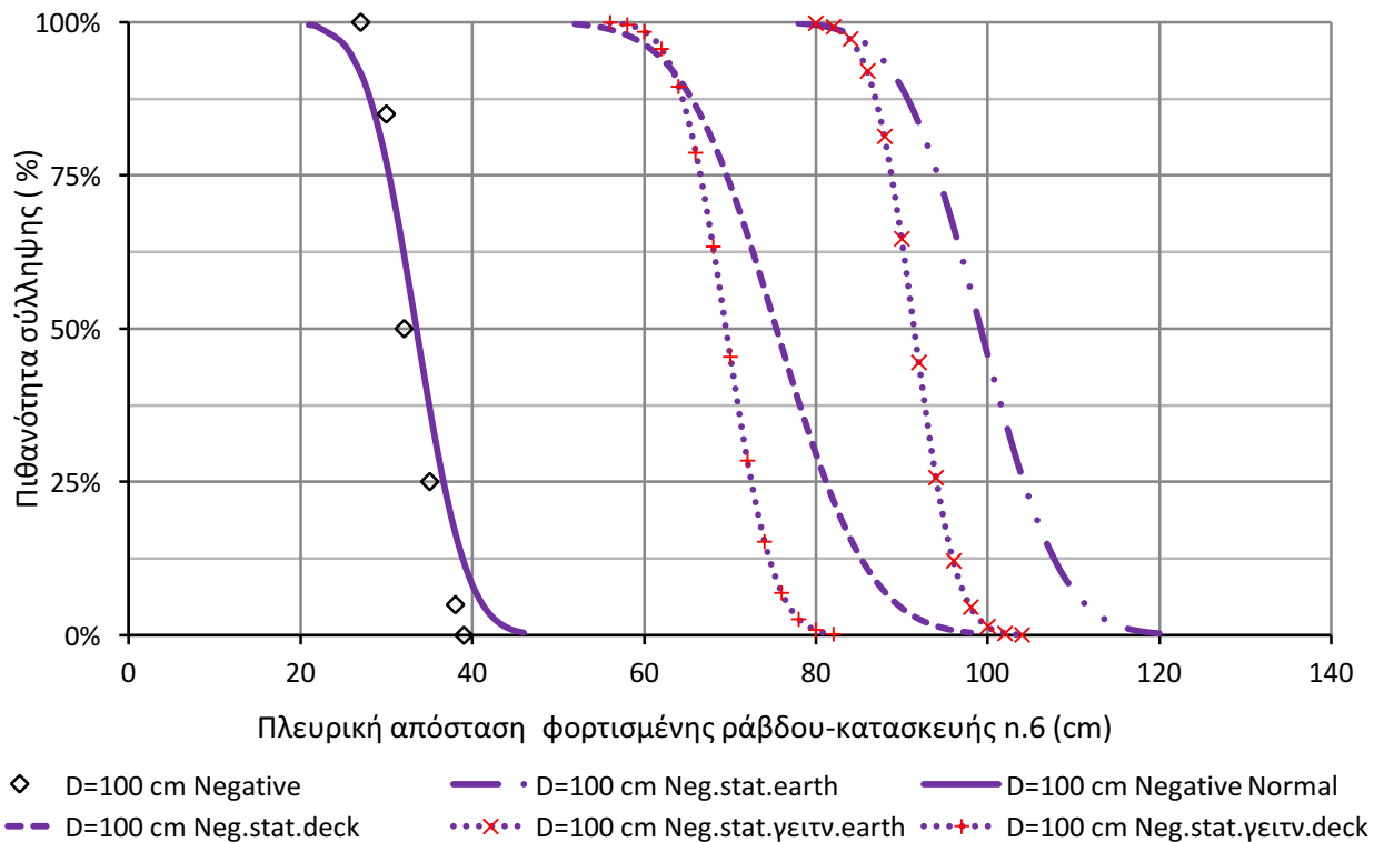
Σχήμα 4.32: Καμπύλες πιθανότητας σύλληψης εκκένωσης από την κατασκευή n.6 του πλοίου, όταν αυτή προσεγγίζεται από την κατασκευή n.5, για απόσταση φορτισμένης ράβδου-πλάκας D=100cm όπως αυτές προκύπτουν από τα πειραματικά δεδομένα και το στατιστικό μοντέλο.
