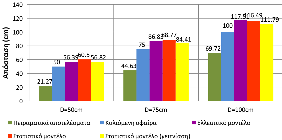
Σχήμα 4.52: Συγκριτικό διάγραμμα των αποστάσεων πρόσκρουσης ανά απόσταση φορτισμένης ράβδου-πλάκας, όπου D μετρημένο από το επίπεδο της γειωμένης πλάκας. Αρνητική πολικότητα.
