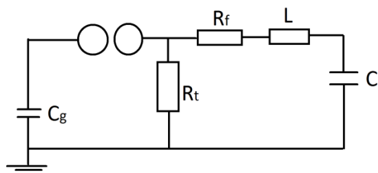
Σχήμα 4.2: Ισοδύναμο κύκλωμα μιας βαθμίδας της κρουστικής γεννήτριας, όπου διακρίνονται τα επιμέρους στοιχεία της [35].
