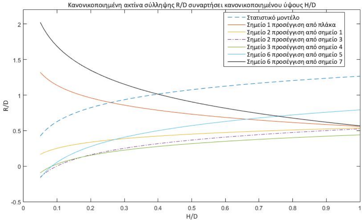
Σχήμα 5.6: Σχήμα 5.5: Κανονικοποιημένη ακτίνα σύλληψης R/D συναρτήσει H/D, όπως αυτή προκύπτει από το στατιστικό μοντέλο και τα πειραματικά δεδομένα, με βάση το εκάστοτε επίπεδο αναφοράς. Αρνητική πολικότητα.
