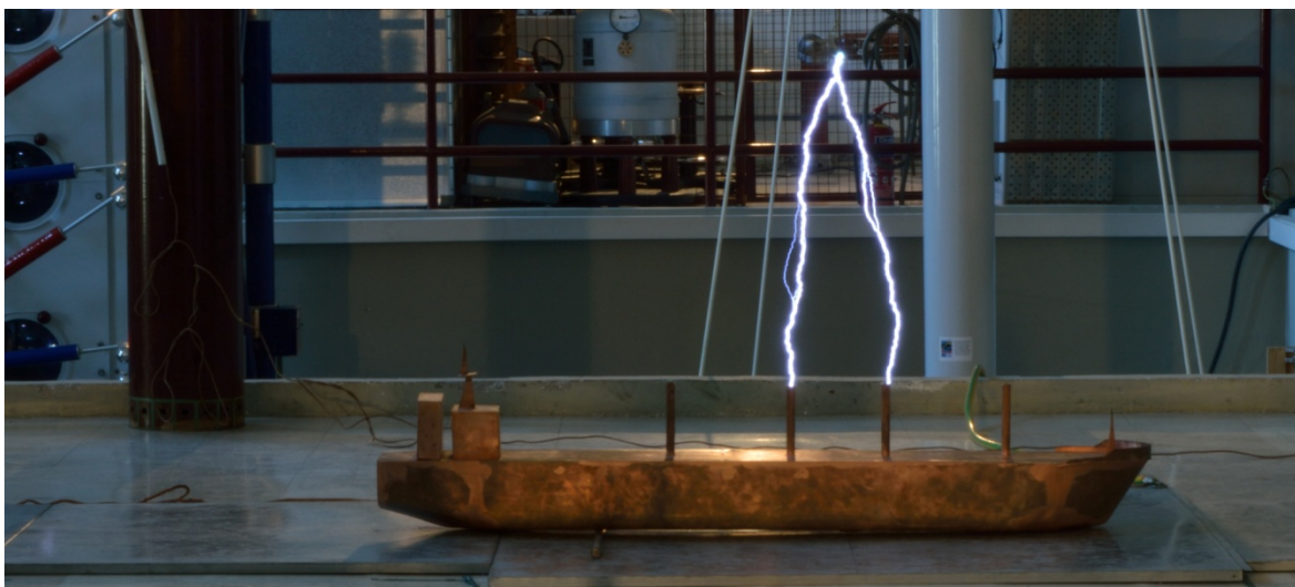
D=100cm Αστοχία
