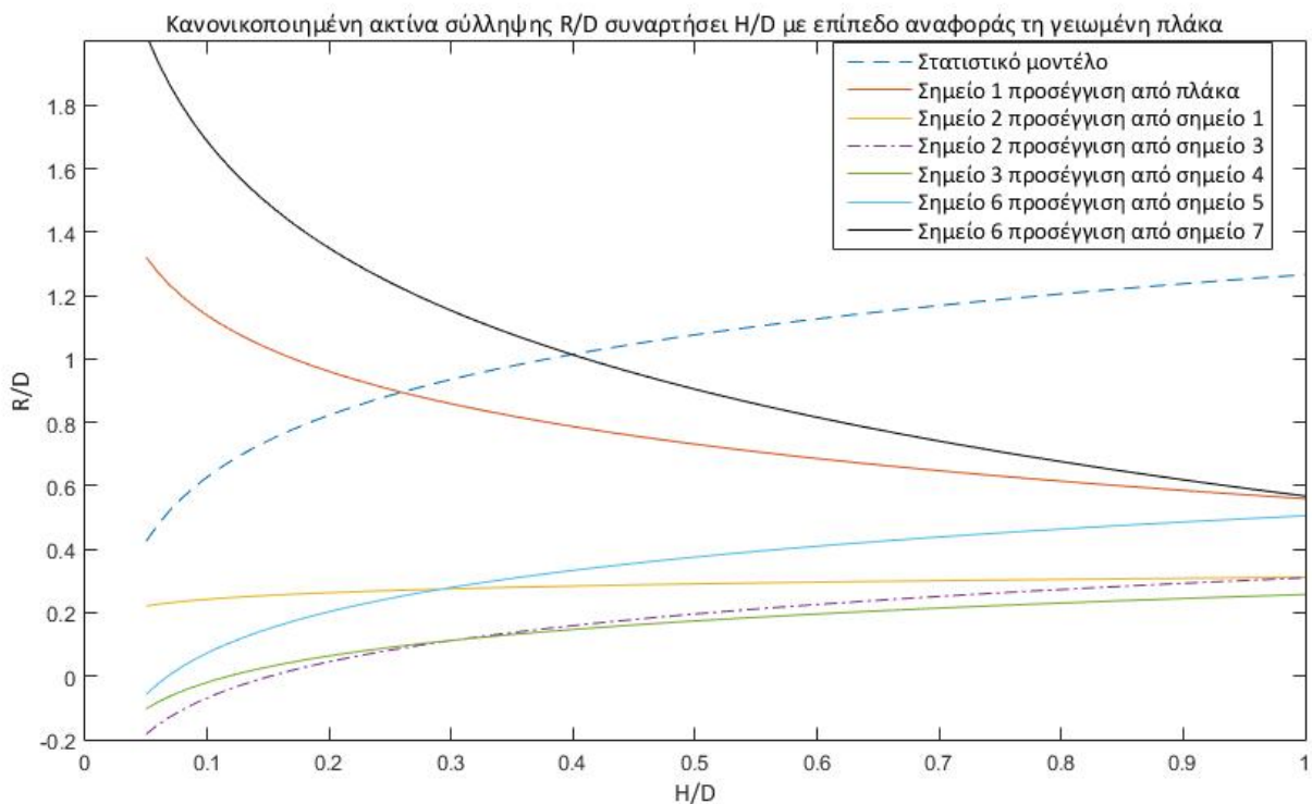
Σχήμα 5.2: Κανονικοποιημένη ακτίνα σύλληψης R/D συναρτήσει H/D , όπως αυτή προκύπτει από το στατιστικό μοντέλο και τα εκάστοτε πειραματικά δεδομένα, με επίπεδο αναφοράς τη γειωμένη πλάκα. Αρνητική πολικότητα.
