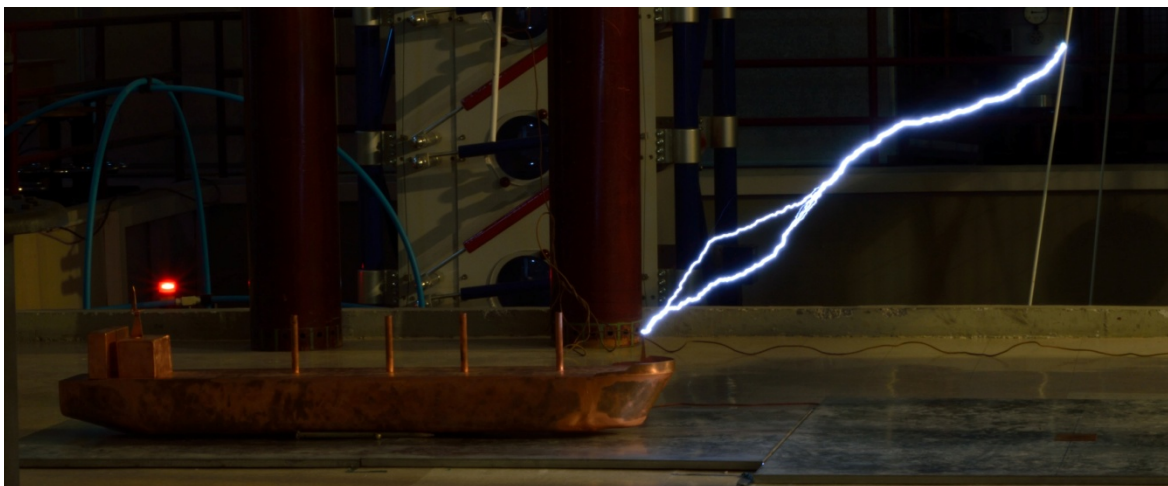
D=100cm Σύλληψη
