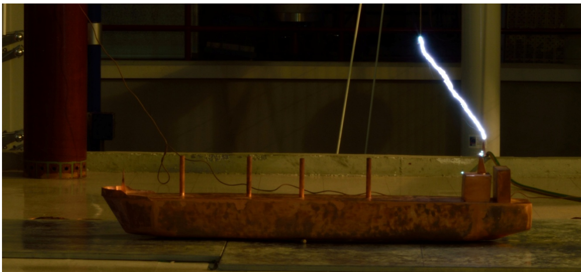
D=75cm Σύλληψη
