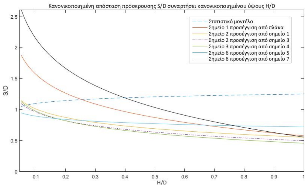
Σχήμα 5.5: Κανονικοποιημένη απόσταση πρόσκρουσης S/D συναρτήσει H/D, όπως αυτή προκύπτει από το στατιστικό μοντέλο και τα πειραματικά δεδομένα, με βάση το εκάστοτε επίπεδο αναφοράς. Αρνητική πολικότητα.
