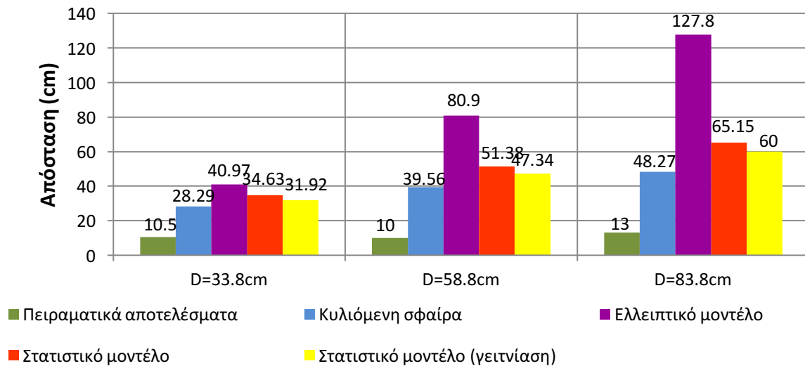
Σχήμα 4.53: Συγκριτικό διάγραμμα των ακτίνων σύλληψης ανά απόσταση φορτισμένης ράβδου-πλάκας, όπου D μετρημένο από το επίπεδο του καταστρώματος. Αρνητική πολικότητα
