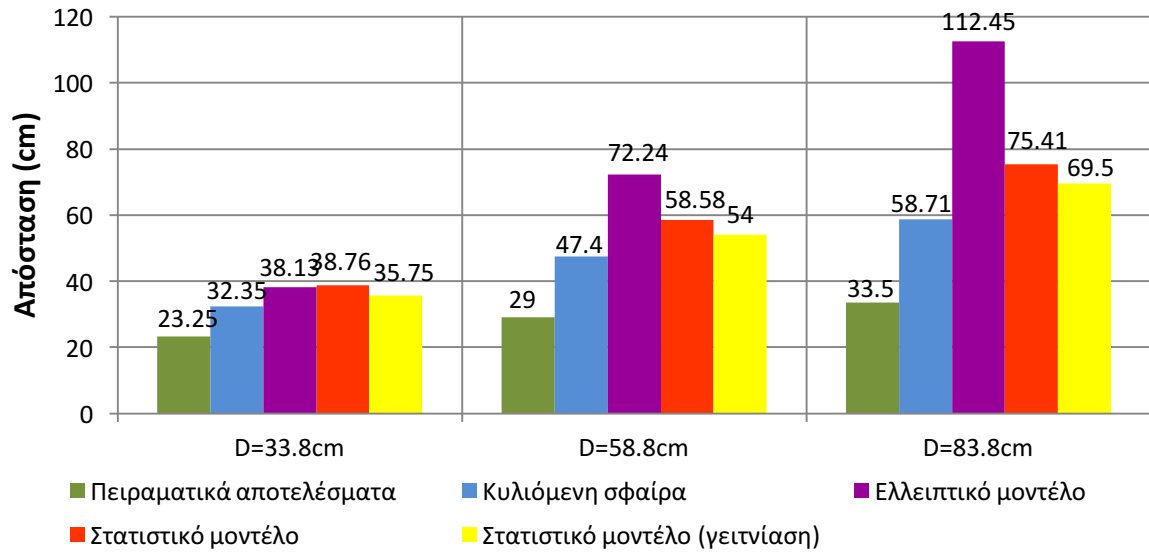
Σχήμα 4.35: Συγκριτικό διάγραμμα των ακτίνων σύλληψης ανά απόσταση φορτισμένης ράβδου-πλάκας, όπου D μετρημένο από το επίπεδο του καταστρώματος. Αρνητική πολικότητα
