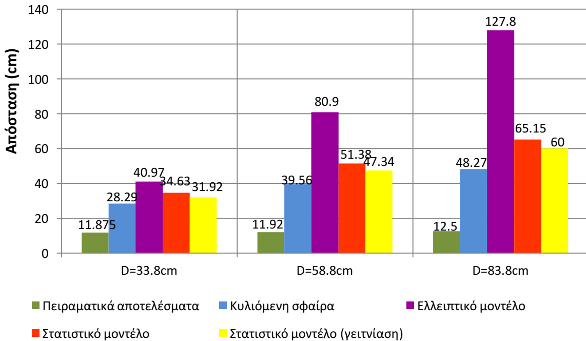
Σχήμα 4.44: Συγκριτικό διάγραμμα των ακτίνων σύλληψης ανά απόσταση φορτισμένης ράβδου-πλάκας, όπου D μετρημένο από το επίπεδο του καταστρώματος. Αρνητική πολικότητα
