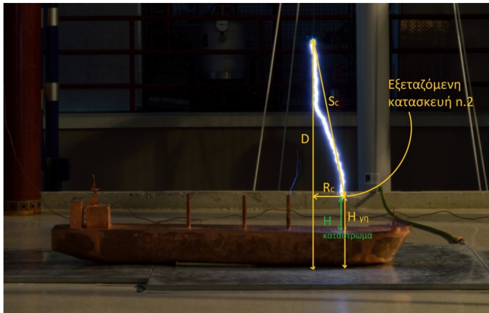
Σχήμα 4.37: Σχηματικό διάγραμμα της προσέγγισης της κατασκευής n.2 από την πλευρά της κατασκευής n.5. R_c : ακτίνα σύλληψης, S_c : απόσταση πρόσκρουσης, D : απόσταση φορτισμένης ράβδου-πλάκας και H : ύψος κατασκευής.
