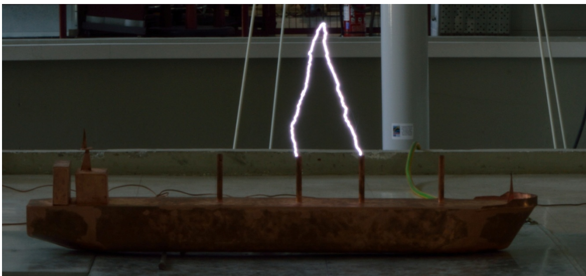
D=75cm Αστοχία
