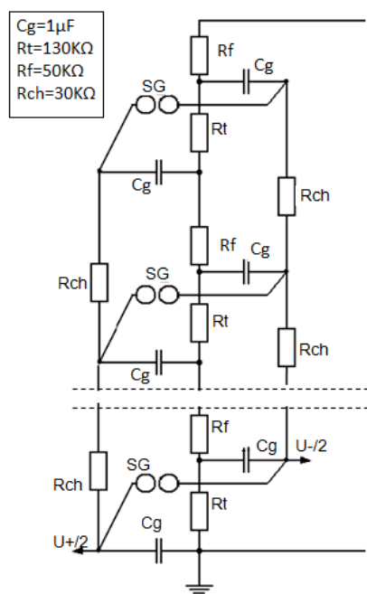
Σχήμα 4.3: Κύκλωμα εννιαβάθμιας κρουστικής γεννήτριας APITZ/CRATOS [35]
