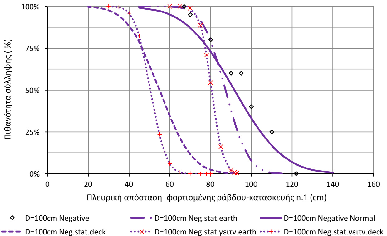
Σχήμα 4.14: Καμπύλες πιθανότητας σύλληψης εκκένωσης από την κατασκευή n.1 του πλοίου για
