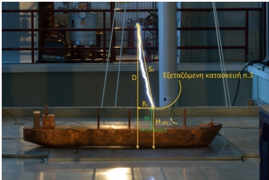
Σχήμα 4.46: Σχηματικό διάγραμμα της προσέγγισης της κατασκευής n.3 από την πλευρά της κατασκευής n.4. R_c : ακτίνα σύλληψης, S_c : απόσταση πρόσκρουσης, D : ύψος φορτισμένης ράβδου και H : ύψος κατασκευής.
