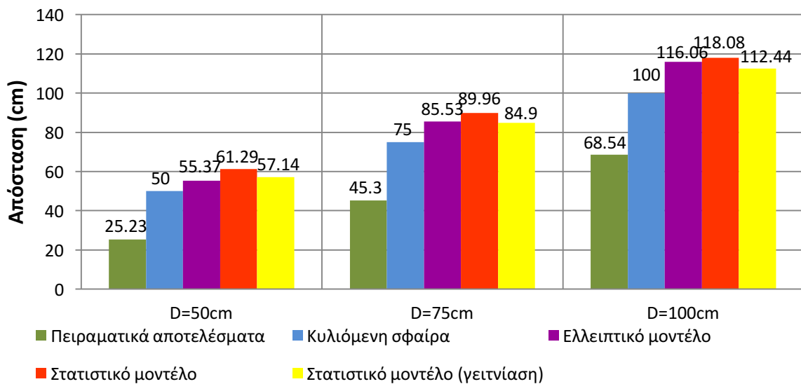
Σχήμα 4.34: Συγκριτικό διάγραμμα των αποστάσεων πρόσκρουσης ανά απόσταση φορτισμένης ράβδου-πλάκας, όπου D μετρημένο από το επίπεδο της γειωμένης πλάκας. Αρνητική πολικότητα.
