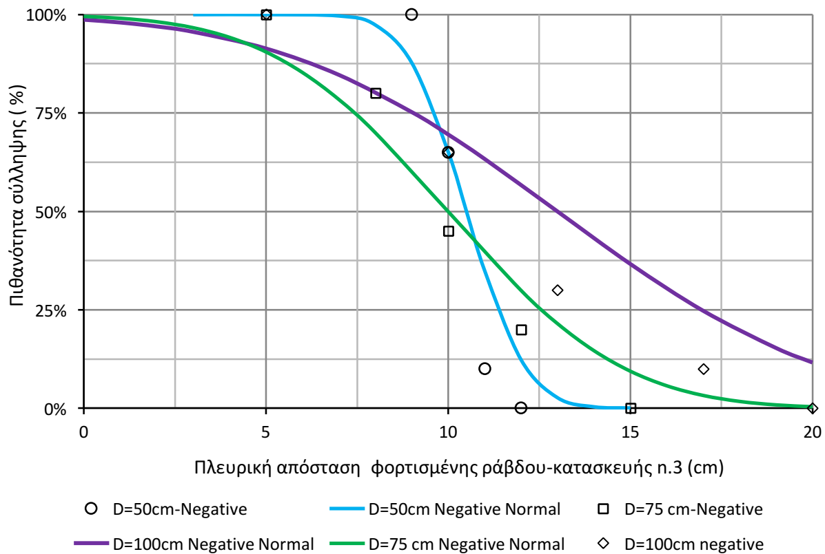
Σχήμα 4.47: Πειραματικές καμπύλες πιθανότητας σύλληψης της εκκένωσης από την κατασκευή n.3 του πλοίου, όταν προσεγγίζεται από την κατασκευή n.4, οι οποίες ακολουθούν κανονική κατανομή.
