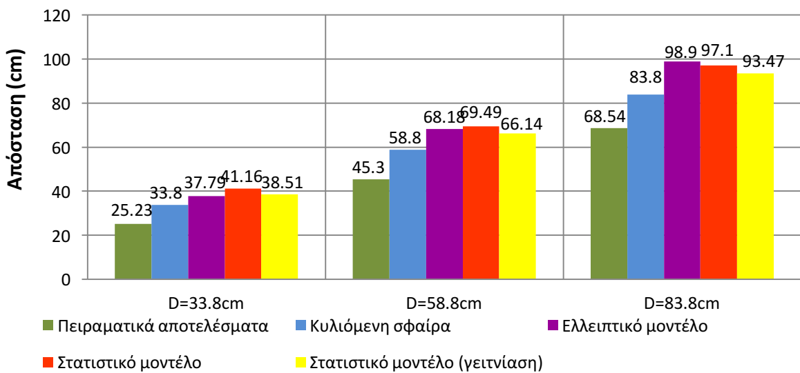
Σχήμα 4.36: Συγκριτικό διάγραμμα των αποστάσεων πρόσκρουσης ανά απόσταση φορτισμένης ράβδου-πλάκας, όπου D μετρημένο από το επίπεδο του καταστρώματος. Αρνητική πολικότητα
