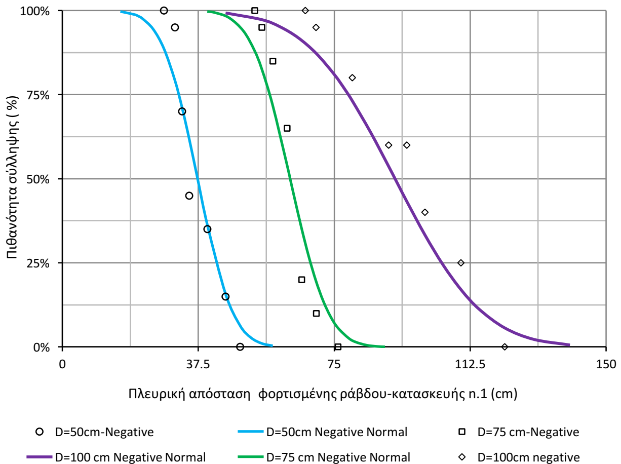
Σχήμα 4.11: Πειραματικές καμπύλες πιθανότητας σύλληψης της εκκένωσης από την κατασκευή n.1 του πλοίου οι οποίες ακολουθούν κανονική κατανομή.
