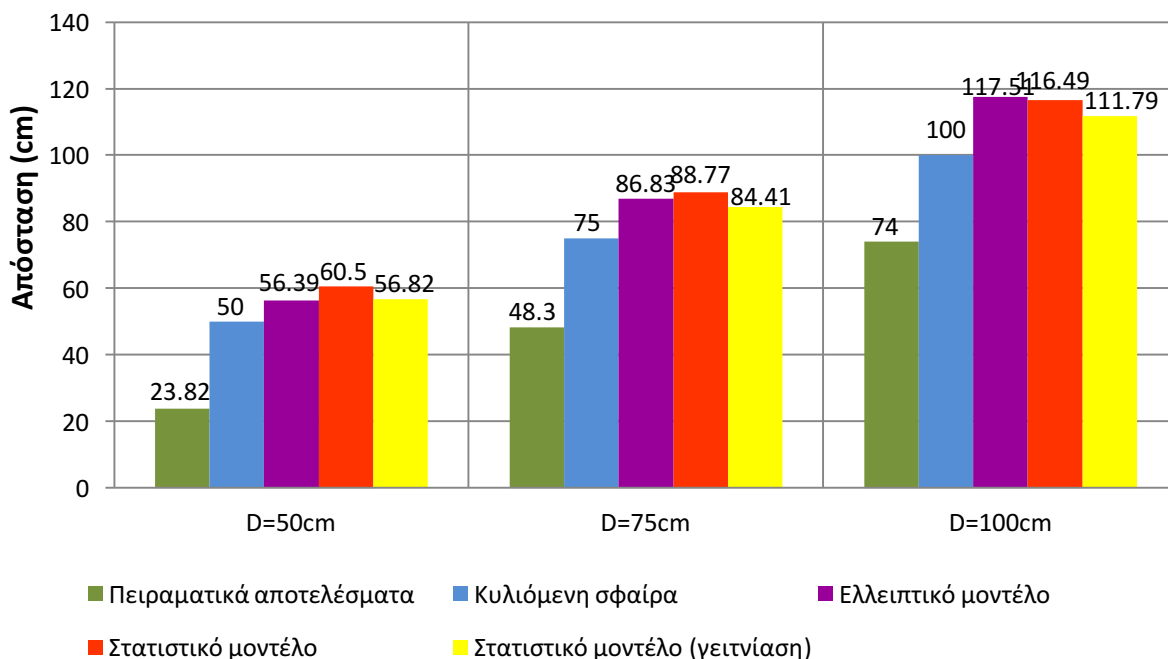
Σχήμα 4.25: Συγκριτικό διάγραμμα των αποστάσεων πρόσκρουσης ανά απόσταση φορτισμένης ράβδου-πλάκας, όπου D μετρημένο από το επίπεδο της γειωμένης πλάκας. Αρνητική πολικότητα
