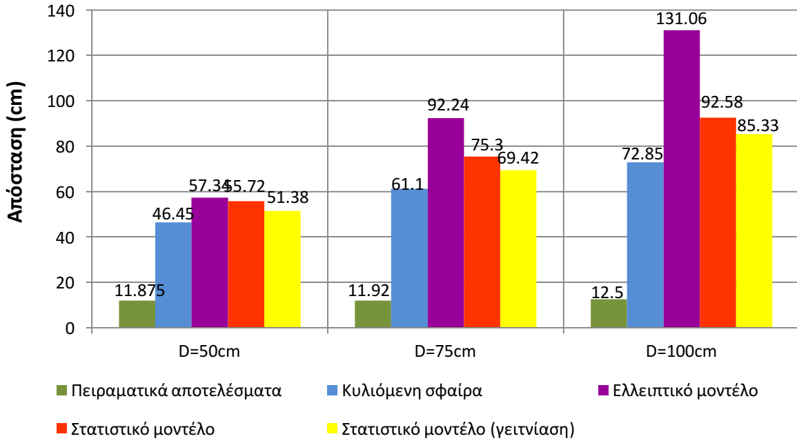
Σχήμα 4.42: Συγκριτικό διάγραμμα των ακτίνων σύλληψης ανά απόσταση φορτισμένης ράβδου-πλάκας, όπου D μετρημένο από το επίπεδο της γειωμένης πλάκας. Αρνητική πολικότητα.
