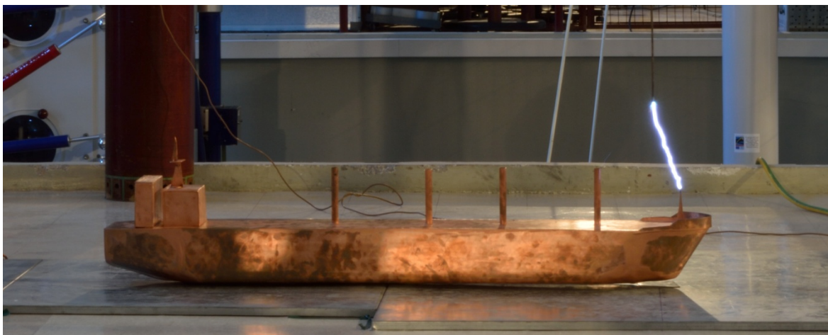
D=50cm Αστοχία
