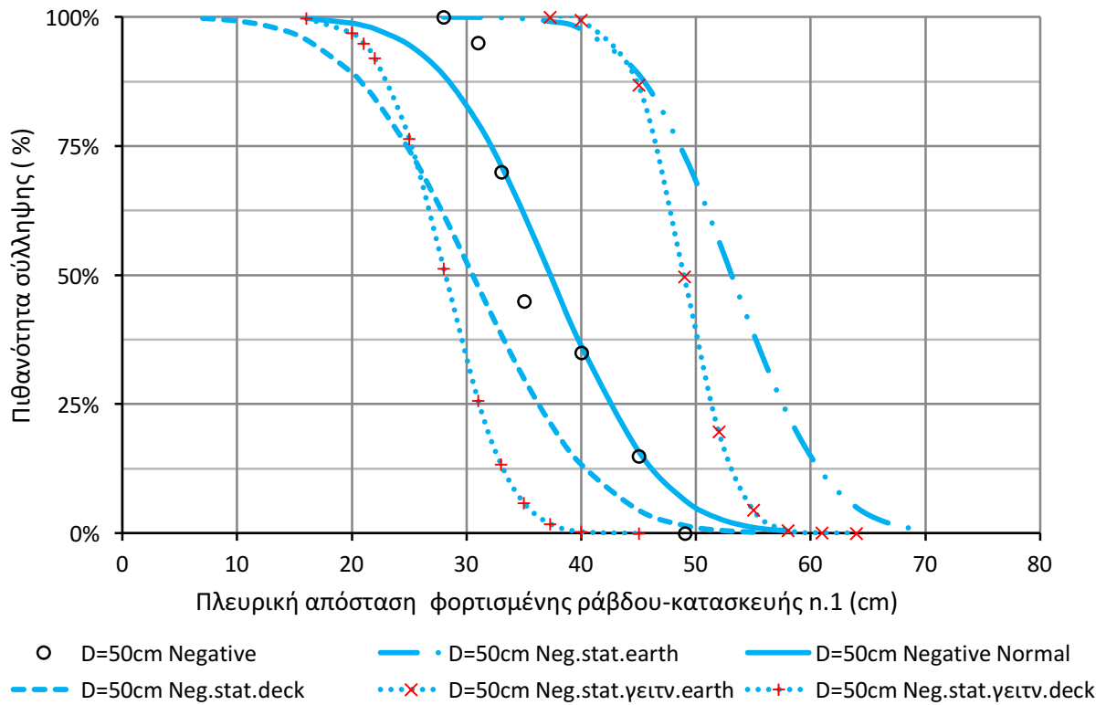
Σχήμα 4.12: Καμπύλες πιθανότητας σύλληψης εκκένωσης από την κατασκευή n.1 του πλοίου για απόσταση φορτισμένης ράβδου-πλάκας D=50cm όπως αυτές προκύπτουν από τα πειραματικά δεδομένα και το στατιστικό μοντέλο.
