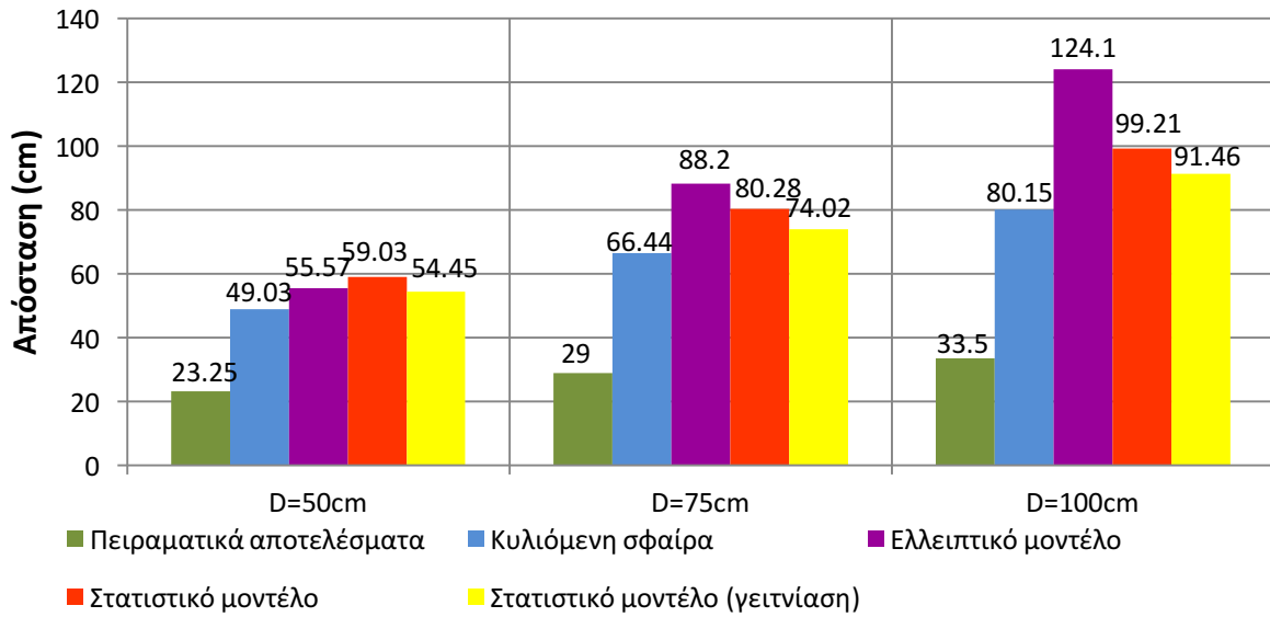
Σχήμα 4.33: Συγκριτικό διάγραμμα των ακτίνων σύλληψης ανά απόσταση φορτισμένης ράβδου-πλάκας, όπου D μετρημένο από το επίπεδο της γειωμένης πλάκας. Αρνητική πολικότητα.
