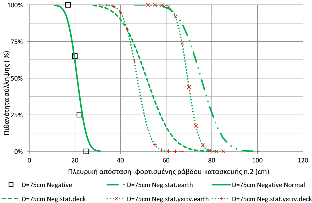
Σχήμα 4.22: Καμπύλες πιθανότητας σύλληψης εκκένωσης από την κατασκευή n.2 του πλοίου, όταν αυτή προσεγγίζεται από την κατασκευή n.1, για απόσταση φορτισμένης ράβδου-πλάκας D=75cm όπως αυτές προκύπτουν από τα πειραματικά δεδομένα και το στατιστικό μοντέλο.
