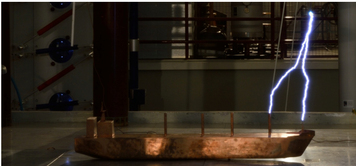
D=100cm Αστοχία
