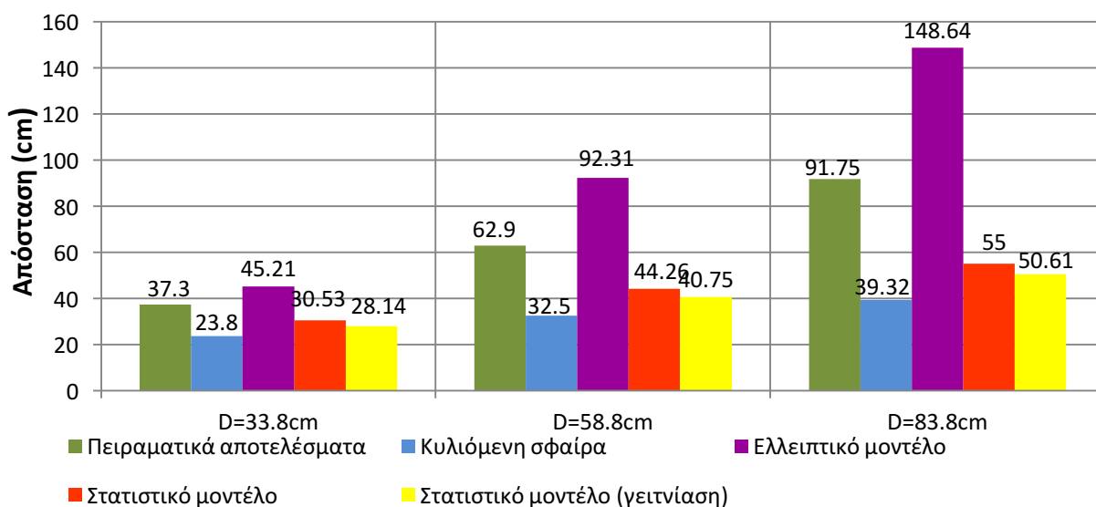
Σχήμα 4.17: Συγκριτικό διάγραμμα των ακτίνων σύλληψης ανά απόσταση φορτισμένης ράβδου-πλάκας, όπου D μετρημένο από το επίπεδο του καταστρώματος. Αρνητική πολικότητα
