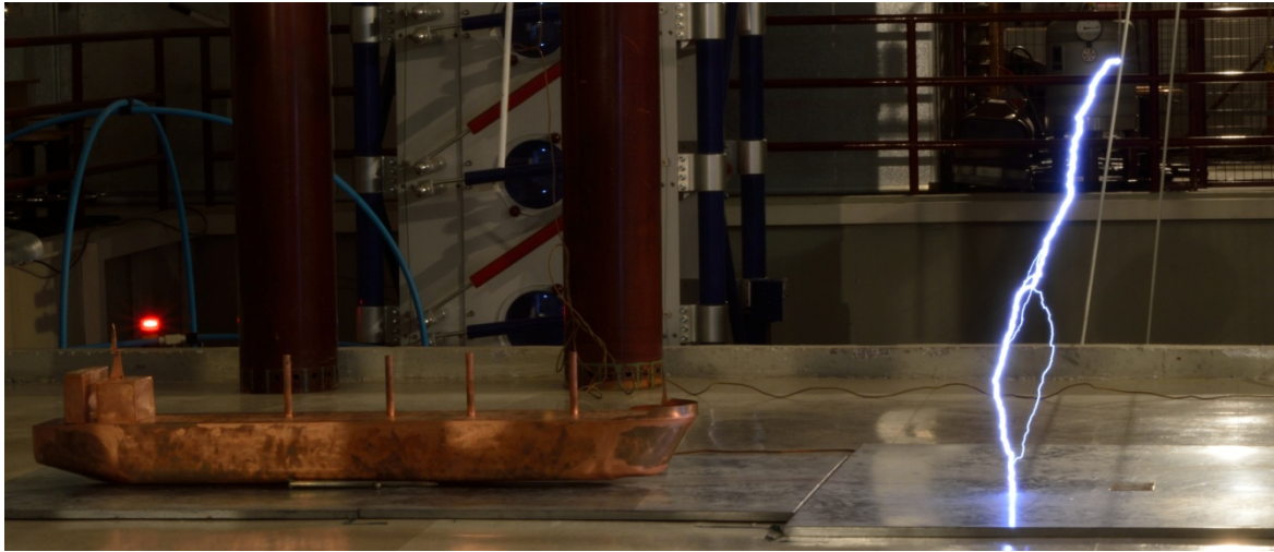
D=100cm Αστοχία
