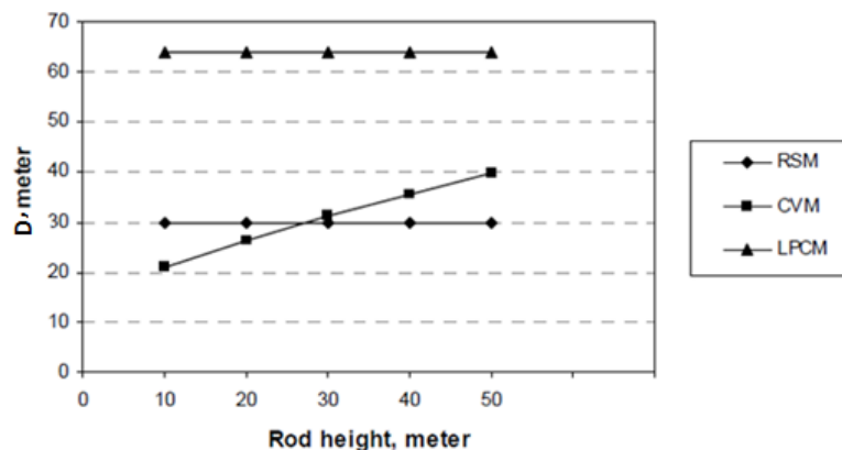
Σχήμα 3.22: Απόσταση πρόσκρουσης για τις μεθόδους RCM, CVM και LPCM συναρτήσεως του ύψους αλεξικέραυνου H για Z = 5000\text{m} και I_p = 5.4 \text{ kA} [29]
