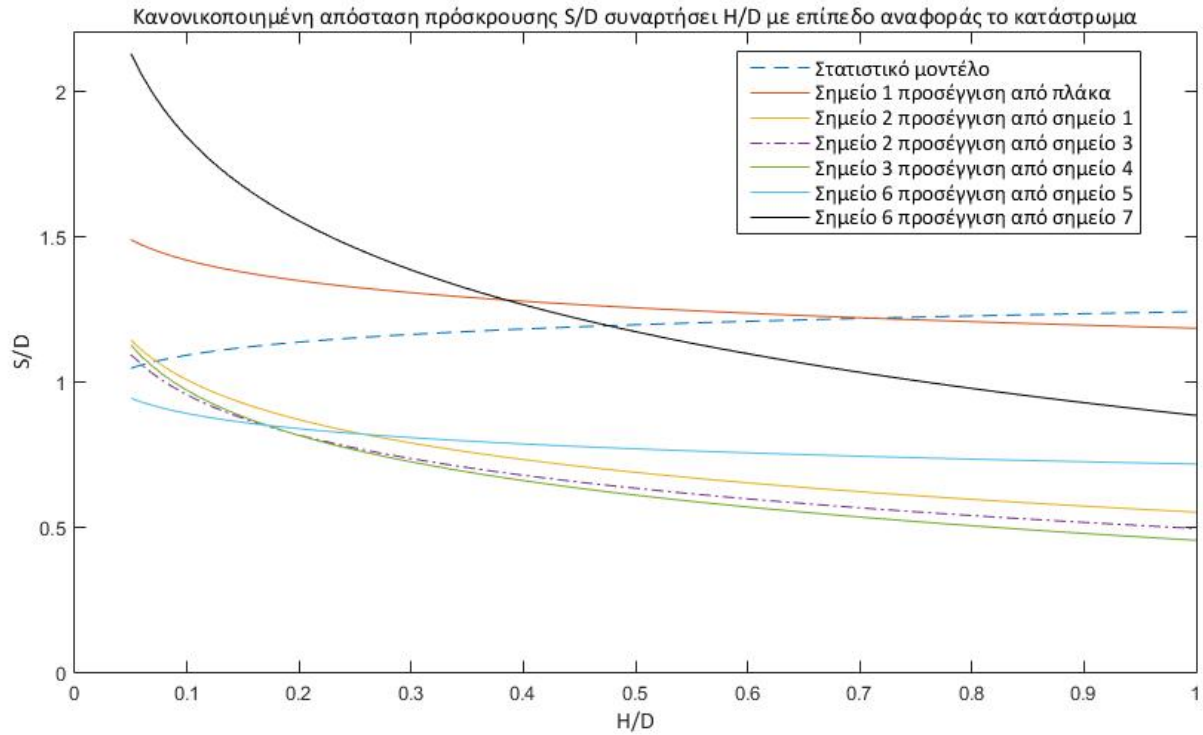
Σχήμα 5.3: Κανονικοποιημένη απόσταση πρόσκρουσης S/D συναρτήσει H/D , όπως αυτή προκύπτει από το στατιστικό μοντέλο και τα εκάστοτε πειραματικά δεδομένα, με επίπεδο αναφοράς το κατάστρωμα. Αρνητική πολικότητα.
