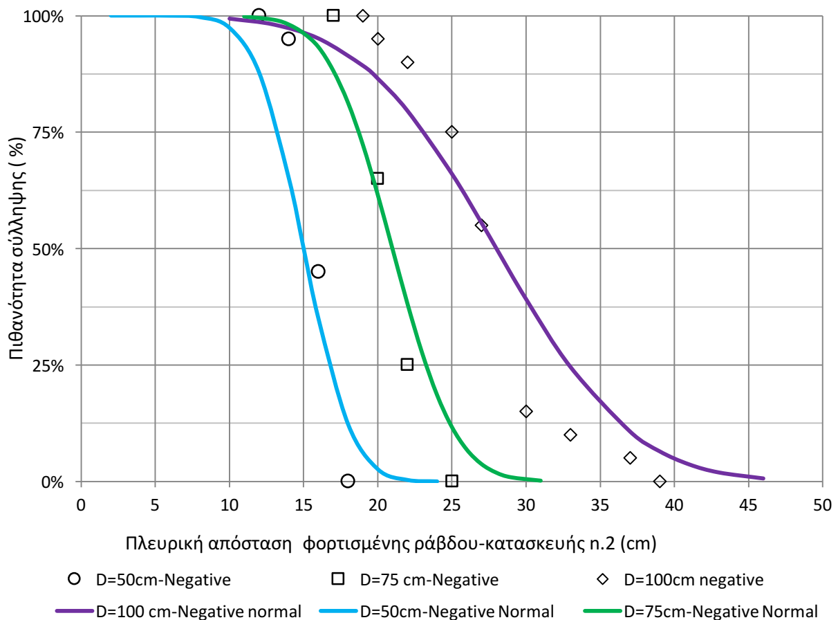
Σχήμα 4.20: Πειραματικές καμπύλες πιθανότητας σύλληψης της εκκένωσης από την κατασκευή n.2 του πλοίου, όταν προσεγγίζεται από την κατασκευή n.1, οι οποίες ακολουθούν κανονική κατανομή.
