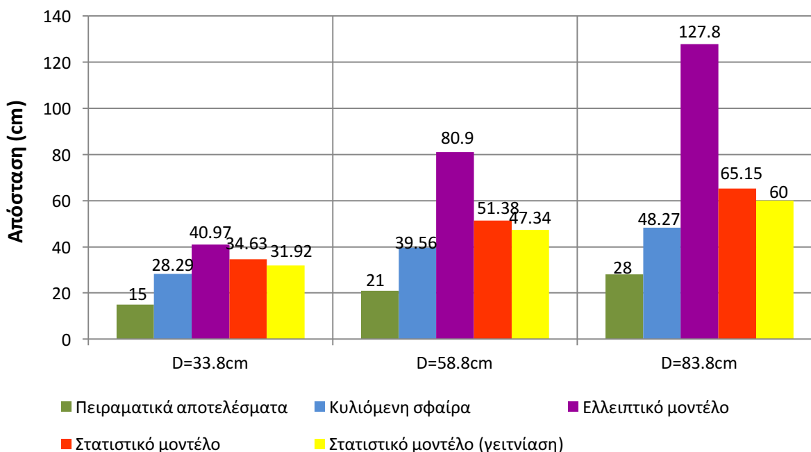
Σχήμα 4.26: Συγκριτικό διάγραμμα των ακτίνων σύλληψης ανά απόσταση φορτισμένης ράβδου-πλάκας, όπου D μετρημένο από το επίπεδο του καταστρώματος. Αρνητική πολικότητα
