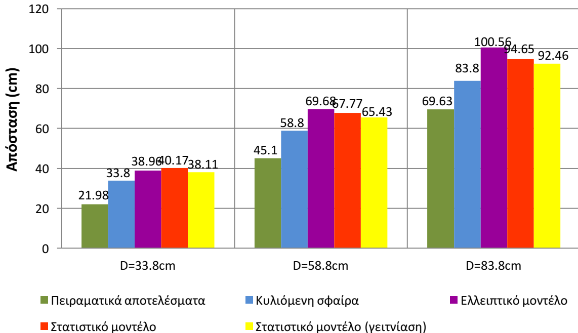
Σχήμα 4.45: Συγκριτικό διάγραμμα των αποστάσεων πρόσκρουσης ανά απόσταση φορτισμένης ράβδου-πλάκας, όπου D μετρημένο από το επίπεδο του καταστρώματος. Αρνητική πολικότητα
