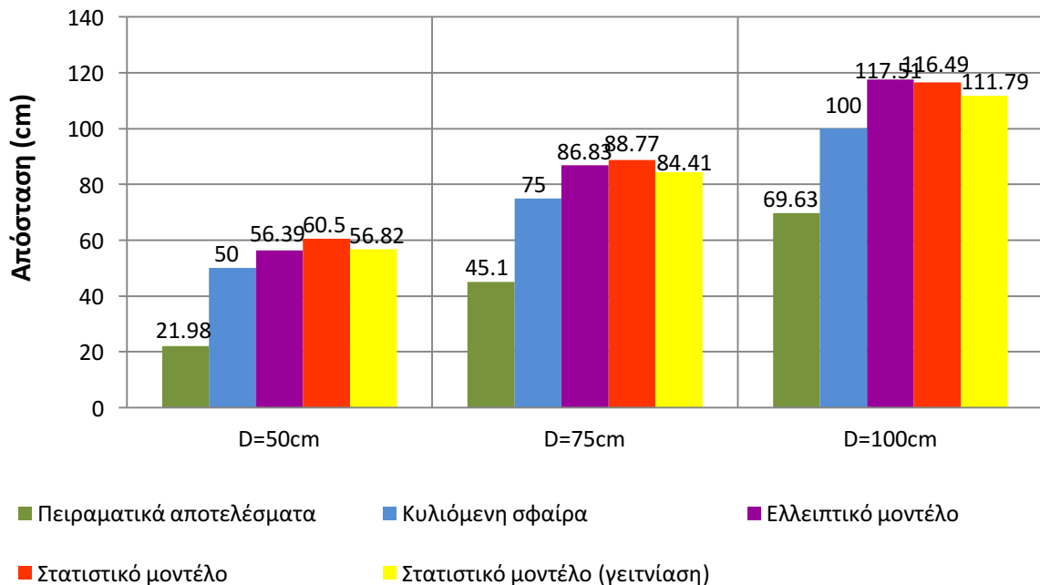
Σχήμα 4.43: Συγκριτικό διάγραμμα των αποστάσεων πρόσκρουσης ανά απόσταση φορτισμένης ράβδου-πλάκας, όπου D μετρημένο από το επίπεδο της γειωμένης πλάκας. Αρνητική πολικότητα.
