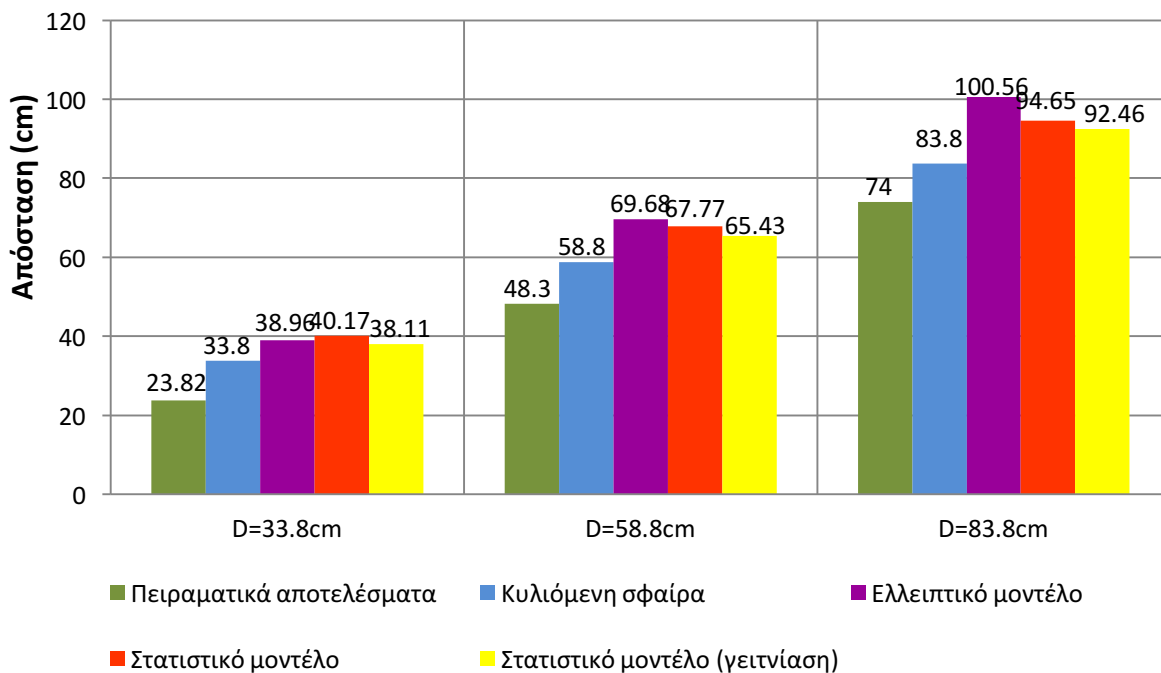
Σχήμα 4.27: Συγκριτικό διάγραμμα των αποστάσεων πρόσκρουσης ανά απόσταση φορτισμένης ράβδου-πλάκας, όπου D μετρημένο από το επίπεδο του καταστρώματος. Αρνητική πολικότητα
