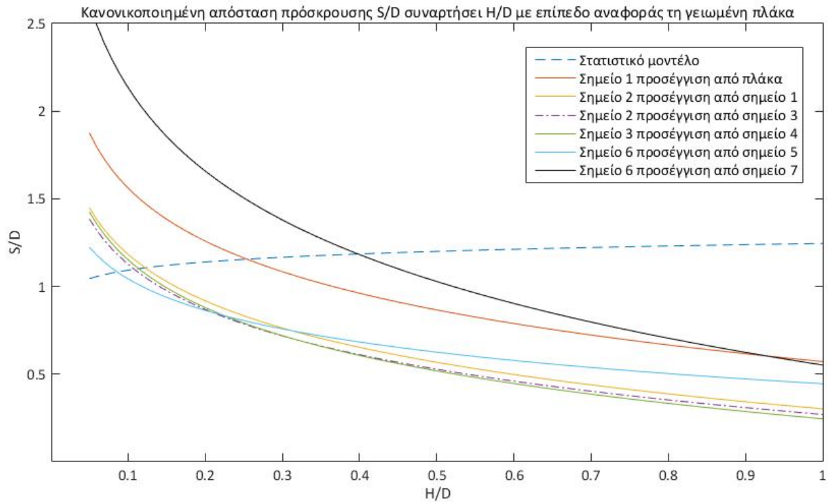
Σχήμα 5.1: Κανονικοποιημένη απόσταση πρόσκρουσης S/D συναρτήσει H/D , όπως αυτή προκύπτει από το στατιστικό μοντέλο και τα εκάστοτε πειραματικά δεδομένα, με επίπεδο αναφοράς τη γειωμένη πλάκα. Αρνητική πολικότητα.
