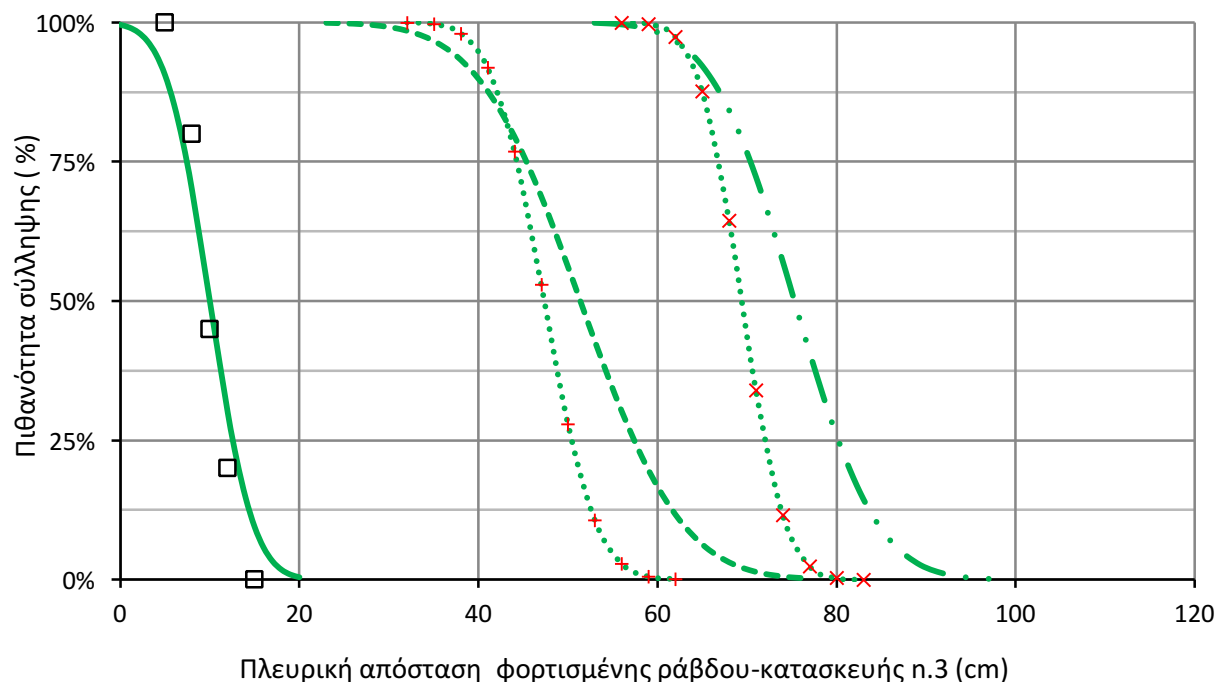
Σχήμα 4.48: Καμπύλες πιθανότητας σύλληψης εκκένωσης από την κατασκευή n.3 του πλοίου, όταν αυτή προσεγγίζεται από την κατασκευή n.4, για απόσταση φορτισμένης ράβδου-πλάκας D=50cm όπως αυτές προκύπτουν από τα πειραματικά δεδομένα και το στατιστικό μοντέλο.
