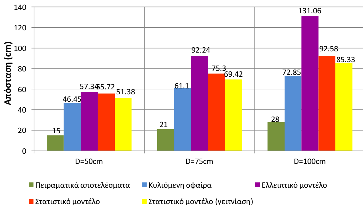
Σχήμα 4.24: Συγκριτικό διάγραμμα των ακτίνων σύλληψης ανά απόσταση φορτισμένης ράβδου-πλάκας, όπου D μετρημένο από το επίπεδο της γειωμένης πλάκας. Αρνητική πολικότητα.
