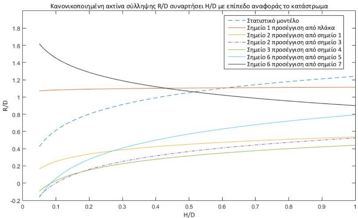
Σχήμα 5.4: Κανονικοποιημένη ακτίνα σύλληψης R/D συναρτήσει H/D , όπως αυτή προκύπτει από το στατιστικό μοντέλο και τα εκάστοτε πειραματικά δεδομένα, με επίπεδο αναφοράς το κατάστρωμα. Αρνητική πολικότητα.
