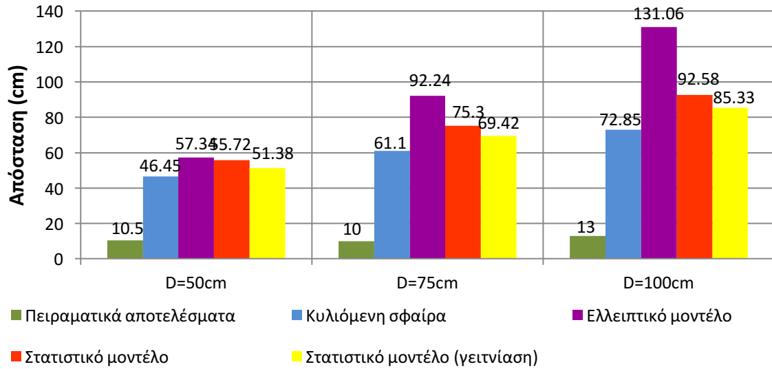
Σχήμα 4.51: Συγκριτικό διάγραμμα των ακτίνων σύλληψης ανά απόσταση φορτισμένης ράβδου-πλάκας, όπου D μετρημένο από το επίπεδο της γειωμένης πλάκας. Αρνητική πολικότητα.
