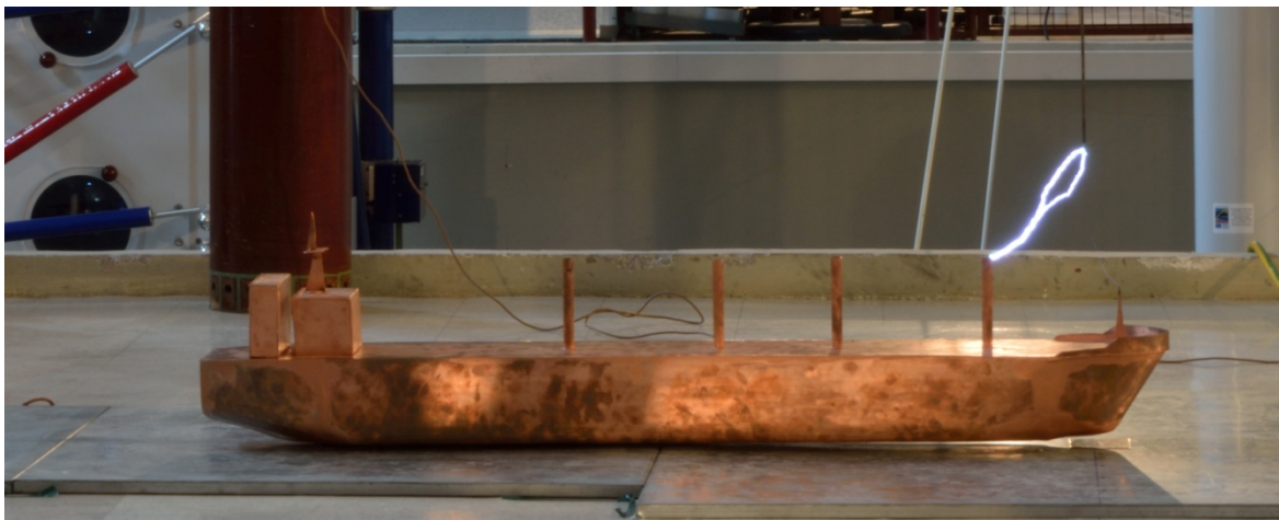
D=50cm, Σύλληψη
