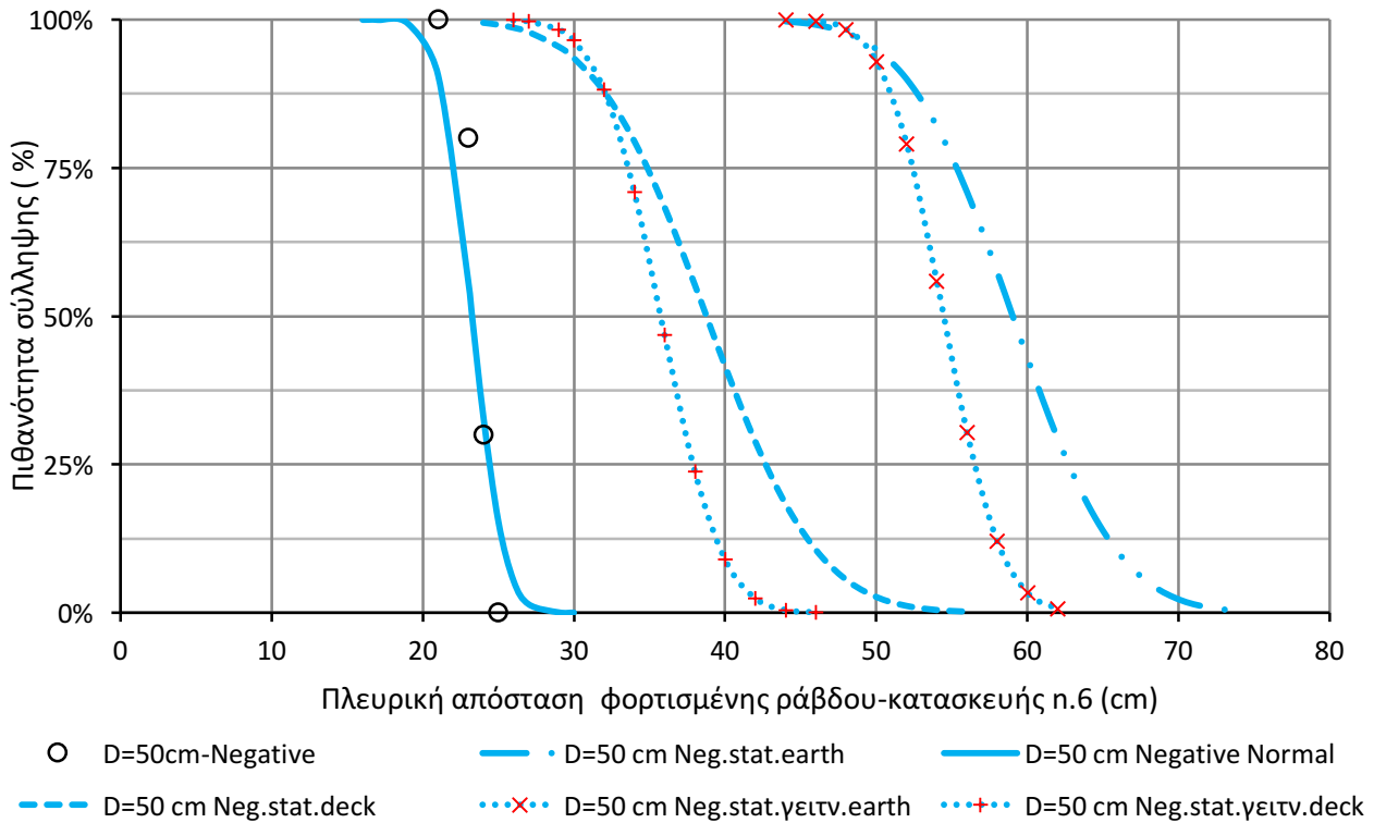
Σχήμα 4.30: Καμπύλες πιθανότητας σύλληψης εκκένωσης από την κατασκευή n.6 του πλοίου, όταν αυτή προσεγγίζεται από την κατασκευή n.5, για απόσταση φορτισμένης ράβδου-πλάκας D=50cm όπως αυτές προκύπτουν από τα πειραματικά δεδομένα και το στατιστικό μοντέλο.
