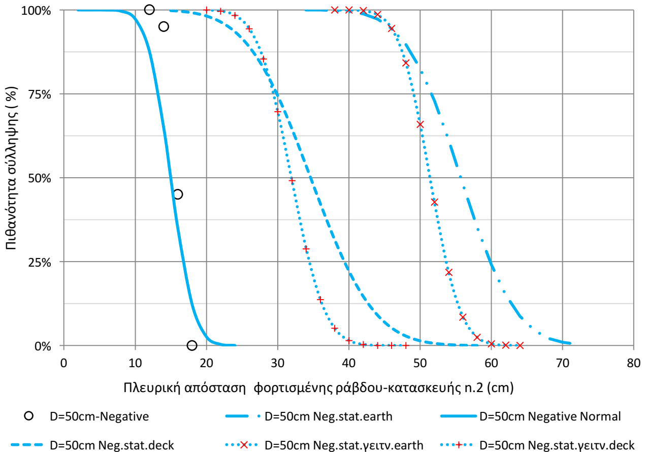
Σχήμα 4.21: Καμπύλες πιθανότητας σύλληψης εκκένωσης από την κατασκευή n.2 του πλοίου, όταν αυτή προσεγγίζεται από την κατασκευή n.1, για απόσταση φορτισμένης ράβδου-πλάκας D=50cm όπως αυτές προκύπτουν από τα πειραματικά δεδομένα και το στατιστικό μοντέλο.
