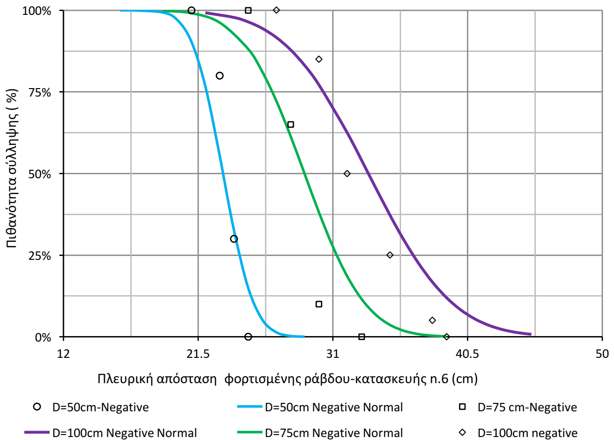
Σχήμα 4.29: Πειραματικές καμπύλες πιθανότητας σύλληψης της εκκένωσης από την κατασκευή n.6 του πλοίου, όταν προσεγγίζεται από την κατασκευή n.5, οι οποίες ακολουθούν κανονική κατανομή.
