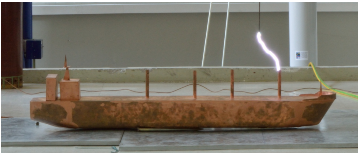
D=50cm Σύλληψη
