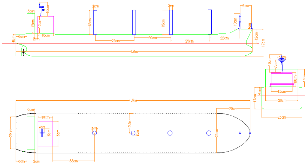
Σχήμα 4.6: Σχέδιο μοντέλου πλοίου σχεδιασμένο μέσω AutoCad.
