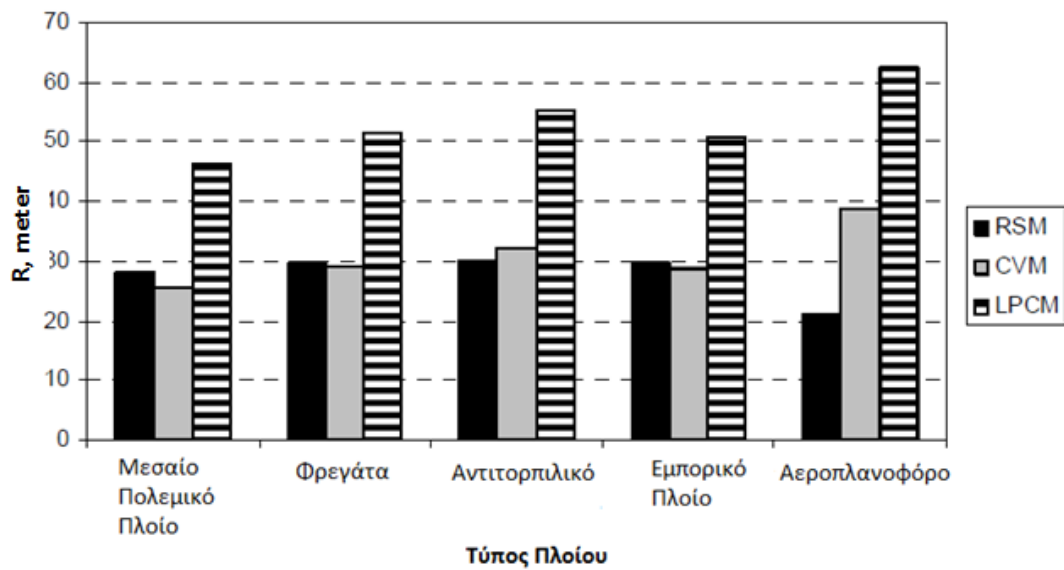
Σχήμα 3.31: Ακτίνα σύλληψης για κάθε είδος πλοίου. Z = 5000\text{m} , I_p = 5.4\text{ kA} [29]
