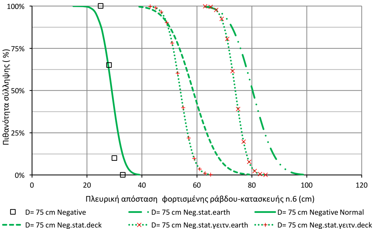
Σχήμα 4.31: Καμπύλες πιθανότητας σύλληψης εκκένωσης από την κατασκευή n.6 του πλοίου, όταν αυτή προσεγγίζεται από την κατασκευή n.5, για απόσταση φορτισμένης ράβδου-πλάκας D=75cm όπως αυτές προκύπτουν από τα πειραματικά δεδομένα και το στατιστικό μοντέλο.
