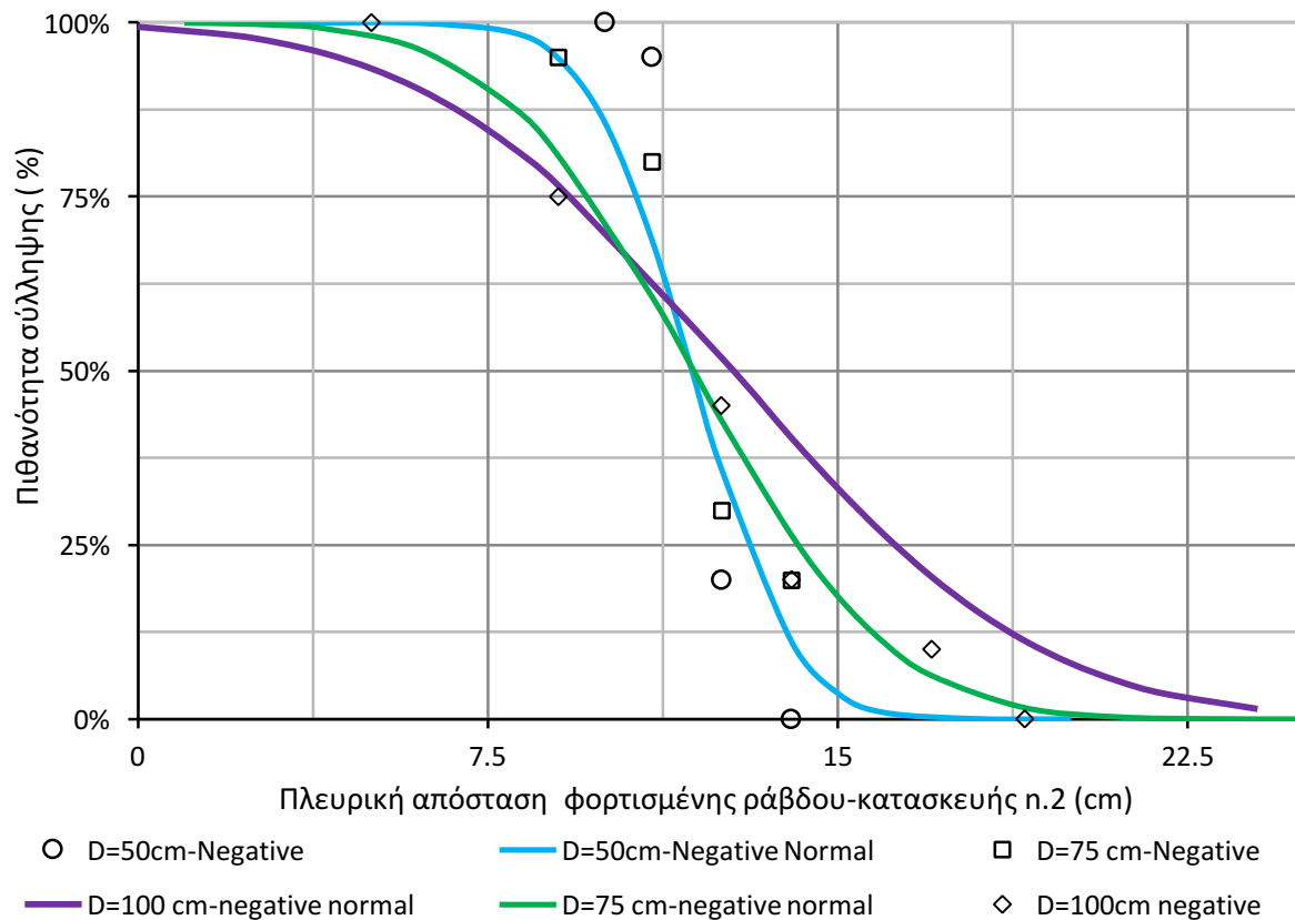
Σχήμα 4.38: Πειραματικές καμπύλες πιθανότητας σύλληψης της εκκένωσης από την κατασκευή n.2 του πλοίου, όταν προσεγγίζεται από την κατασκευή n.3, οι οποίες ακολουθούν κανονική κατανομή.
