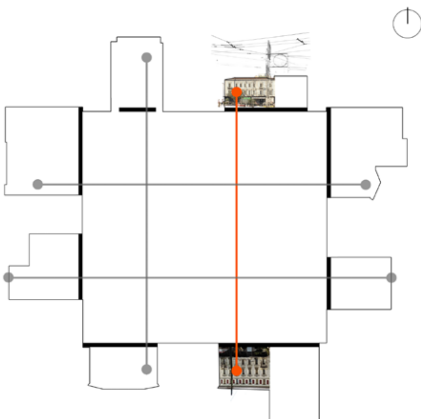
ΑΞΟΝΑΣ 4-4 ' .ΔΙΑΓΡΑΜΜΑ ΚΑΤΟΥΦΗΣ
