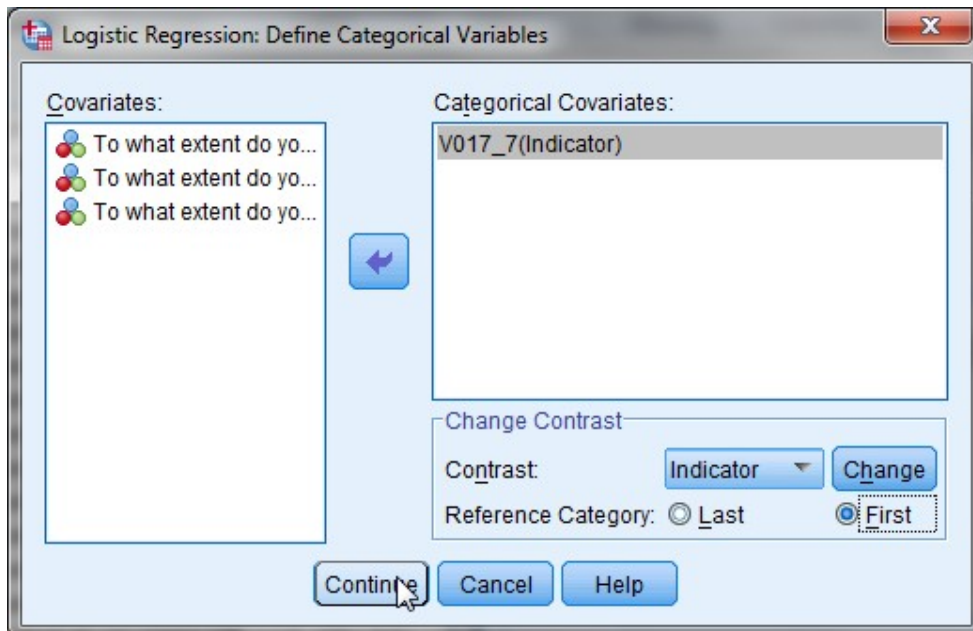
Εικόνα 4.20: Ανάλυση Δυναμικής Λογιστικής Παλινδρόμησης (2)
