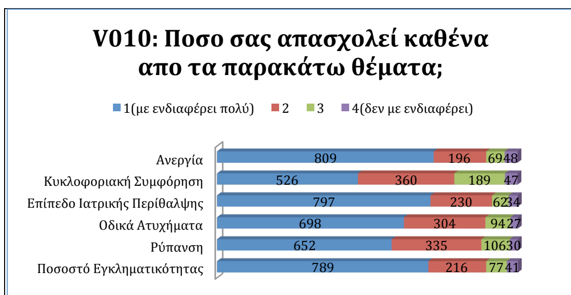
Διάγραμμα 4.4: Κατανομή απαντήσεων για την ερώτηση V010
