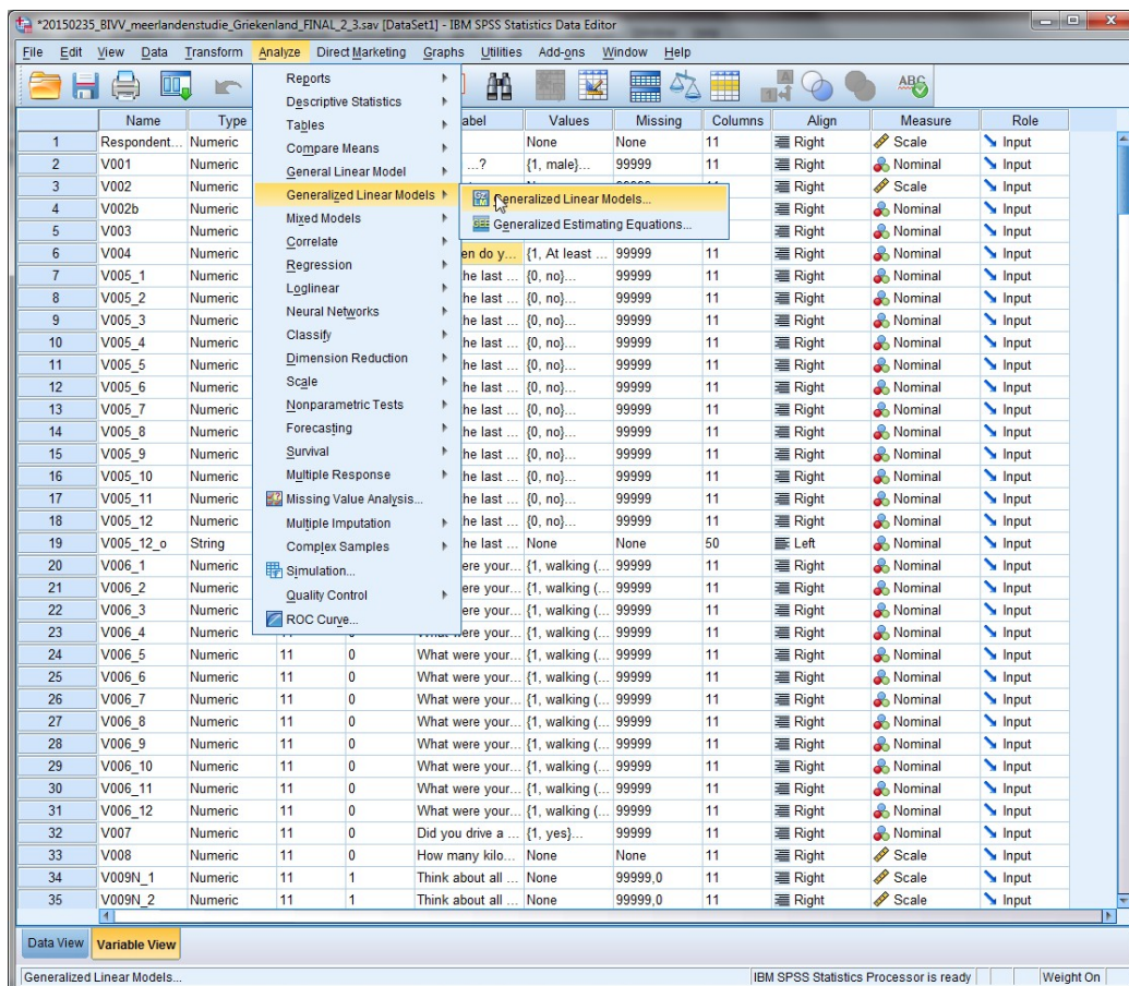
Εικόνα 4.22: Ανάλυση Αρνητικής Διωνυμικής Παλινδρόμησης (1)
