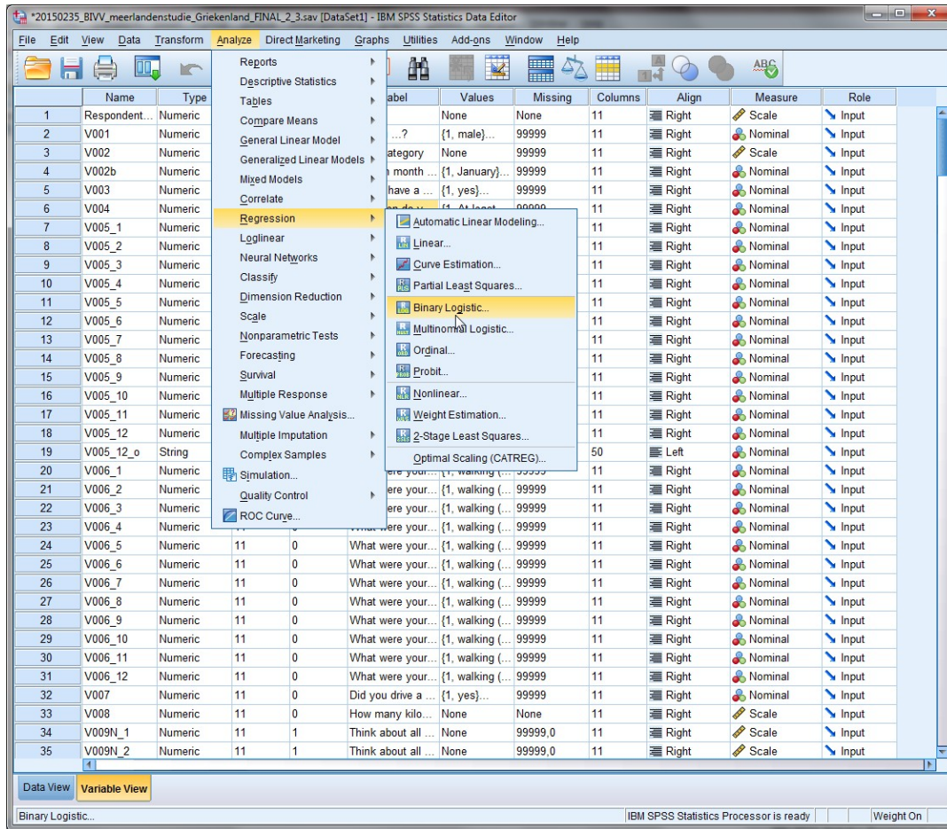
Εικόνα 4.19: Ανάλυση Δυναμικής Λογιστικής Παλινδρόμησης (1)
