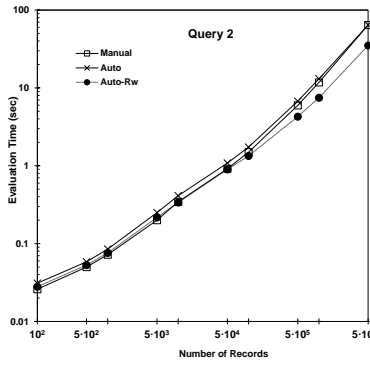
(β) Query 2
