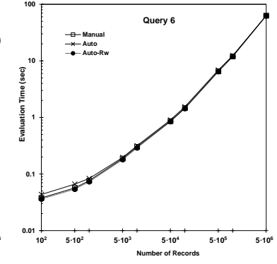
(φ) Query 6
