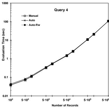
(δ) Query 4
