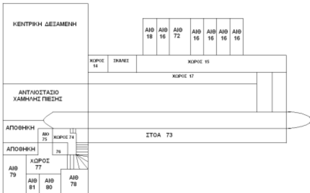
Σχήμα 6.1: Κάτοψη υπογείου.
