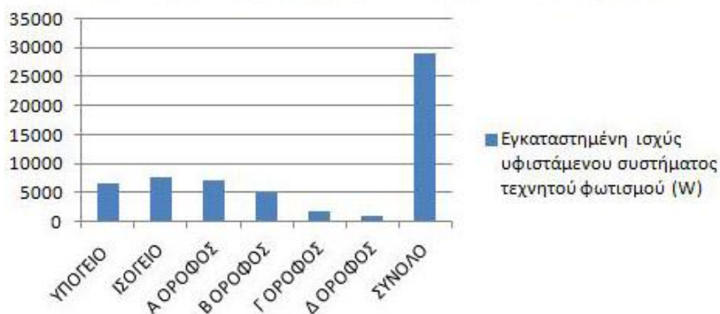
Σχήμα 6.7: Εγκαταστημένη ισχύς υφιστάμενου συστήματος τεχνητού φωτισμού για όλο το κτίριο.
