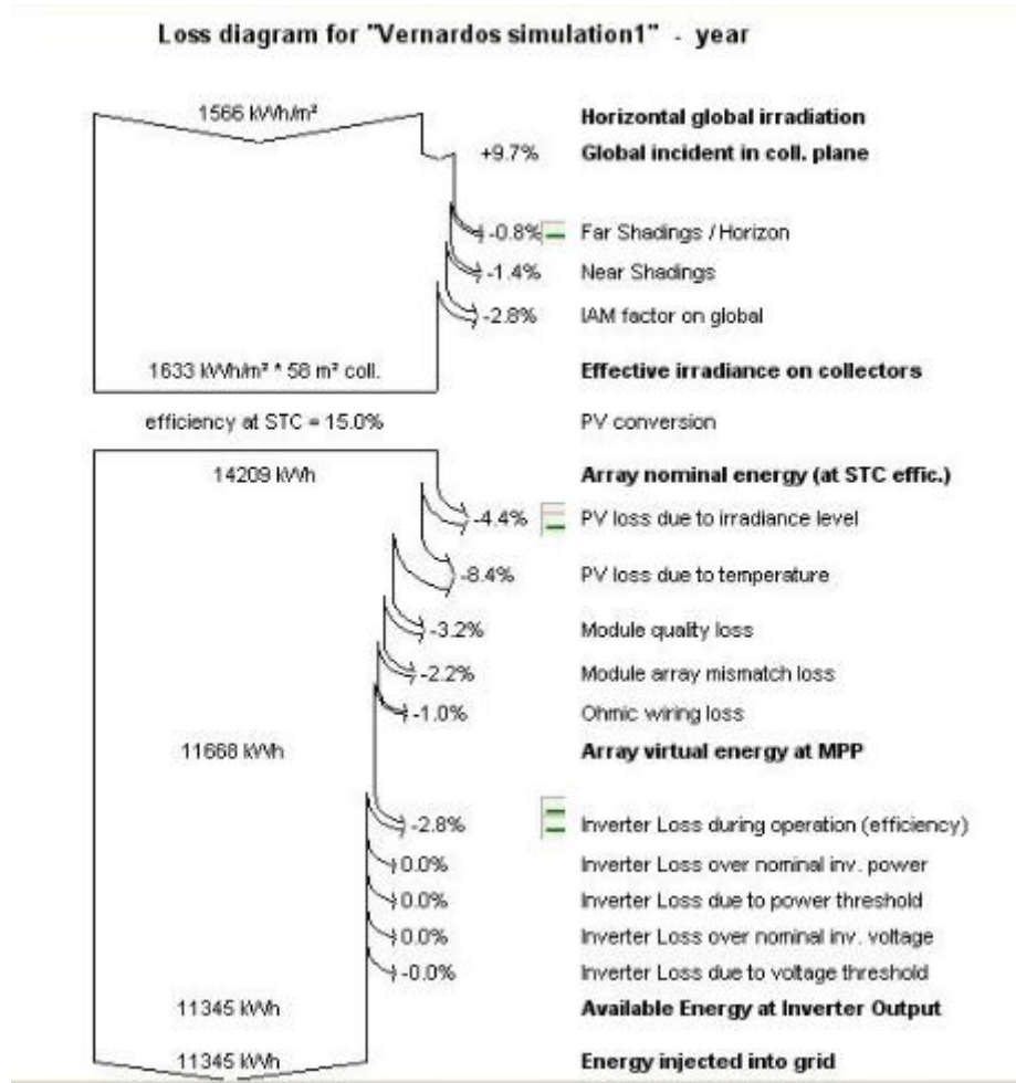
Εικόνα 12.10: Αναλυτικές απώλειες.
