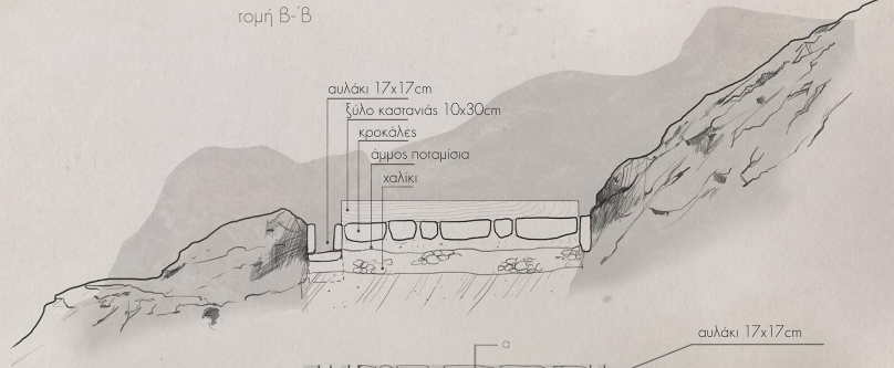
τομή β-β
