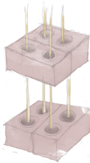
ελεύθερο υποστήλωμα
