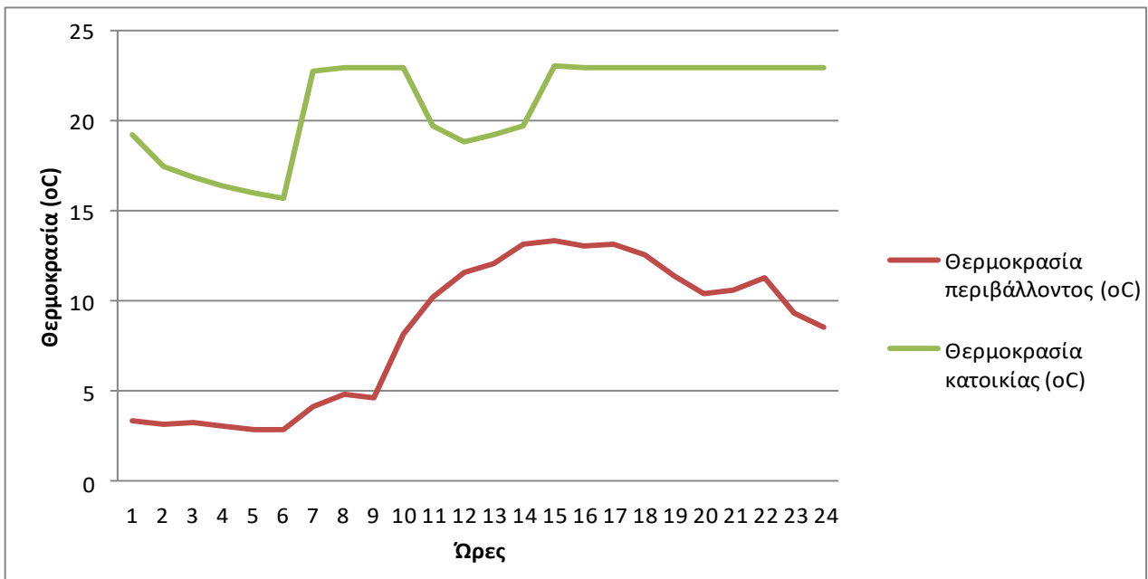
Διάγραμμα 3-3-1 Εσωτερική και εξωτερική θερμοκρασία στις 17 Φεβρουαρίου
