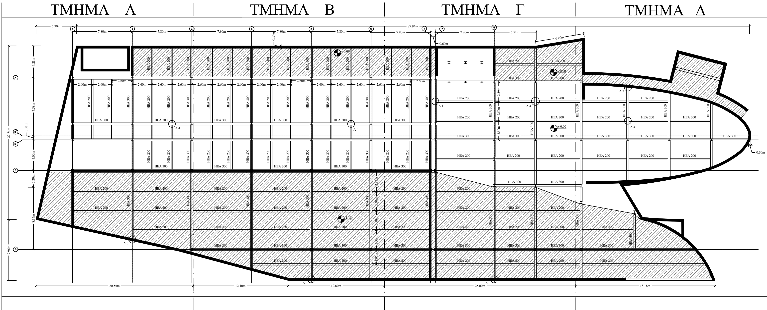
ΕΥΛΟΤΥΠΟΣ ΟΡΟΦΗΣ ΥΠΟΓΕΙΟΥ
