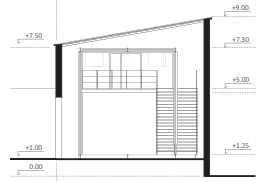
ΤΟΜΗ αα
