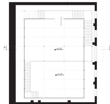
ΚΑΤΟΨΗ Β' ΣΤΑΘΜΗΣ
