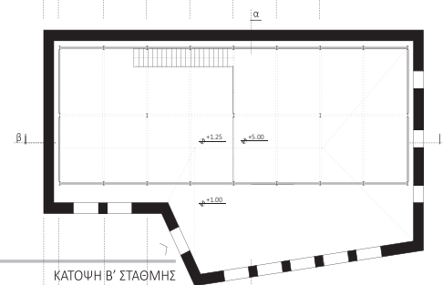
ΚΑΤΟΨΗ Β' ΣΤΑΘΜΗΣ
