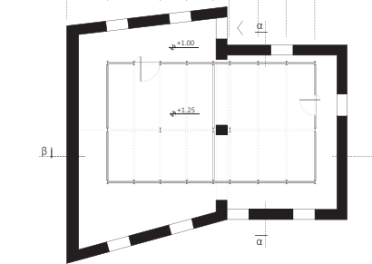
ΚΑΤΟΨΗ Β' ΣΤΑΘΜΗΣ
