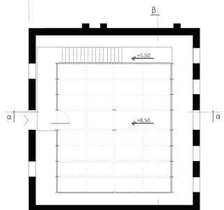
ΚΑΤΟΨΗ Γ' ΣΤΑΘΜΗΣ
