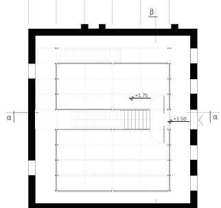
ΚΑΤΟΨΗ Α' ΣΤΑΘΜΗΣ
