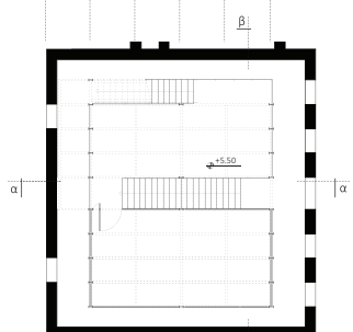
ΚΑΤΟΨΗ Β' ΣΤΑΘΜΗΣ
