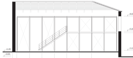
ΤΟΜΗ ββ
