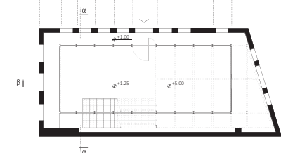
ΚΑΤΟΨΗ Α' ΣΤΑΘΜΗΣ
