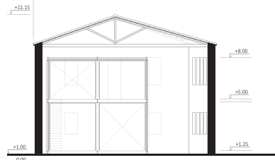
ΤΟΜΗ αα
