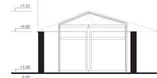
ΤΟΜΗ αα
