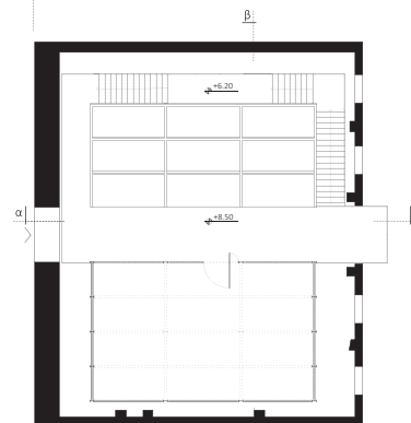
ΚΑΤΟΨΗ Γ' ΣΤΑΘΜΗΣ
