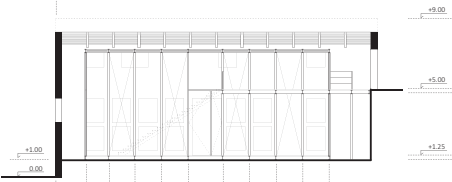
ΤΟΜΗ ββ
