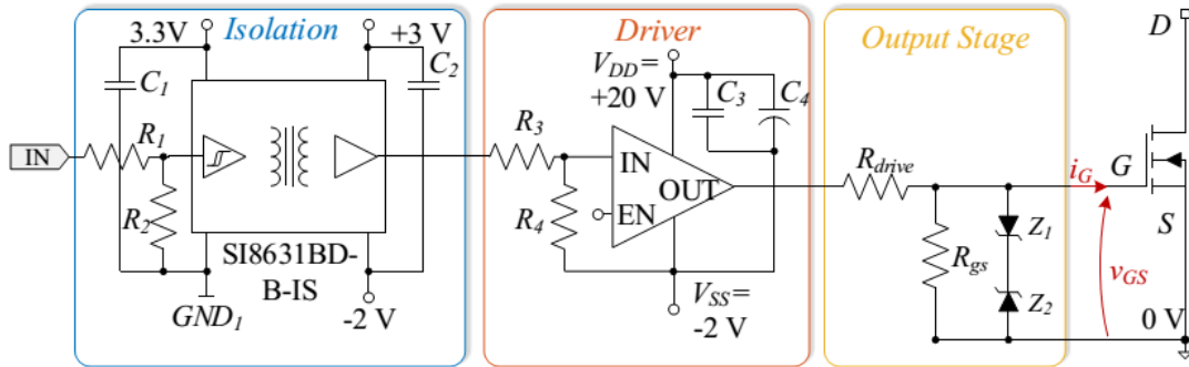
Σχήμα 3.2 Σχηματικό διάγραμμα του υλοποιημένου κυκλώματος οδήγησης SiC Mosfet [26]
