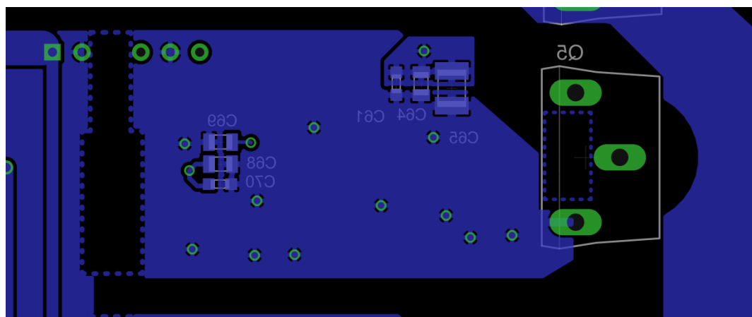
Σχήμα 3.4 Άνοψη σχεδιασμένου κυκλώματος οδήγησης SiC Mosfet
