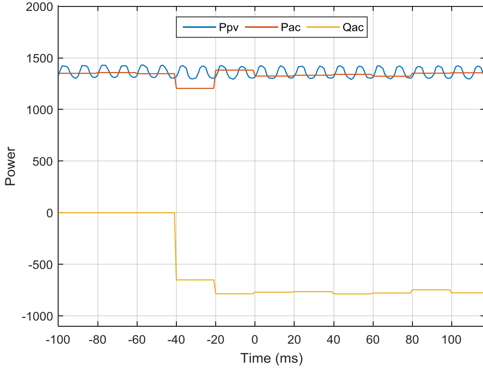
Σχήμα 5.44 Ισχύς Φ/Β ( P_{pv} ), Ενεργός Ισχύς εξόδου ( P_{ac} ) και Άεργος Ισχύς εξόδου ( Q_{ac} ) μεταβάλλοντας της άεργο ισχύ (0-600Var σε 1m/s)
