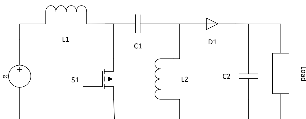
Σχήμα 2.18 Κυκλωματικό διάγραμμα Sepic μετατροπέα
