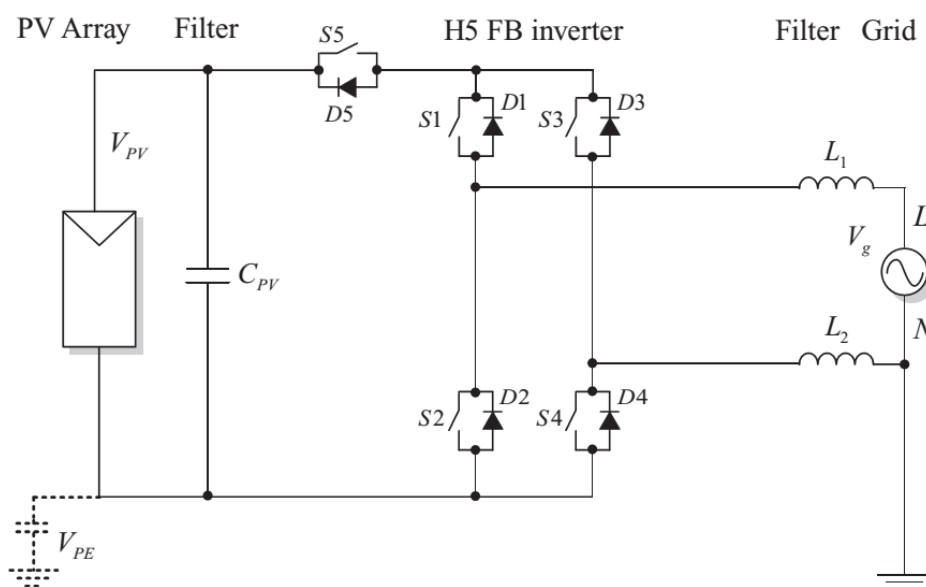
Σχήμα 2.5 H5 τοπολογία αντιστροφέα (SMA) [6]
