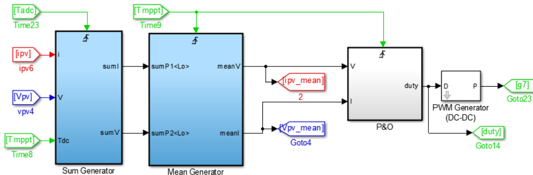
Σχήμα 5.8 Δομικό διάγραμμα για την υλοποίηση του MPPT στο Simulink
