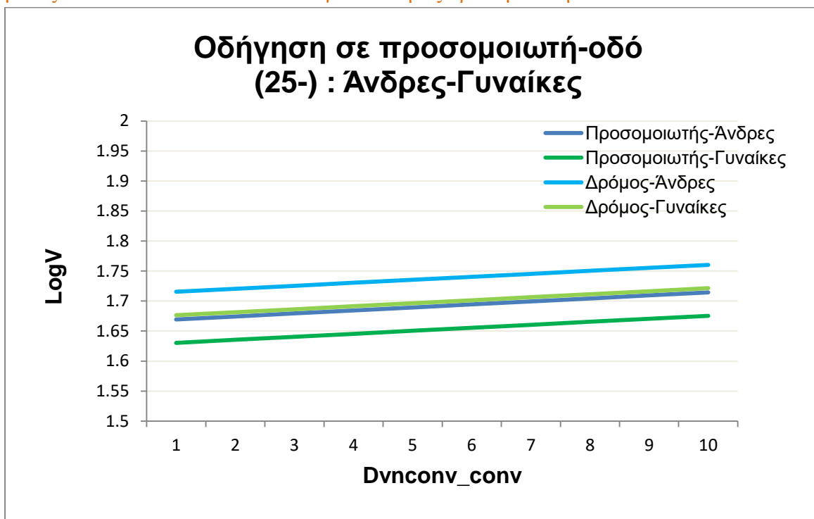
Διάγραμμα 6.22 : Συσχέτιση μέσης ταχύτητας με την διαφορά ταχυτήτων με και χωρίς ομίλια μεταξύ των νέων κάτω των 25 ετών για συνθήκες προσομοιωτή και οδού
