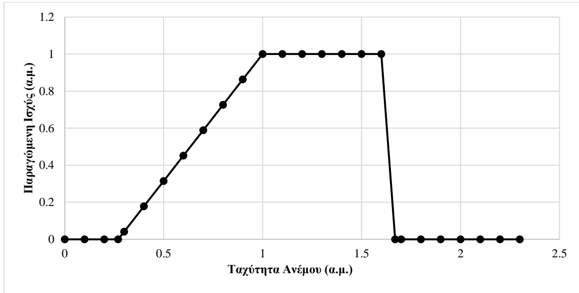
Σχήμα 4.2: Παραγόμενη Ισχύς Ανεμογεννήτριας Συναρτήσει της Ταχύτητας του Ανέμου
