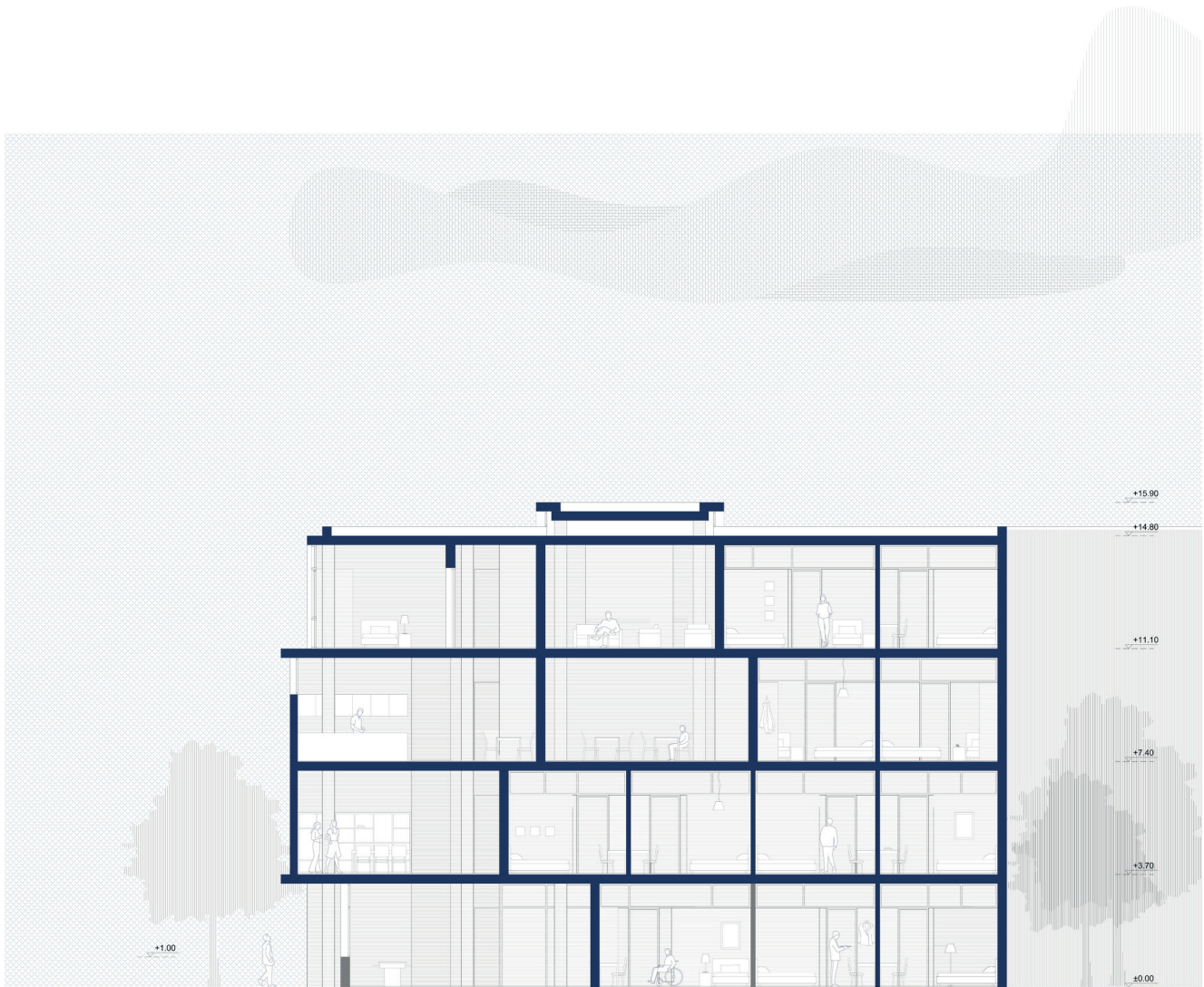
τομή Β-Β
