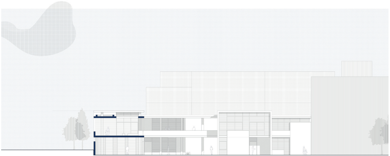
τομή A-A
