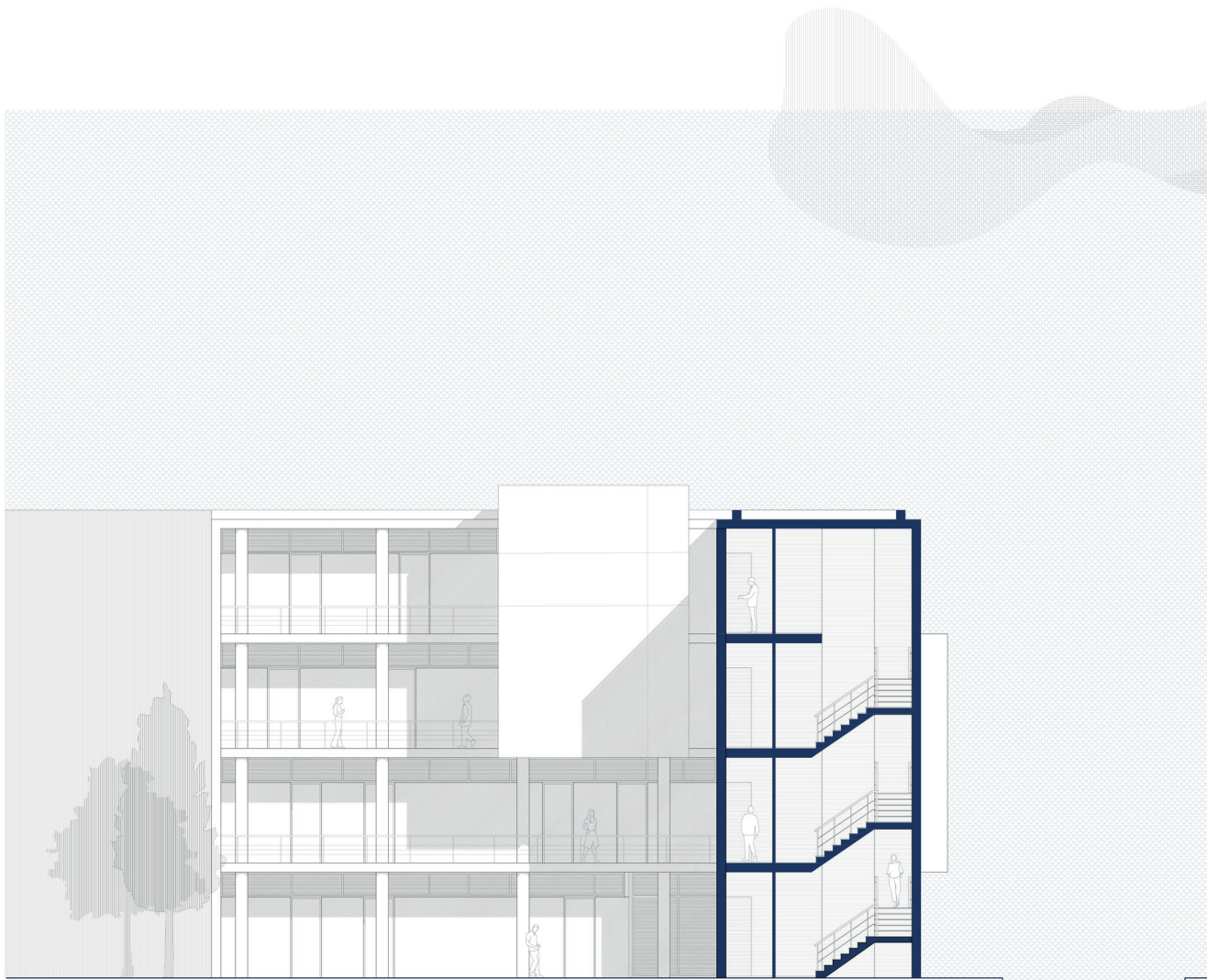
δυτική όψη
