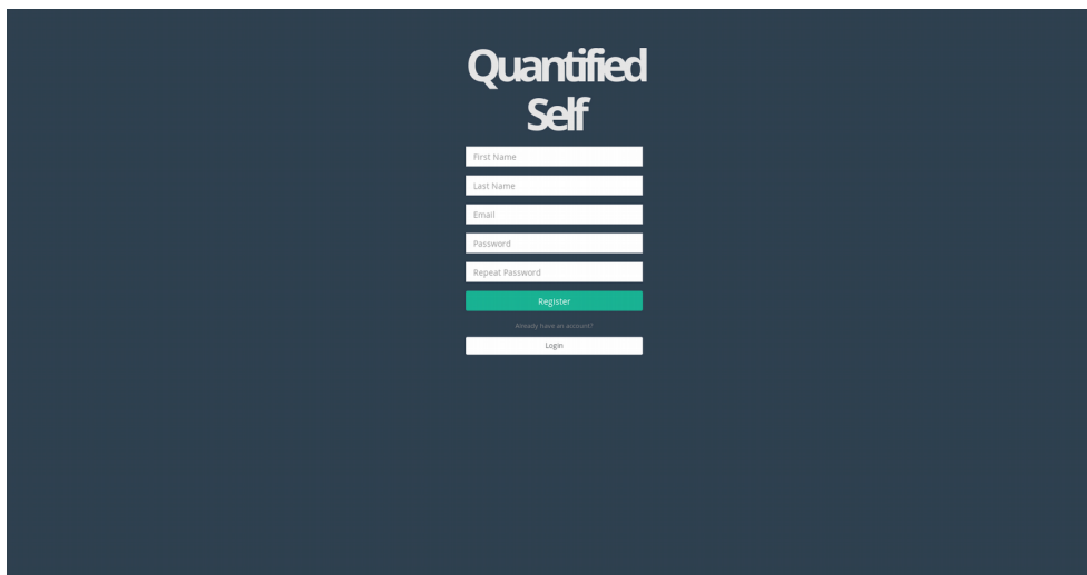
Σχήμα 75: Register Page
