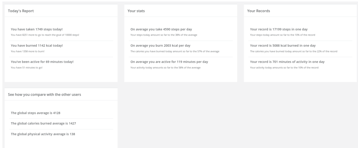
Σχήμα 101: Ανανεωμένο Homepage
