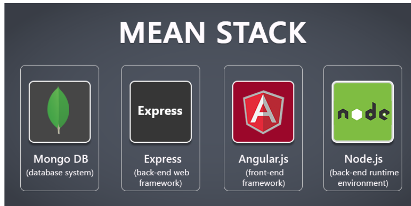
Σχήμα 8: MEAN Stack
