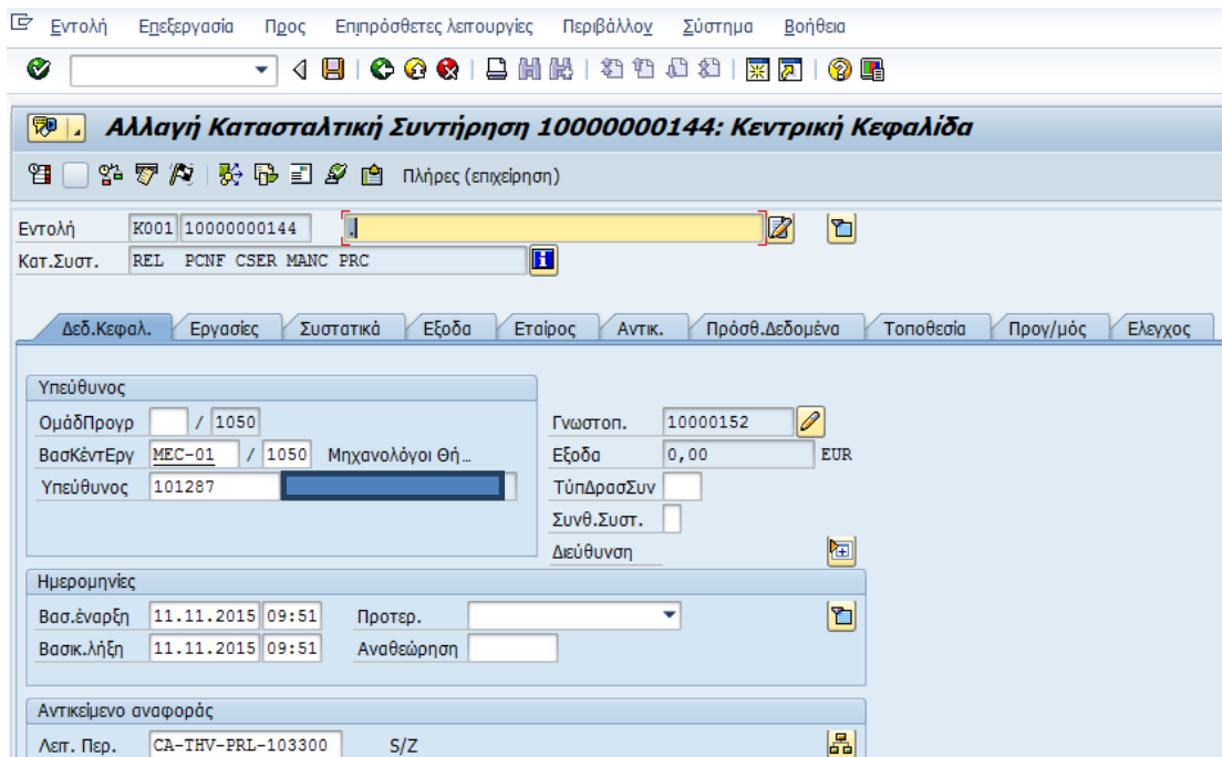
Εικόνα 65: Ολοκλήρωση εργασιών συντήρησης εικ.1
