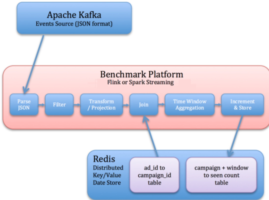
Figure 3.3: Επειμέρους λειτουργίες σεναρίου
