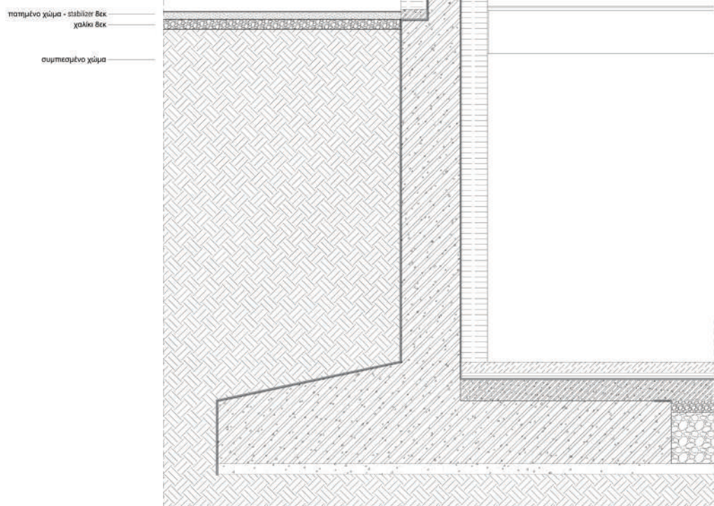
κατασκευαστική τομή κλ. 1:20
