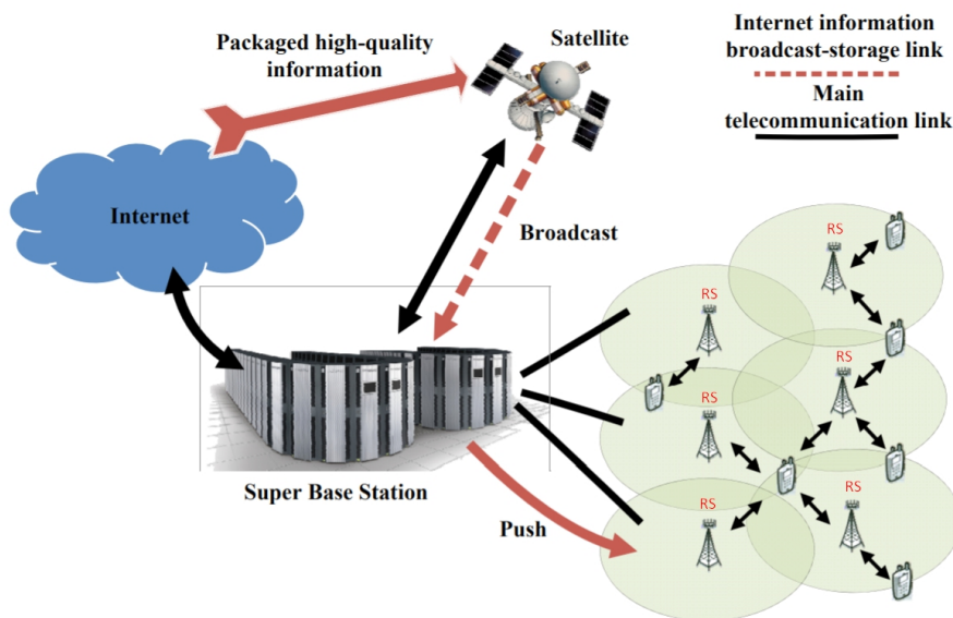
Σχήμα 2.2: Αρχιτεκτονική του προς σχεδίαση τηλεπικοινωνιακού δικτύου.
