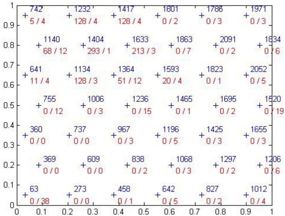
Σχήμα 6.9: Εναπομείναντες πόροι και μη εξυπηρετηθέντες χρήστες στην πρώτη υλοποίηση του τρίτου σεναρίου με δυνατότητα ανακατανομής πόρων με depthmax = 0 και μέγεθος δείγματος ίσο με 170 χρήστες. Με μπλε αναγράφεται ο αριθμός των πόρων που κατανεμήθηκαν αρχικά σε κάθε ισχυρό κόμβο, ενώ με κόκκινο αναγράφονται ο αριθμός εναπομεινάντων πόρων (αριστερά) και ο αριθμός μη εξυπηρετηθέντων χρηστών (δεξιά).
