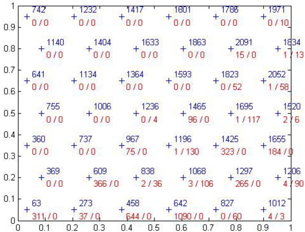
Σχήμα 5.16: Εναπομεινάντες πόροι και μη εξυπηρετηθέντες χρήστες στην πρώτη υλοποίηση του δεύτερου σεναρίου με δυνατότητα ανακατανομής πόρων με depthmax = 0 . Με μπλε αναγράφεται ο αριθμός των πόρων που κατανεμήθηκαν αρχικά σε κάθε ισχυρό κόμβο, ενώ με κόκκινο αναγράφονται ο αριθμός εναπομεινάντων πόρων (αριστερά) και ο αριθμός μη εξυπηρετηθέντων χρηστών (δεξιά).
