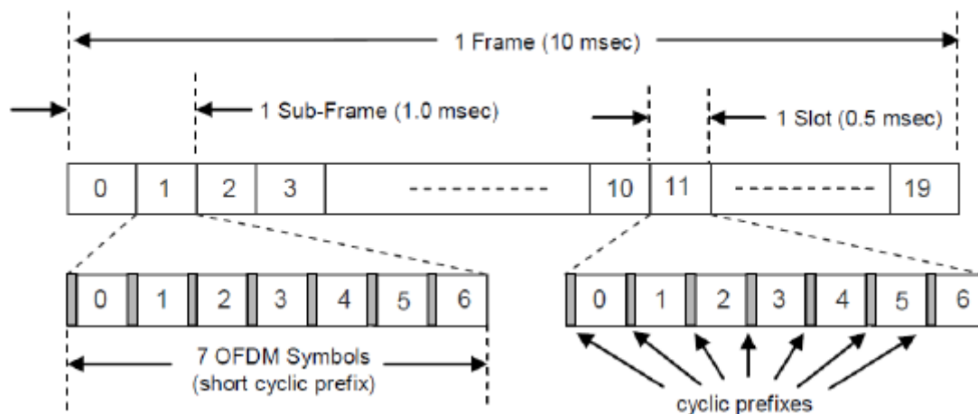
Σχήμα 7.1: Δομή πλαισίου στο LTE (LTE frame structure)
