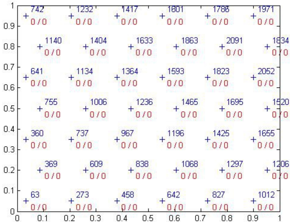
Σχήμα 5.4: Εναπομείναντες πόροι και μη εξυπηρετηθέντες χρήστες στην πρώτη υλοποίηση του πρώτου σεναρίου με depthmax = 5. Με μπλε αναγράφεται ο αριθμός των πόρων που κατανεμήθηκαν αρχικά σε κάθε ισχυρό κόμβο, ενώ με κόκκινο αναγράφονται ο αριθμός εναπομεινάντων πόρων (αριστερά) και ο αριθμός μη εξυπηρετηθέντων χρηστών (δεξιά).
