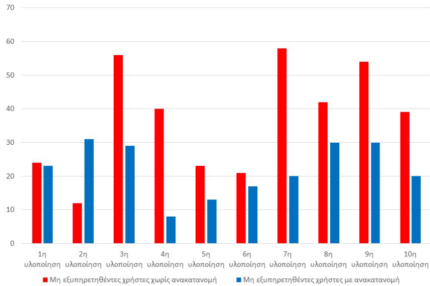
Σχήμα 5.23: Μη εξυπηρετηθέντες χρήστες σε καθεμιά από τις 10 υλοποιήσεις ( seednumber=55 ) του δεύτερου σεναρίου προσομοίωσης με (οι μπλε στήλες) και χωρίς (οι κόκκινες στήλες) δυνατότητα ανακατανομής πόρων και depthmax = 1 .
