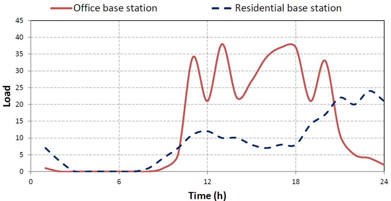
Σχήμα 2.5: Ημερήσιο φορτίο σταθμών βάσης σε περιοχές εργασίας (Office BS) και σε περιοχές κατοικίας (Residential BS).
