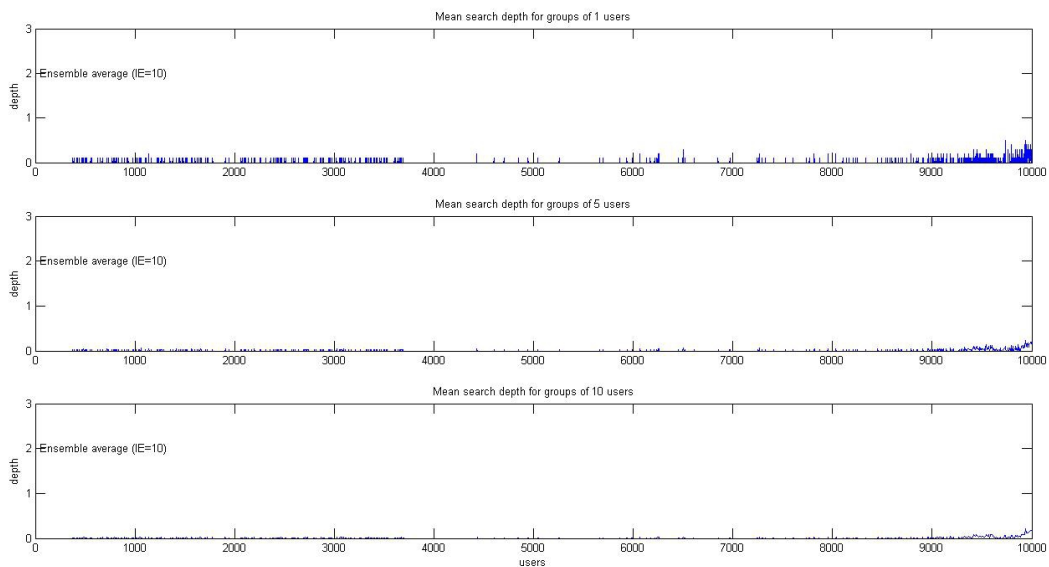
Σχήμα 7.15: Μέσο βάθος αναζήτησης ανά χρήστη που προέκυψε από τις 10 υλοποιήσεις του δεύτερου σεναρίου με δυνατότητα ανακατανομής πόρων, με διαφοροποίηση υπηρεσιών και με δυνατότητα προσαρμογής σε αλλαγές προτίμησης των 3 τύπων υπηρεσιών. Στο μεσαίο και στο κάτω διάγραμμα τα αποτελέσματα ομαδοποιούνται ανά 5 και 10 χρήστες αντίστοιχα.
