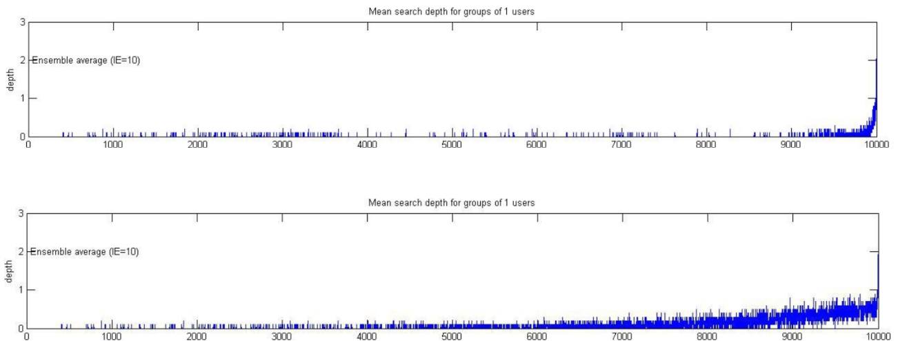
Σχήμα 5.21: Μέσο βάθος αναζήτησης ανά χρήστη που προέκυψε από τις 10 υλοποιήσεις του δεύτερου σεναρίου με δυνατότητα ανακατανομής πόρων, με (πάνω διάγραμμα) και χωρίς (κάτω διάγραμμα) δυνατότητα καλύτερης προσέγγισης στατικής κατανομής.
