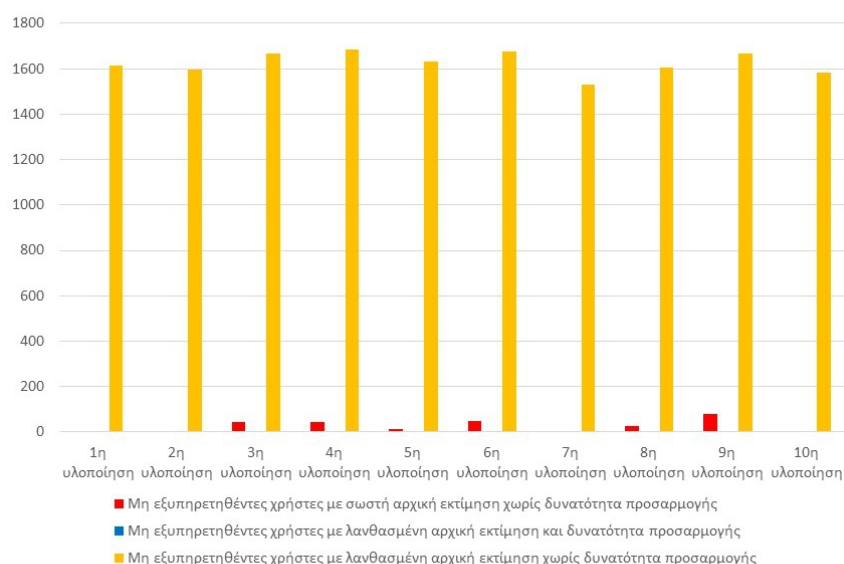
Σχήμα 7.14: Μη εξυπηρετηθέντες χρήστες σε καθεμία από τις 10 υλοποιήσεις του δεύτερου σεναρίου
