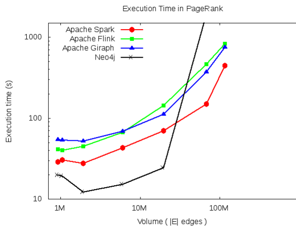
Σχήμα 5.7: Χρόνος εκτέλεσης του τελεστή Page Rank
