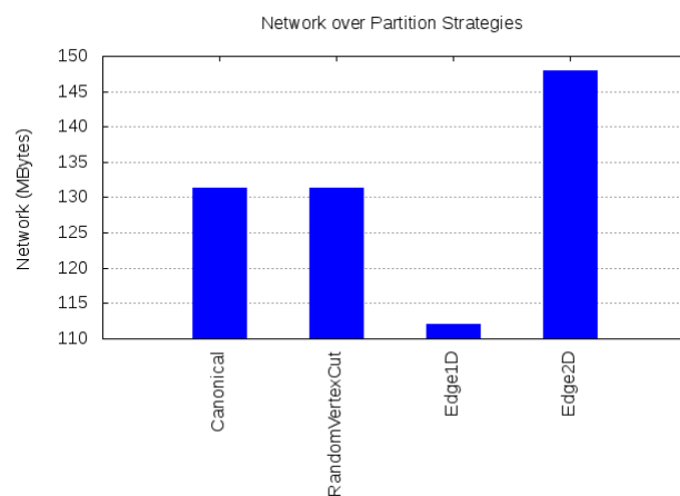
Σχήμα 5.30: Η χρήση του δικτύου του GraphX για διαφορετικές στρατηγικές καταμερισμού.
