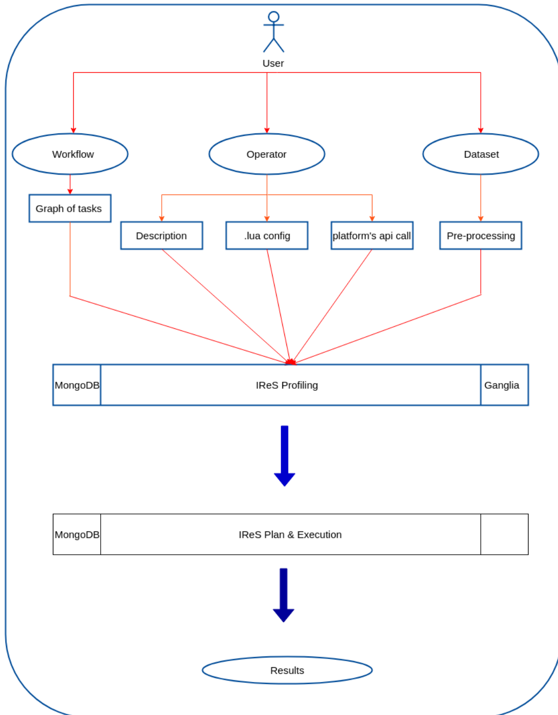
Σχήμα 5.6: Η ροή διεξαγωγής των πειραμάτων
