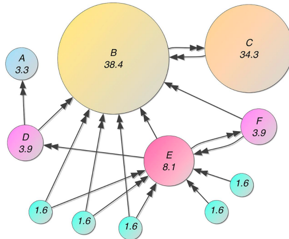
Σχήμα 5.1: Ο αλγόριθμος PageRank. Η σημαντικότητα του κόμβου B εξαρτάται τόσο από το πλήθος των κόμβων που αναφέρουν τον κόμβο B καθώς επίσης και την ποιότητα των κόμβων που τον αναφέρουν.
