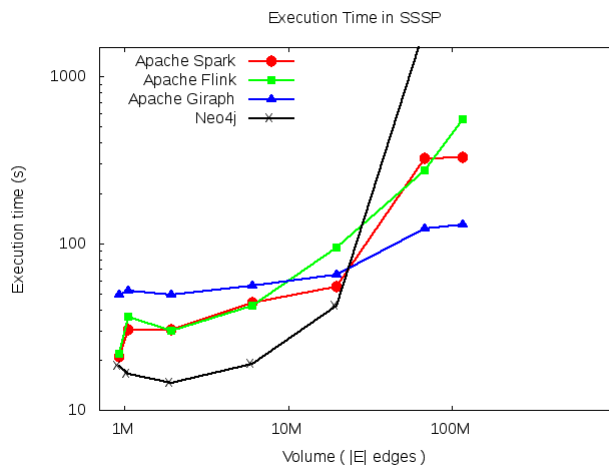
Σχήμα 5.9: Χρόνος εκτέλεσης του τελεστή SSSP
