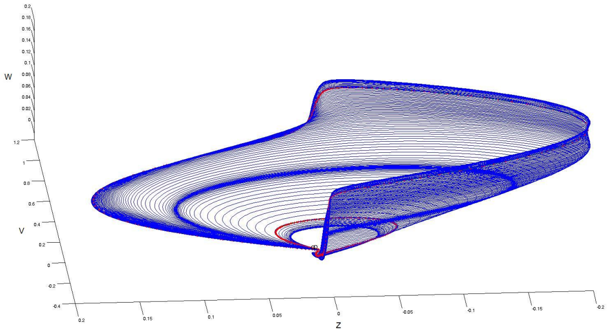
Εικόνα 4.1.3: Σύνολο ομοκλιτικών τροχιών του συστήματος (4.1), στην περίπτωση \varepsilon = 0,005 . Κάθε τέτοια τροχιά θα αντιστοιχεί σε ένα σημείο του από πάνω διαγράμματος διακλάδωσης, με τις ερυθρές τροχιές να αντιστοιχούν στα ερυθρά σημεία.
