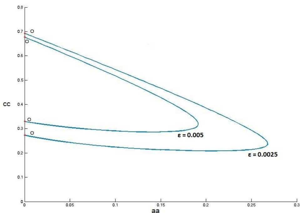
Εικόνα 4.1.4: Ομοκλιτικές καμπύλες διακλάδωσης για δύο διαφορετικές τιμές της παραμέτρου \varepsilon .
