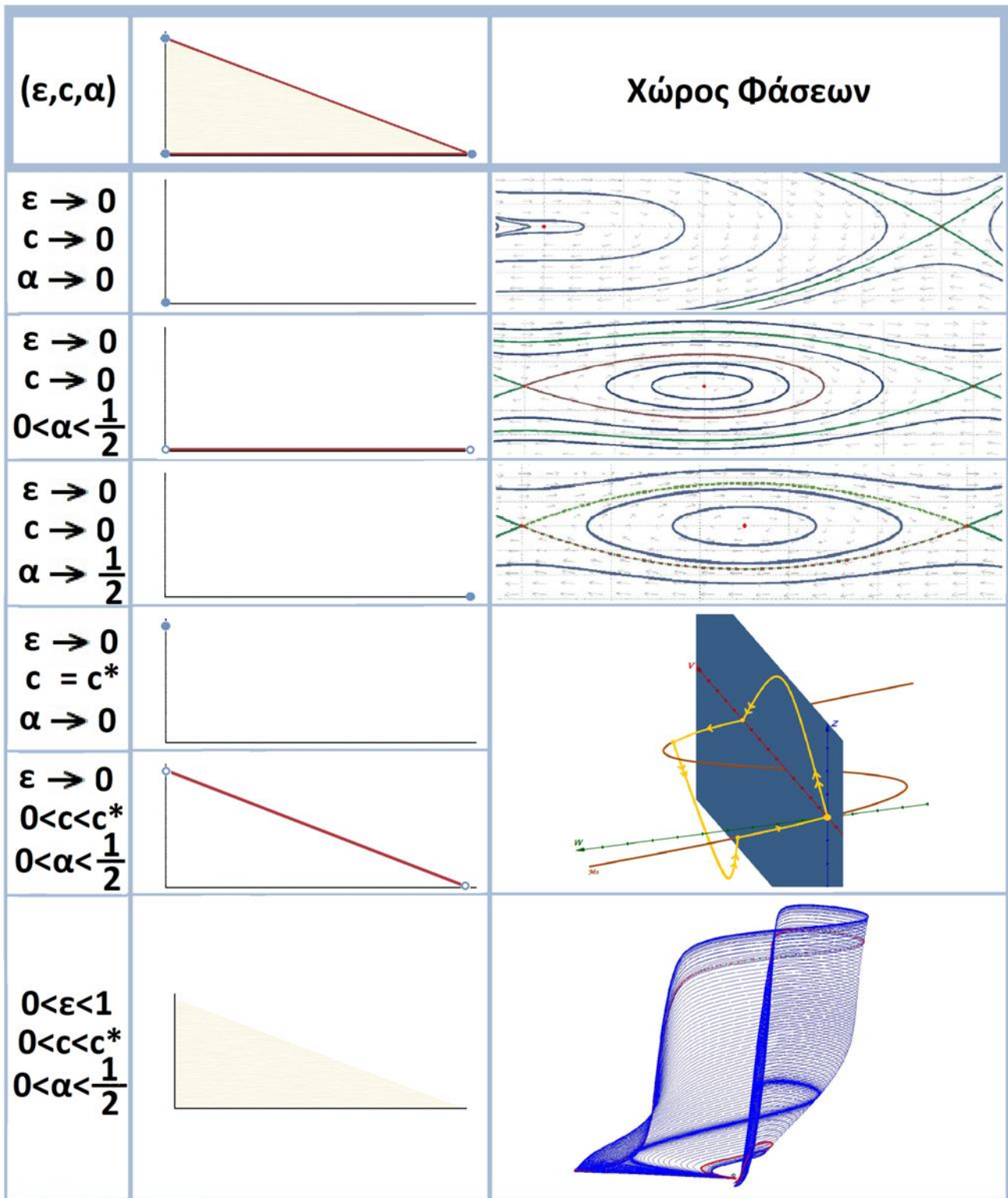
Εικόνα 4.1.8: Συγκεντρωτικός πίνακας. Στην πρώτη στήλη φαίνονται οι τιμές των παραμέτρων \epsilon, c, \alpha , με τις αντίστοιχες θέσεις τους στο επίπεδο a, c (δεύτερη στήλη). Τέλος στην τρίτη στήλη απεικονίζεται η κατά περίπτωση διαμόρφωση του χώρου φάσεων με έμφαση κυρίως στην σχεδίαση των ομοκλικών τροχιών.
