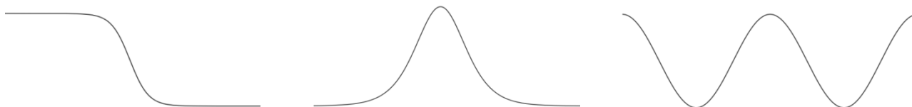
Εικόνα 2.1.1: Μορφές οδεύοντων κυμάτων. Διαδοχικά απεικονίζονται το μέτωπο οδεύον κύμα, ο παλμός και ο περιοδικός κυματισμός.
