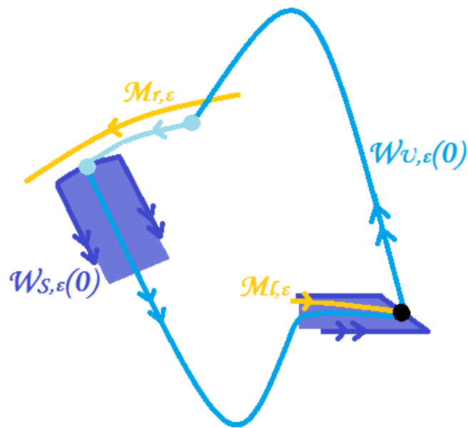
Εικόνα 3.3.5: Σχηματική αναπαράσταση της διαταραγμένης ομοκλιτικής τροχιάς.
