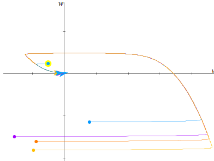
Εικόνα 2.2.2: Χώρος φάσεων για πέντε διαφορετικές αρχικές συνθήκες του συστήματος, οι τροχιές των οποίων προσεγγίζουν την αρχή των αξόνων.
