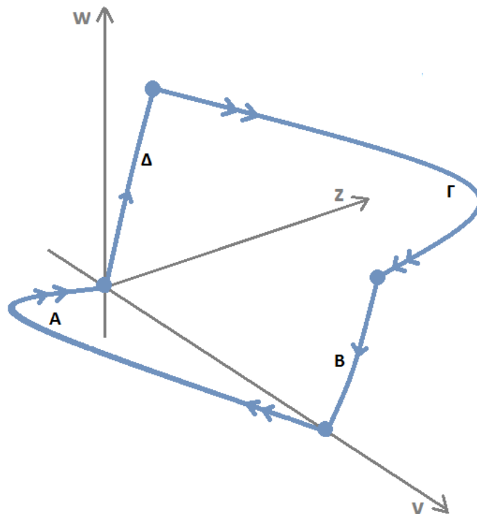
Εικόνα 1.2.2: Η ομοκλινική τροχιά στο χώρο φάσεων, με τις αντίστοιχες περιοχές της προηγούμενης εικόνας να σημειώνονται.
