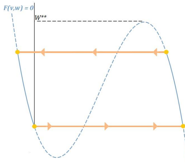
Εικόνα 2.3.4: Πορτρέτο της ομοκλιτικής τροχιάς. Η τροχιά ξεκινά από την αρχή των αξόνων κινούμενη προς τα δεξιά. Έπειτα ανέρχεται στην V_+ έως ότου φθάσει στο σημείο \tilde{W} , όπου τότε θα κινηθεί προς τα αριστερά και μέσω της V_- θα καταλήξει από όπου ξεκίνησε.
