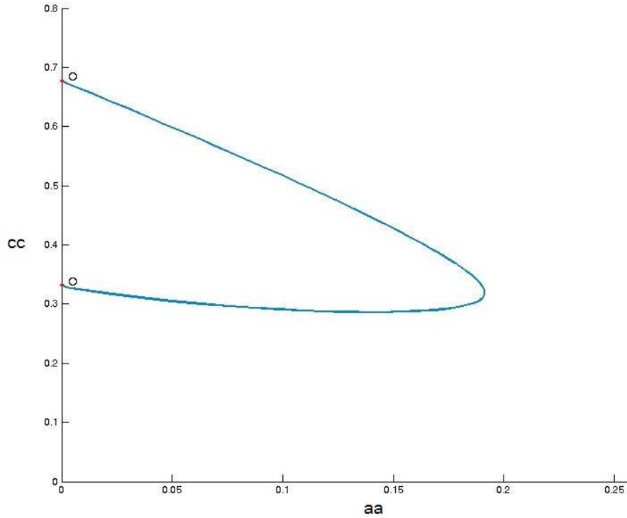
Εικόνα 4.1.2: Καμπύλη ομοκλιτικής διακλάδωσης στο επίπεδο a - c (στο διάγραμμα, aa-cc αντίστοιχα), στην περίπτωση όπου \varepsilon = 0,005 .
