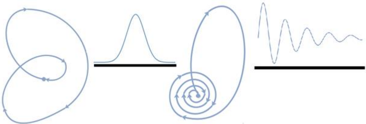
Εικόνα 4.1.1: Μορφές ομοκλινικών τροχιών στην περίπτωση σαγματικού σημείου ισορροπίας (αριστερά) και στην περίπτωση σαγματικής εστίας (δεξιά).
