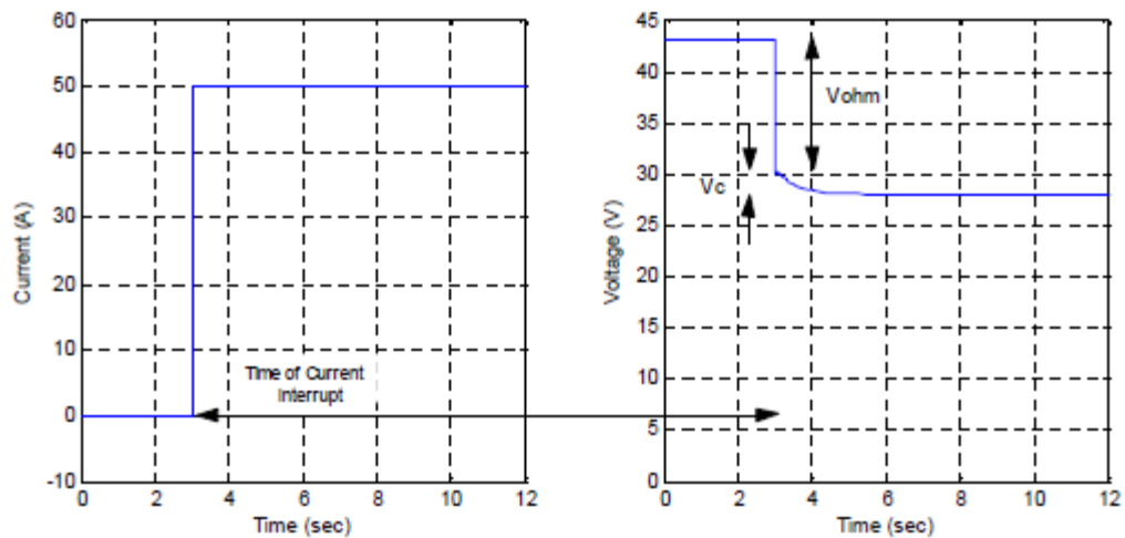
Σχήμα 4.6 Μέθοδος διακοπής ρεύματος.
