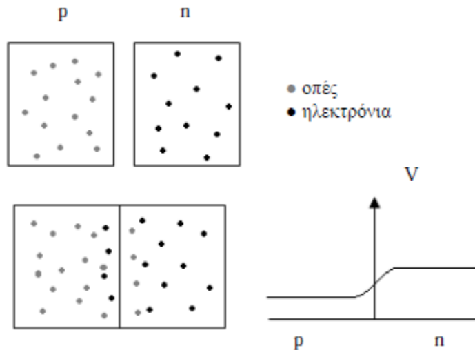
Σχήμα 3.7 Φαινόμενο διπλού στρώματος p-n.
