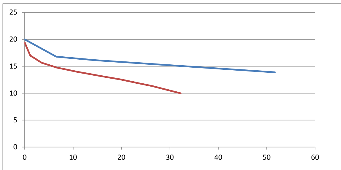
Διάγραμμα 5.1 Διάγραμμα τάση-ρεύμα κατασκευαστή(μπλε) – μετρούμενο V-I(κόκκινο) [21].
