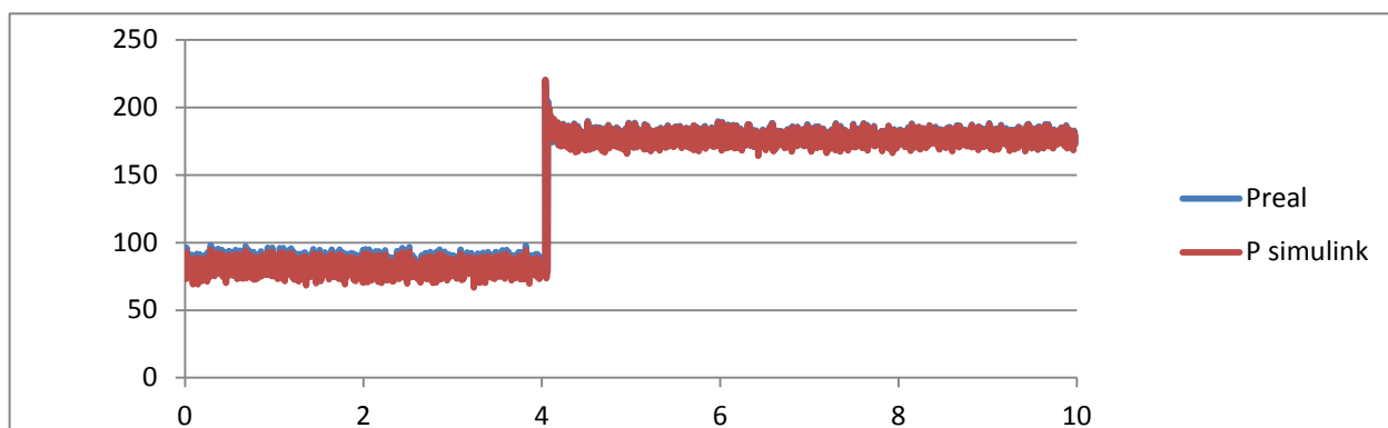
Διάγραμμα 5.14 Μετρούμενη-προσομοιωμένη Ισχύς σε Watt.
