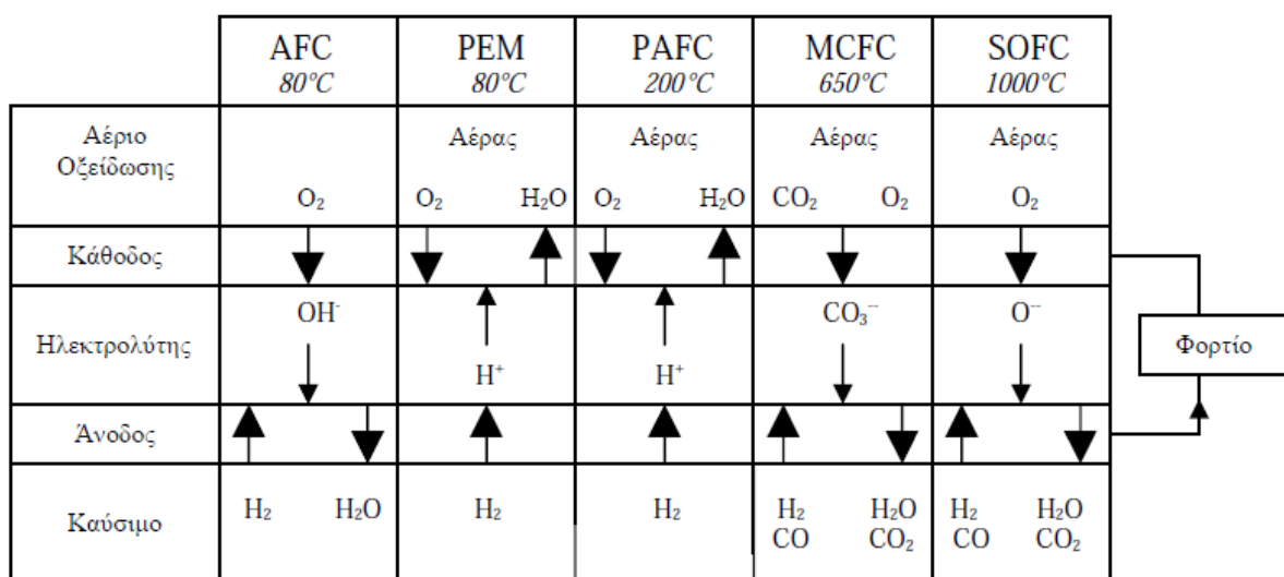
Σχήμα 2.7 Η δομή των διαφόρων τύπων κυψελών καυσίμου[2].
