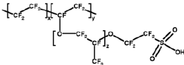
Σχήμα 3.3 Δομή του πολυμερές Nafion ( C_7HF_{13}O_5S C_2F_4 )[1]
