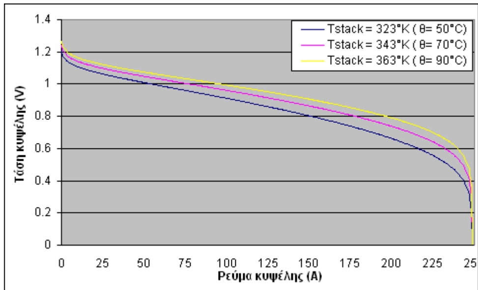
Διάγραμμα 4.1 Αναμενόμενες χαρακτηριστικές για διάφορες θερμοκρασίες λειτουργίας [3].
