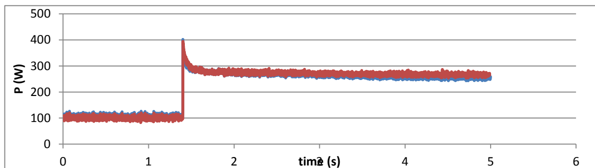
Διάγραμμα 5.17 Μετρούμενη-προσομοιωμένη Ισχύς σε Watt.
