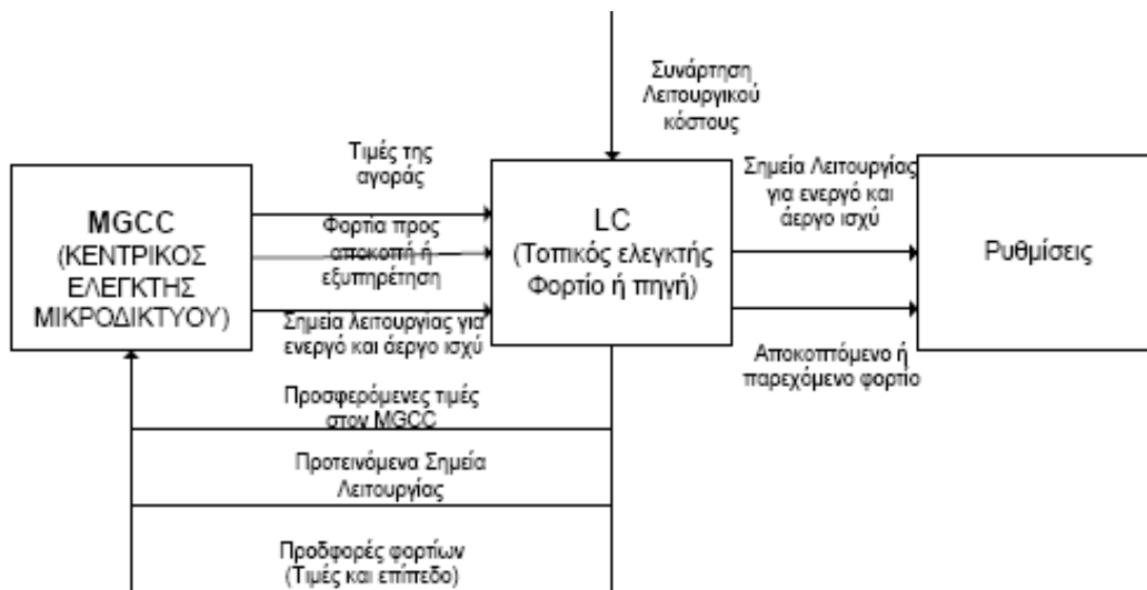
Εικόνα Γ.2.4. Η ροή πληροφορίας μεταξύ του κεντρικού ελέγκτη και των τοπικών ελεγκτών σε ένα μικροδίκτυο.
