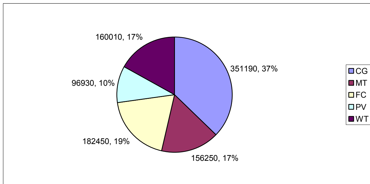
Εικόνα ΣΤ.4. 172. Κάλυψη του ηλεκτρικού φορτίου. Σεναριο DSB, DG=148kW, Χαμηλή ΟΤΣ.
