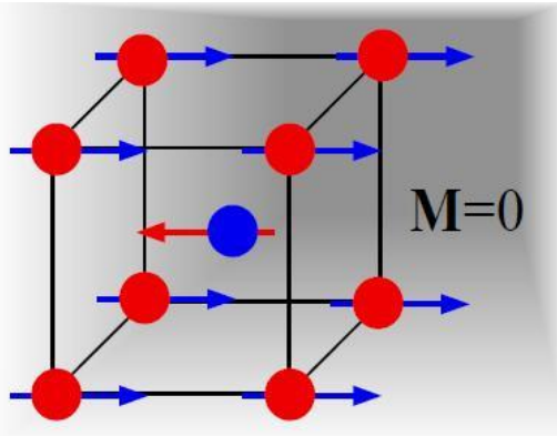
Σχήμα 8: Οι μαγνητικές ροπές σε αντισιδηρομαγνήτες (https://eclass.uowm.gr/modules/document/)
