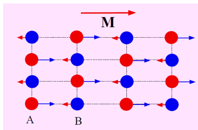
Σχήμα 9: Οι μαγνητικές ροπές σε σιδηριμαγνήτες (https://eclass.uowm.gr/modules/document/)
