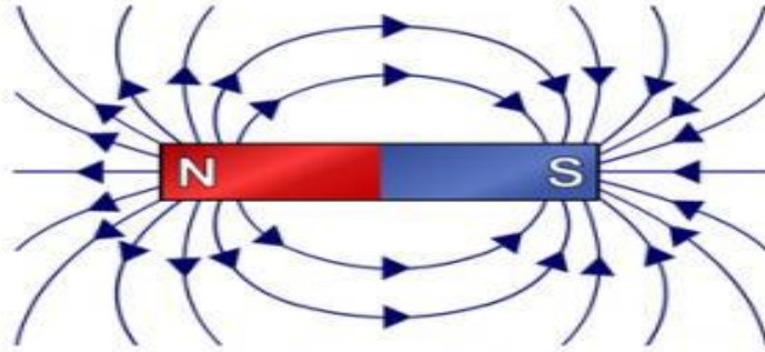
Σχήμα 2: Μαγνητικές γραμμές διανυσματικά στο χώρο, που αναπτύσσονται με βάση την ένταση και την κατεύθυνση του μαγνητικού πεδίου ( https://brilliant.org/wiki/magnetic-field-lines/ )
