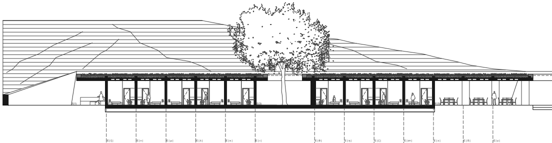
0 1 2 3 4 5 10 15 20 25 ΚΑΙΜΑΚΑ 1:200 ΤΙΤΛΟΣ ΣΧΕΔΙΟΥ :ΤΟΜΗ Θ-Θ' | ΔΥΤΙΚΗ ΟΨΗ E (1) ΗΜΙΥΠΑΙΘΡΙΑ ΚΑΤΟΙΚΙΕΣ E (2) ΚΑΤΟΙΚΙΕΣ
