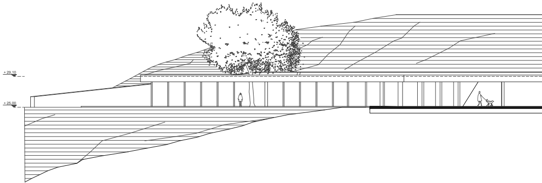
0 1 2 3 4 5 10 15 20 25 ΚΑΙΜΑΚΑ 1:200 ΤΙΤΛΟΣ ΣΧΕΔΙΟΥ :ΤΟΜΗ Η-Η' | ΒΟΡΕΙΟΔΥΤΙΚΗ ΟΨΗ Δ (1) Δ (2)
