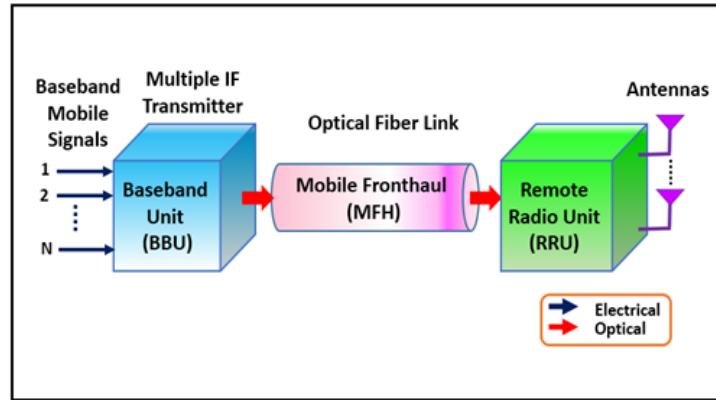
Σχήμα 5: Σχηματικό διάγραμμα κινητού fronthaul ενός οπτικού καναλιού.
