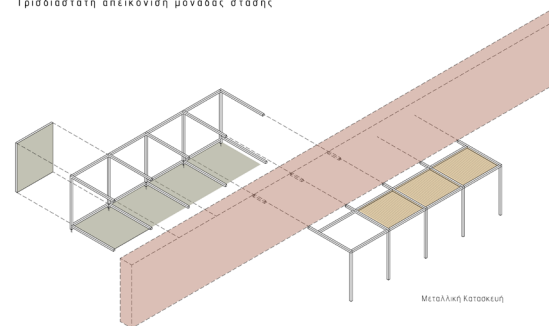
Αξονομετρικό Μονάδας Στάσης ΚΑ 1/100
