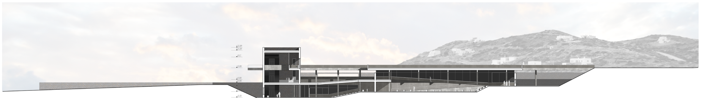
ΤΟΜΗ Α-Α ΚΑ 1/200 0 5 10 20m
