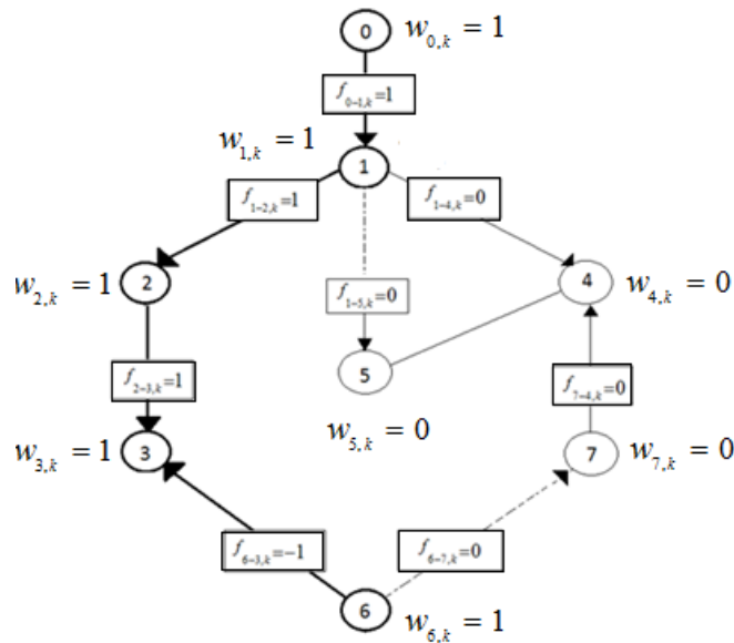
Σχήμα 3.3 : Σχέση μεταξύ των μεταβλητών y_{ij} , f_{ij,k} και zact_{z(i),k}
