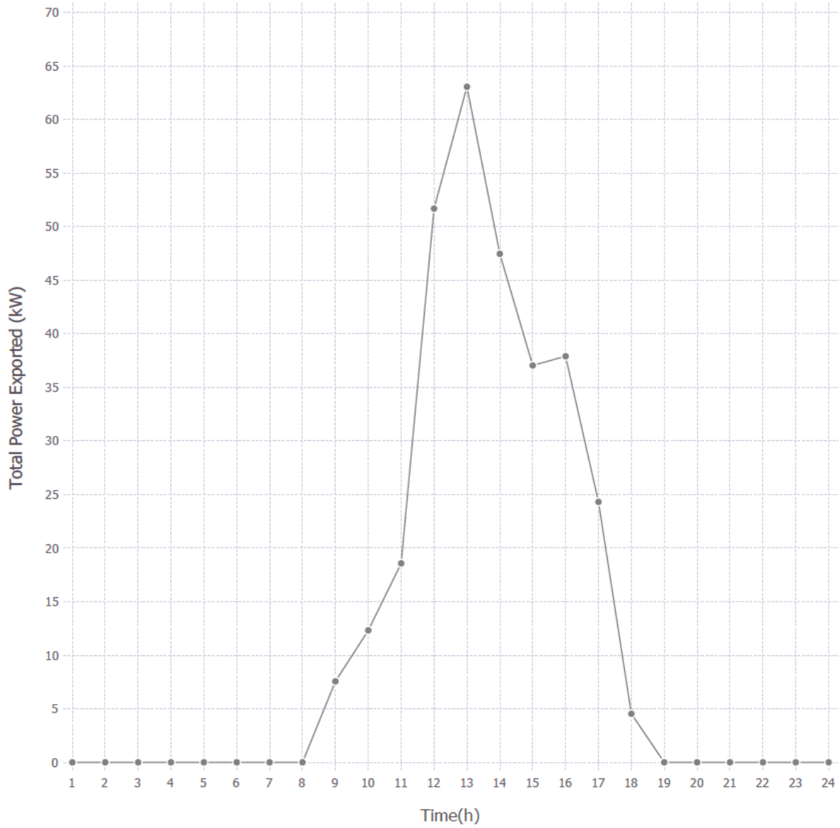
Σχήμα 24. Συνολική Ωριαία Εξαγόμενη Ισχύς από την Κοινότητα
