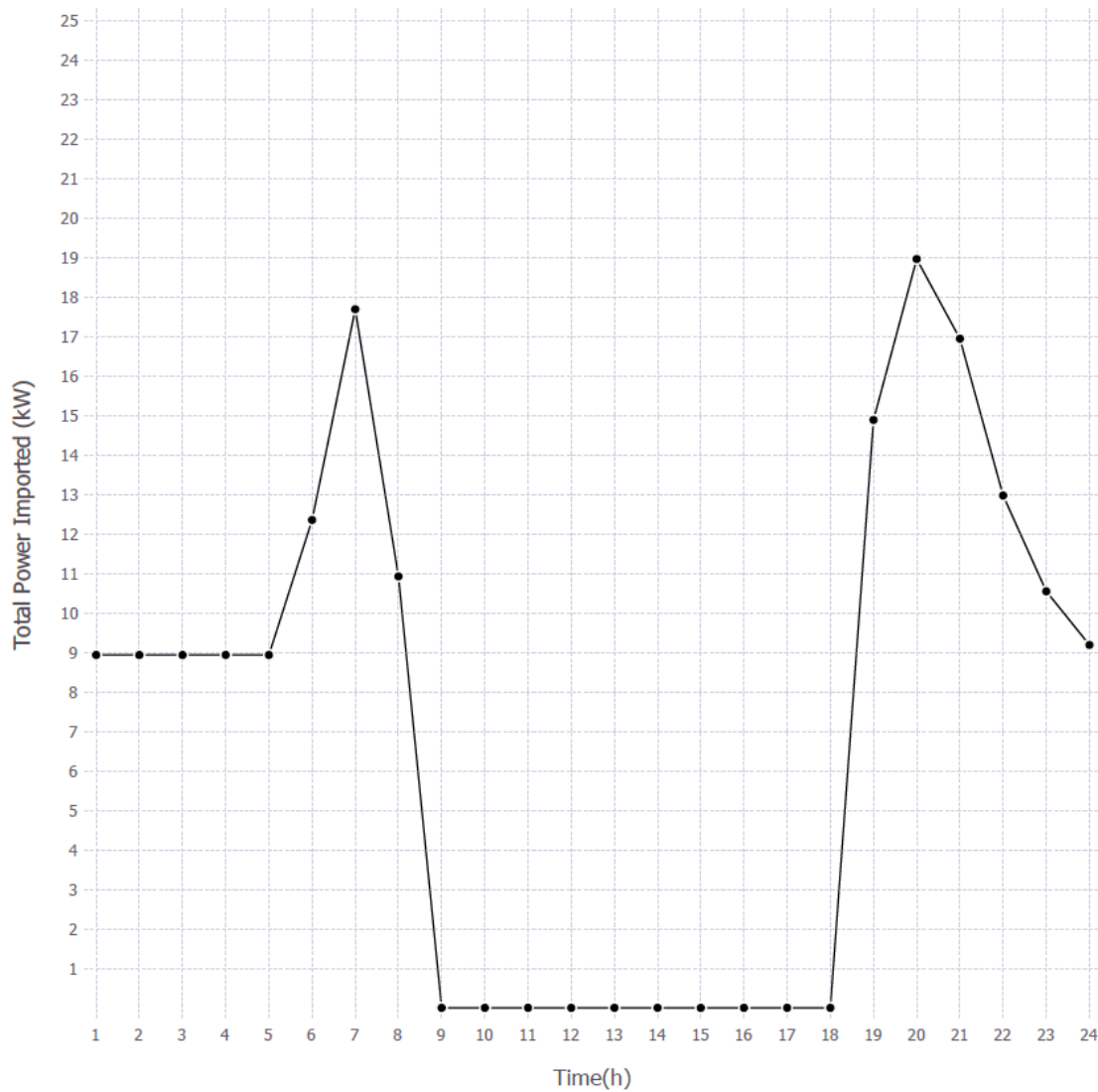
Σχήμα 23. Συνολική Ωριαία Εισαγόμενη ισχύς στη Κοινότητα την αντιπροσωπευτική ημέρα του Απριλίου
