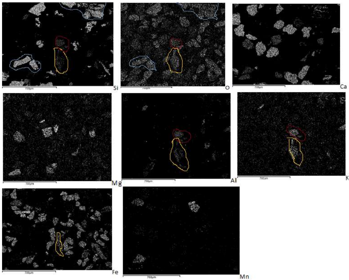
Εικόνα 3.15: Φωτογραφία Ηλεκτρονικού Μικροσκοπίου Σάρωσης από το πρώτο δείγμα που λήφθηκε από την παραλία του Θορικού. Από τις πιο πάνω εικόνες ελέγχθηκε η παρουσία χαλαζία και διάφορων πυριτικών ορυκτών. Με γαλάζιο χρώμα σημειώθηκε η παρουσία χαλαζία και με κίτρινο και κόκκινο τα πυριτικά ορυκτά που βρέθηκαν.
