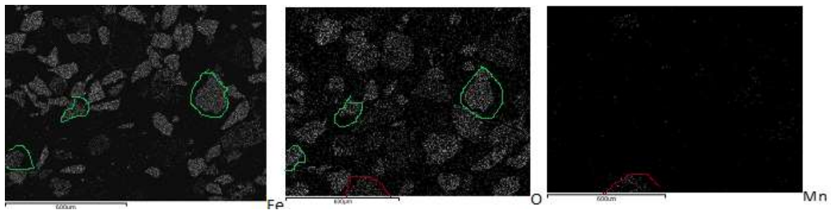
Εικόνα 3.24: Φωτογραφία Ηλεκτρονικού Μικροσκοπίου Σάρωσης από το δεύτερο δείγμα που λήφθηκε από την παραλία του Θορικού. Από τις πιο πάνω εικόνες ελέγχθηκε η παρουσία οξειδίων του σιδήρου και οξειδίων του μαγγανίου. Με πράσινο χρώμα σημειώθηκε η παρουσία οξειδίων του σιδήρου (αιματίτης, γκαϊτίτης, υδροξείλιο), ενώ με κόκκινο η παρουσία οξειδίων του μαγγανίου (πυρολουσίτη, μαγγανίτη).
