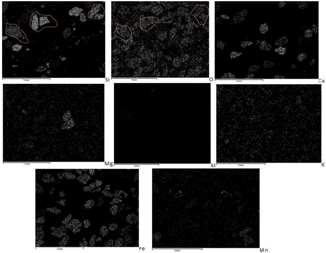
Εικόνα 3.11: Φωτογραφία Ηλεκτρονικού Μικροσκοπίου Σάρωσης από το τρίτο δείγμα που λήφθηκε από την παραλία του Οξυγόνου. Από τις πιο πάνω εικόνες ελέγχθηκε η παρουσία χαλαζία και διάφορων πυριτικών ορυκτών. Με καφέ χρώμα σημειώθηκε η παρουσία χαλαζία. Δεν παρατηρήθηκε κάποιο άλλο πυριτικό ορυκτό.
