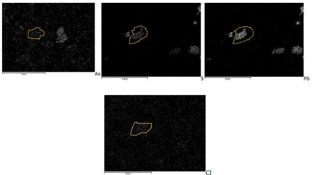
Εικόνα 3.10: Φωτογραφία Ηλεκτρονικού Μικροσκοπίου Σάρωσης από το τρίτο δείγμα που λήφθηκε από την παραλία του Οξυγόνου. Στα κυκλωμένα σημεία έχουμε συνύπαρξη Μολύβδου (Pb), Θείου (S) και Αρσενικού (As) που σημαίνει ότι έχουμε ύπαρξη Μιμετίτη ( Pb_5(As_5O_4)_3Cl )
