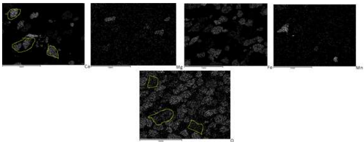
Εικόνα 3.8: Φωτογραφία Ηλεκτρονικού Μικροσκοπίου Σάρωσης από το δεύτερο δείγμα που λήφθηκε από την παραλία του Οξυγόνου. Από τις πιο πάνω εικόνες ελέγχθηκε η παρουσία ανθρακικών ορυκτών. Με πράσινο χρώμα σημειώθηκε η παρουσία ασβεστίτη.
