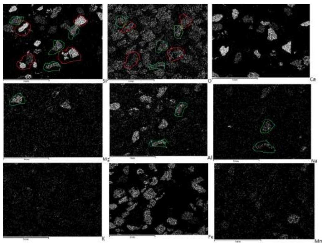
Εικόνα 3.2: Φωτογραφία Ηλεκτρονικού Μικροσκοπίου Σάρωσης από το πρώτο δείγμα που λήφθηκε από την παραλία του Οξυγόνου. Από τις πιο πάνω εικόνες ελέγχθηκε η παρουσία χαλαζία και διάφορων πυριτικών ορυκτών. Με κόκκινο χρώμα σημειώθηκε η παρουσία χαλαζία και με πράσινο τα πυριτικά ορυκτά.
