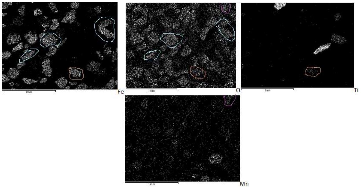
Εικόνα 3.3: Φωτογραφία Ηλεκτρονικού Μικροσκοπίου Σάρωσης από το πρώτο δείγμα που λήφθηκε από την παραλία του Οξυγόνου. Από τις πιο πάνω εικόνες ελέγχθηκε η παρουσία οξειδίων του σιδήρου και οξειδίων του μαγγανίου. Με γαλάζιο χρώμα σημειώθηκε η παρουσία οξειδίων του σιδήρου (αιματίτης, γκαϊτίτης, υδροξείλιο), με καφέ χρώμα η παρουσία τιτανίου μαγνητίτη, ενώ με μωβ χρώμα η παρουσία οξειδίων του μαγγανίου (πυρολουσίτης).
