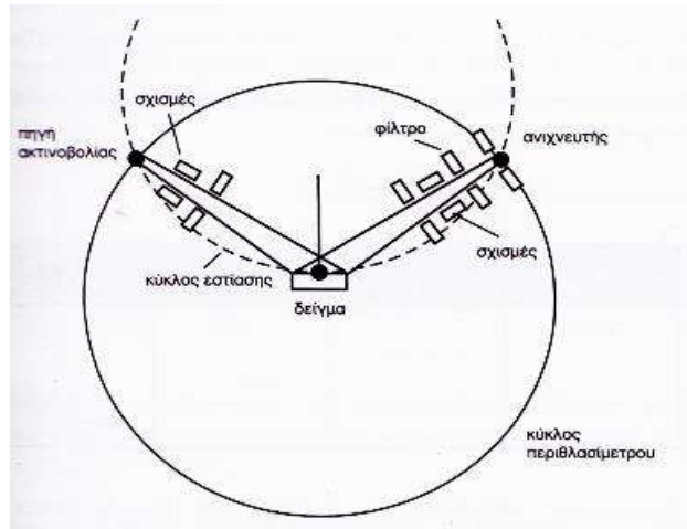
Εικόνα 2.7: Σχηματική απεικόνιση περιθλασιόμετρου Ακτινών X, (Λιοδάκης, 2001)
