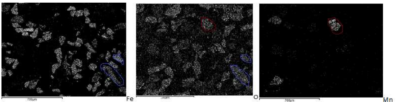
Εικόνα 3.16: Φωτογραφία Ηλεκτρονικού Μικροσκοπίου Σάρωσης από το πρώτο δείγμα που λήφθηκε από την παραλία του Θορικού. Από τις πιο πάνω εικόνες ελέγχθηκε η παρουσία οξειδίων του σιδήρου και οξειδίων του μαγγανίου. Με μπλε χρώμα σημειώθηκε η παρουσία οξειδίων του σιδήρου (αιματίτης, γκαιτίτης, υδροξείλιο). Με κόκκινο σημειώθηκε η παρουσία οξειδίων του μαγγανίου.
