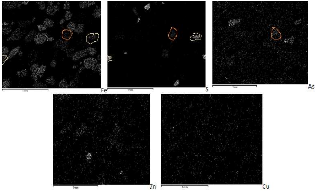
Εικόνα 3.5: Φωτογραφία Ηλεκτρονικού Μικροσκοπίου Σάρωσης από το δεύτερο δείγμα που λήφθηκε από την παραλία του Οξυγόνου. Από τις πιο πάνω εικόνες ελέγχθηκε η παρουσία θειούχων μεταλλευμάτων. Με το λευκό χρώμα σημειώθηκε η παρουσία σιδηροπυρίτη, ενώ με το πορτοκαλί η παρουσία αρσενοπυρίτη.
