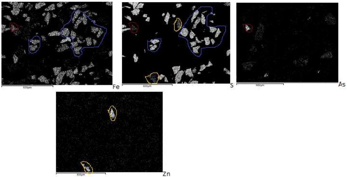
Εικόνα 3.17: Φωτογραφία Ηλεκτρονικού Μικροσκοπίου Σάρωσης από το πρώτο δείγμα που λήφθηκε από την παραλία του Θορικού. Από τις πιο πάνω εικόνες ελέγχθηκε η παρουσία ανθρακικών ορυκτών. Με πορτοκαλί σημειώθηκε η παρουσία ασβεστίτη, ενώ με κόκκινο η παρουσία λοιπών ανθρακικών ορυκτών (πιθανώς ανκερίτη).
