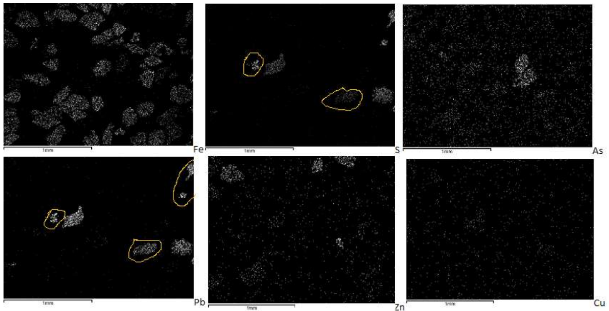
Εικόνα 3.9: Φωτογραφία Ηλεκτρονικού Μικροσκοπίου Σάρωσης από το τρίτο δείγμα που λήφθηκε από την παραλία του Οξυγόνου. Από τις πιο πάνω εικόνες ελέγχθηκε η παρουσία θειούχων μεταλλευμάτων. Παρατηρήθηκε η ύπαρξη γαληνίτη, που σημειώθηκε με κίτρινο χρώμα.
