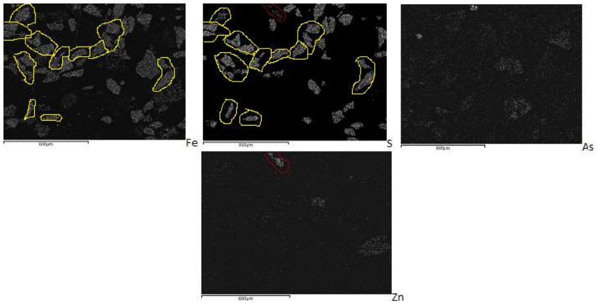
Εικόνα 3.22: Φωτογραφία Ηλεκτρονικού Μικροσκοπίου Σάρωσης από το τρίτο δείγμα που λήφθηκε από την παραλία του Θορικού. Από τις πιο πάνω εικόνες ελέγχθηκε η παρουσία θειούχων μεταλλευμάτων. Παρατηρήθηκε η ύπαρξη σφαλερίτη, που σημειώθηκε με κόκκινο χρώμα. Η παρουσία σιδηροπυρίτη είναι σημειωμένη με κίτρινο.
