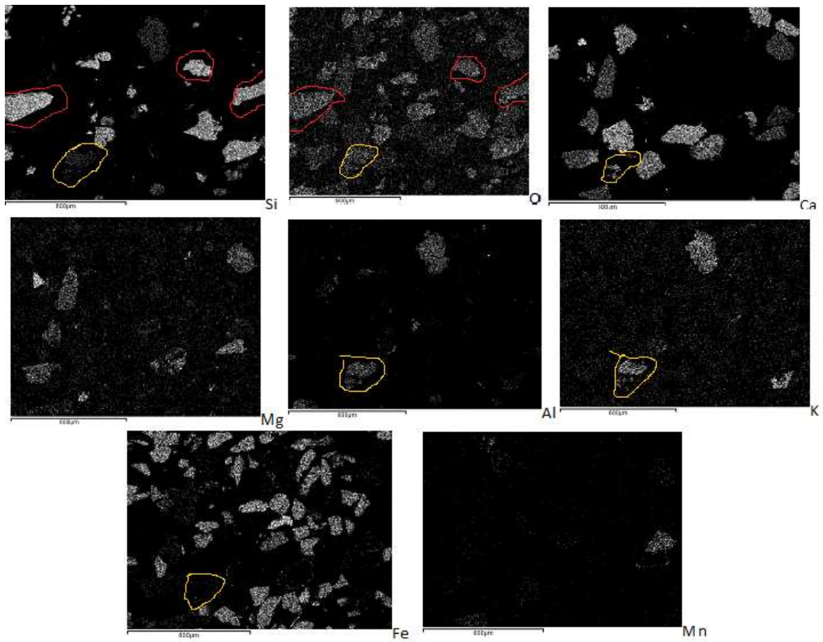
Εικόνα 3.19: Φωτογραφία Ηλεκτρονικού Μικροσκοπίου Σάρωσης από το δεύτερο δείγμα που λήφθηκε από την παραλία του Θορικού. Από τις πιο πάνω εικόνες ελέγχθηκε η παρουσία χαλαζία και διάφορων πυριτικών ορυκτών. Με κόκκινο χρώμα σημειώθηκε η παρουσία χαλαζία και με κίτρινο τα πυριτικά ορυκτά που βρέθηκαν
