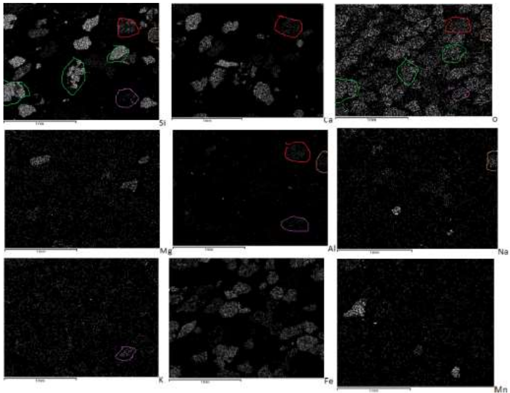
Εικόνα 3.6: Φωτογραφία Ηλεκτρονικού Μικροσκοπίου Σάρωσης από το δεύτερο δείγμα που λήφθηκε από την παραλία του Οξυγόνου. Από τις πιο πάνω εικόνες ελέγχθηκε η παρουσία χαλαζία και διάφορων πυριτικών ορυκτών. Με πράσινο χρώμα σημειώθηκε η παρουσία χαλαζία, ενώ με κόκκινο, καφέ και μωβ σημειώθηκαν η παρουσία διάφορων πυριτικών ορυκτών.
