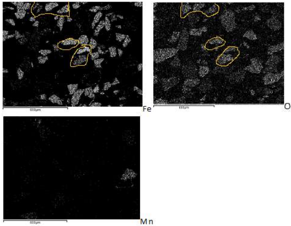
Εικόνα 3.20: Φωτογραφία Ηλεκτρονικού Μικροσκοπίου Σάρωσης από το δεύτερο δείγμα που λήφθηκε από την παραλία του Θορικού. Από τις πιο πάνω εικόνες ελέγχθηκε η παρουσία οξειδίων του σιδήρου και οξειδίων του μαγγανίου. Με κίτρινο χρώμα σημειώθηκε η παρουσία οξειδίων του σιδήρου (αματίτης, γκαϊτίτης, υδροξείλιο).
