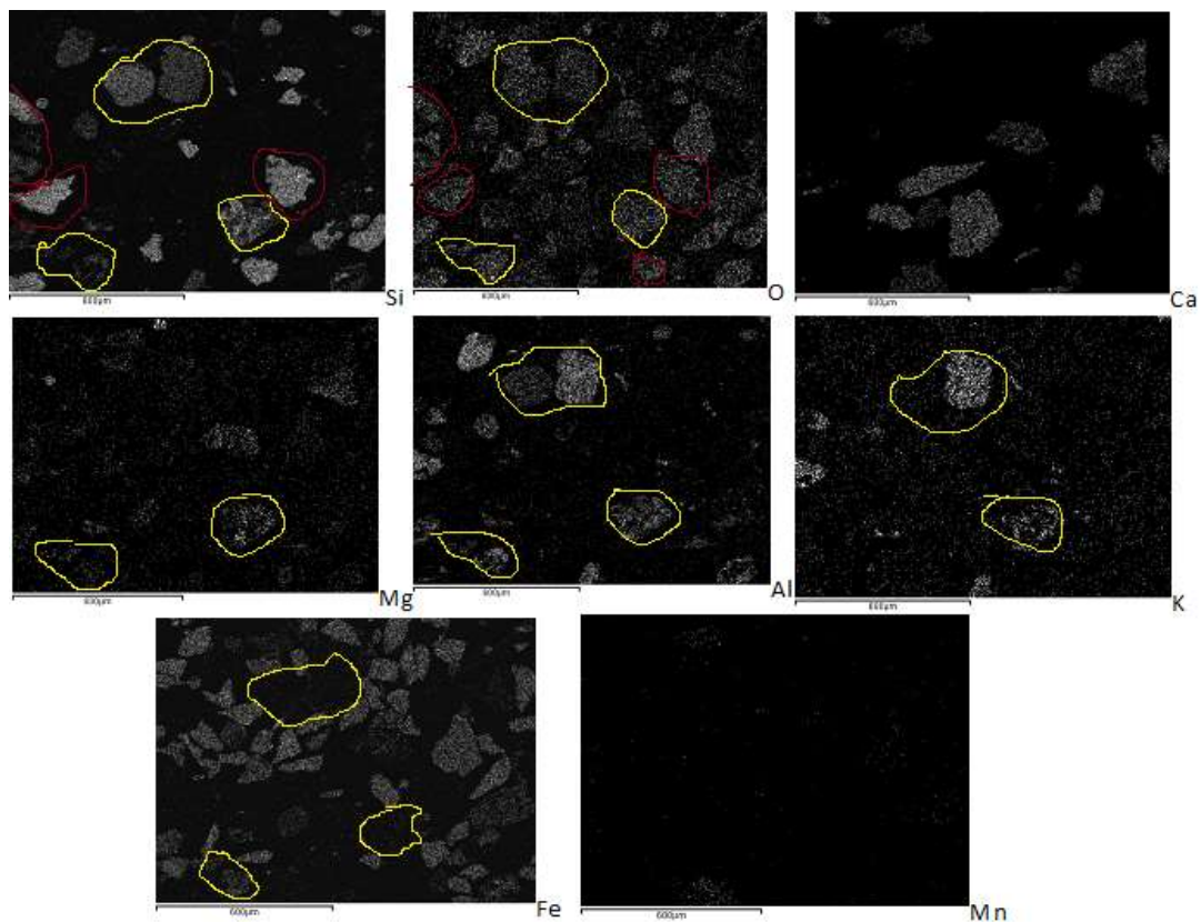
Εικόνα 3.22: Φωτογραφία Ηλεκτρονικού Μικροσκοπίου Σάρωσης από το τρίτο δείγμα που λήφθηκε από την παραλία του Θορικού. Από τις πιο πάνω εικόνες ελέγχθηκε η παρουσία θειούχων μεταλλευμάτων. Παρατηρήθηκε η ύπαρξη σφαλερίτη, που σημειώθηκε με κόκκινο χρώμα. Η παρουσία σιδηροπυρίτη είναι σημειωμένη με κίτρινο.
