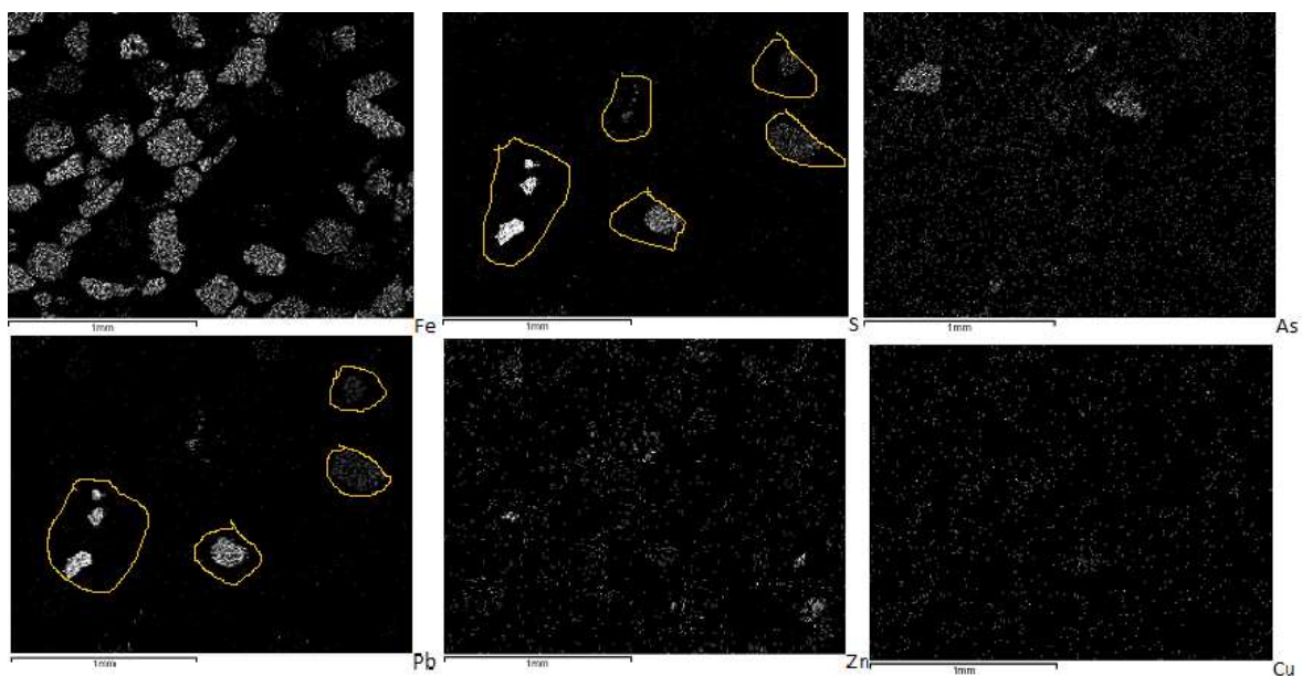
Εικόνα 3.1: Φωτογραφία Ηλεκτρονικού Μικροσκοπίου Σάρωσης από το πρώτο δείγμα που λήφθηκε από την παραλία του Οξυγόνου. Από τις πιο πάνω εικόνες ελέγχθηκε η παρουσία θειούχων μεταλλευμάτων. Παρατηρήθηκε η ύπαρξη γαληνίτη, που σημειώθηκε με κίτρινο χρώμα.
