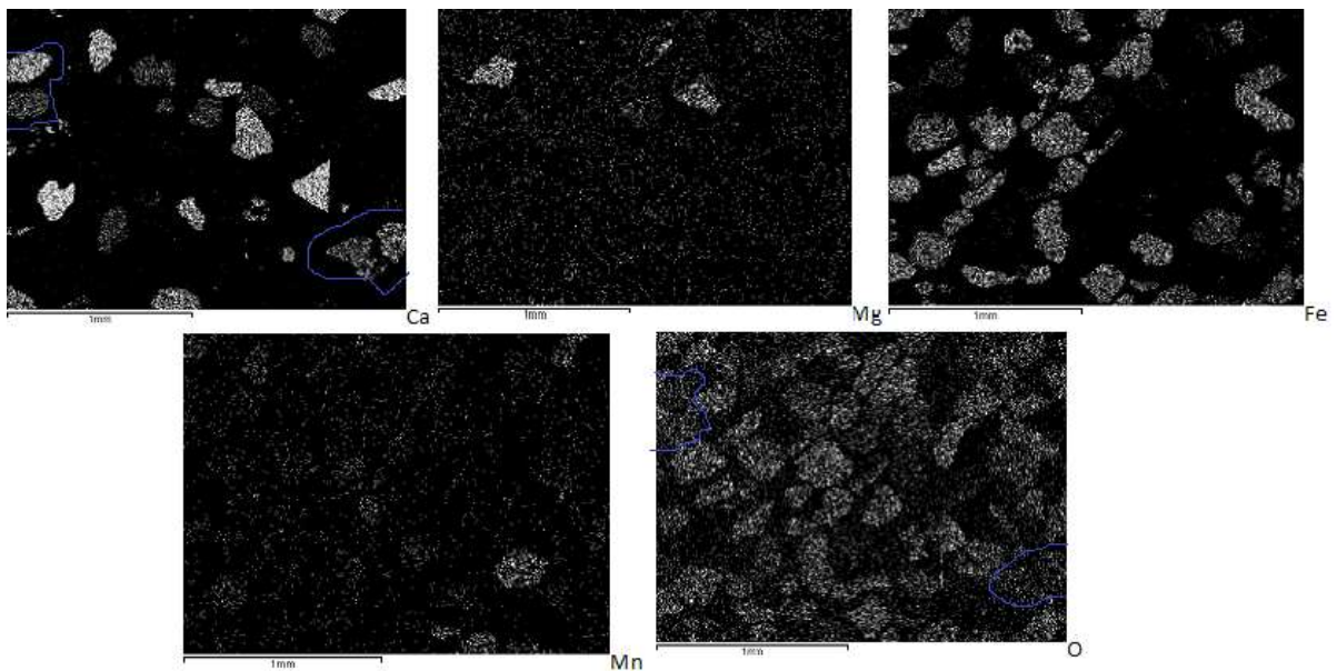
Εικόνα 3.4: Φωτογραφία Ηλεκτρονικού Μικροσκοπίου Σάρωσης από το πρώτο δείγμα που λήφθηκε από την παραλία του Οξυγόνου. Από τις πιο πάνω εικόνες ελέγχθηκε η παρουσία ανθρακικών ορυκτών. Με μπλε χρώμα σημειώθηκε η παρουσία ασβεστίτη.
