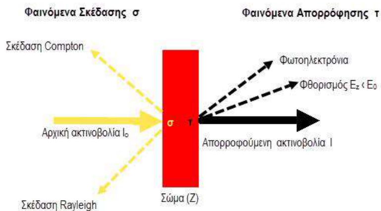
Εικόνα 2.11: Αλληλεπίδραση ακτίνων X με την ύλη (Κουή κ.α., 2015)
