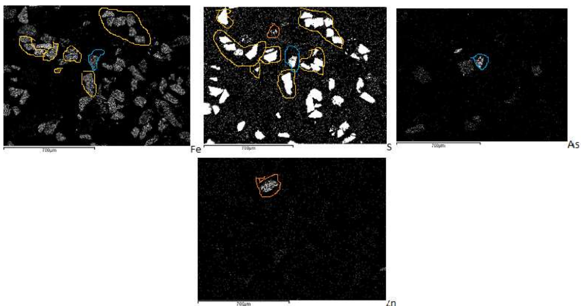
Εικόνα 3.14: Φωτογραφία Ηλεκτρονικού Μικροσκοπίου Σάρωσης από το πρώτο δείγμα που λήφθηκε από την παραλία του Θορικού. Από τις πιο πάνω εικόνες ελέγχθηκε η παρουσία θειούχων μεταλλευμάτων. Παρατηρήθηκε η ύπαρξη σφαλερίτη, που σημειώθηκε με πορτοκαλί χρώμα. Με κίτρινο σημειώθηκε ο σιδηροπυρίτης, ενώ με μπλε ο αρσενοπυρίτης.
