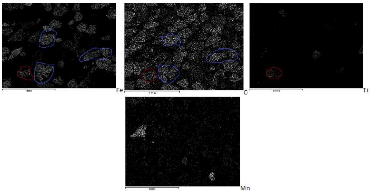
Εικόνα 3.7: Φωτογραφία Ηλεκτρονικού Μικροσκοπίου Σάρωσης από το δεύτερο δείγμα που λήφθηκε από την παραλία του Οξυγόνου. Από τις πιο πάνω εικόνες ελέγχθηκε η παρουσία οξειδίων του σιδήρου και οξειδίων του μαγγανίου. Με μπλε χρώμα σημειώθηκε η παρουσία οξειδίων του σιδήρου (αιματίτης, γκαιτίτης, υδροξείλιο), με κόκκινο χρώμα η παρουσία τιτανιούχου μαγνητίτη.
