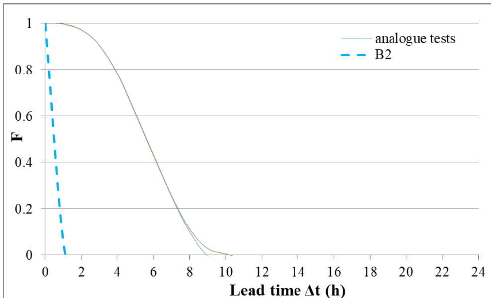
Σχήμα 10. Ανάλυση ευαισθησίας αναλογικού μοντέλου και B2 ( g_{average}=0.5 ) χρονοσειράς ηλιακής ακτινοβολίας στην Αστυπάλαια.
