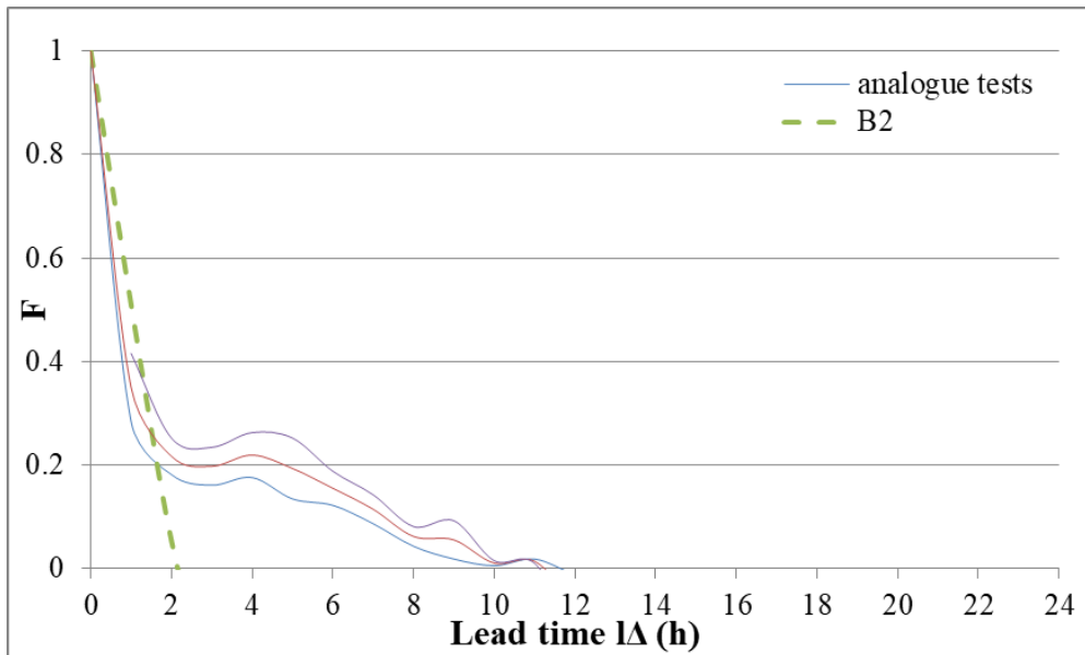
Σχήμα 9. Ανάλυση ευαισθησίας αναλογικού μοντέλου και B2 ( g_{average}=0.5 ) χρονοσειράς ανέμου στην Αστυπάλαια.
