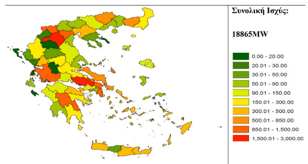
Εικόνα 10 : Συνολική Εγκατεστημένη Ισχύς Σταθμών Ηλεκτροπαραγωγής (πηγή: Ενέργεια και Τοπικές Κοινωνίες, Ιωάννα Τσίγκανου, Ρόη Κίντη)
