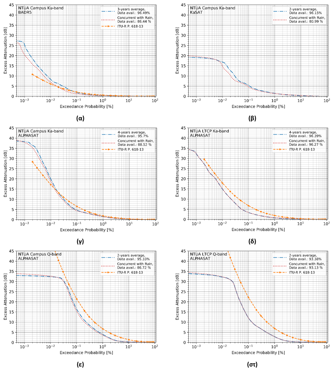
Σχήμα 1-8: Κατανομές υπέρβασης εξασθένησης ως ποσοστό του χρόνου για όλες τις συχνότητες και στις δύο περιοχές (α) Ku-band BADR5 Campus, (β) Ka-band KaSAT Campus, (γ) Ka-band ALPHASAT Campus, (δ) Ka-band ALPHASAT LTCP, (ε) Q-band ALPHASAT Campus, (στ) Q-band ALPHASAT LTCP
