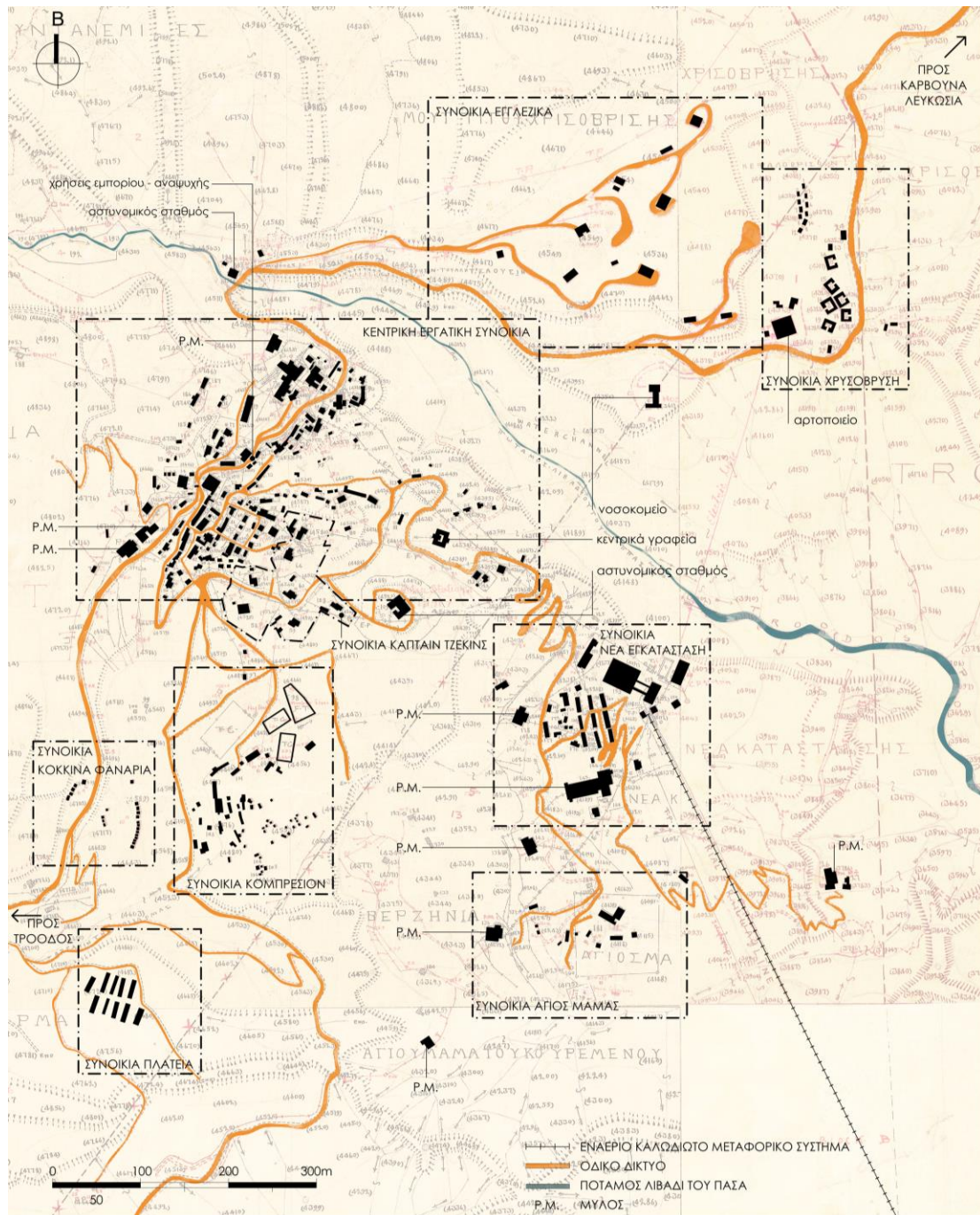
Εικ. 2.58.* Τοπογραφικό σχέδιο των συνοικιών του Αμιάντου την περίοδο του Μεσοπολέμου (υπόβαθρο: Τμ. Κτηματολογίου και Χωρομετρίας, αποσπάσματα τοπογραφικών σχεδίων 3753, 3754, 3761, 3762, original, κλ. 1:5000, 1920-1927).
