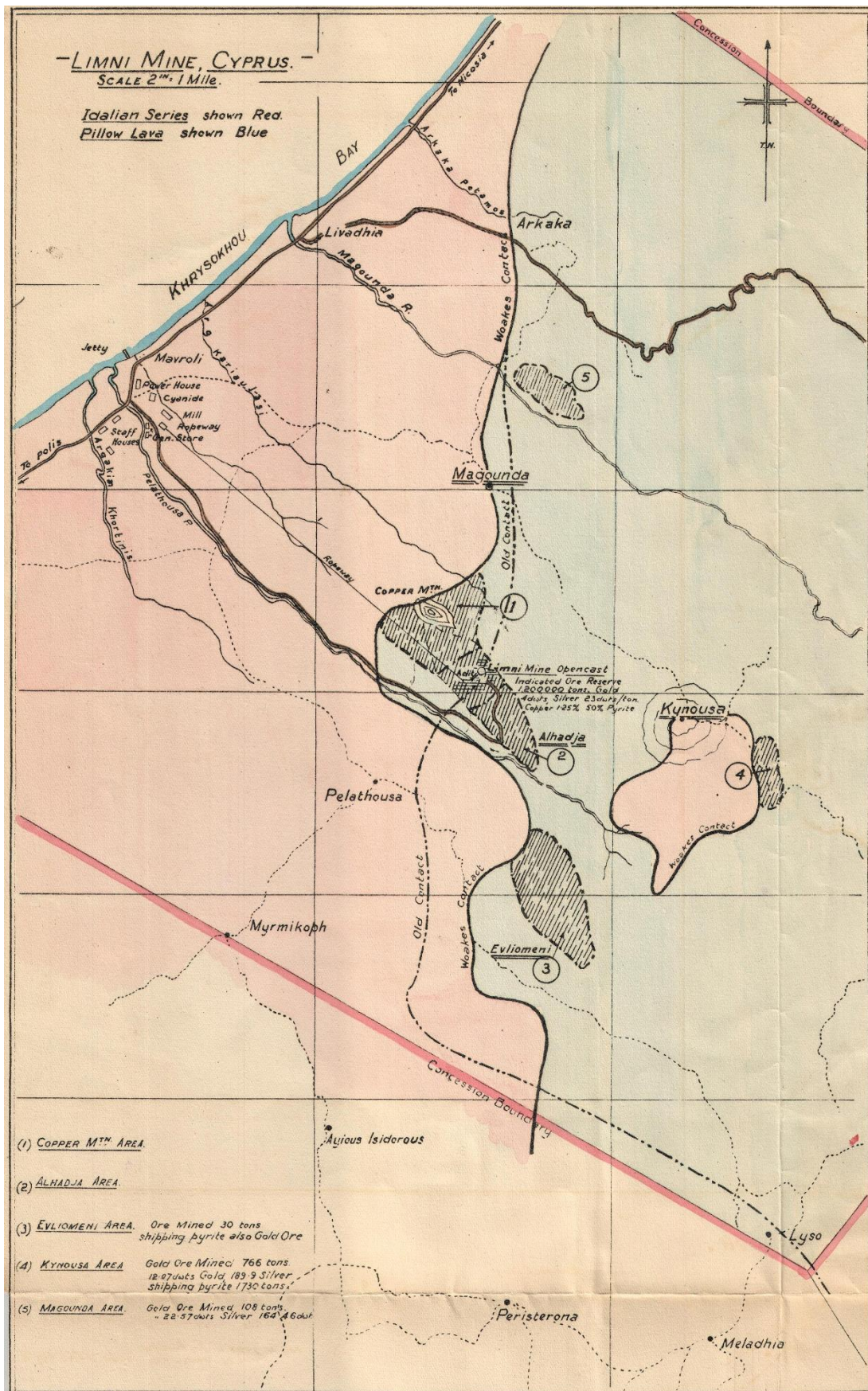
Εικ. 3.23. Τα κοιτάσματα και οι κύριες εγκαταστάσεις της Λίμνης, όπως αποτυπώθηκαν σε χάρτη του 1946 (Τμ. Μεταλλείων, Μ.509.С).
