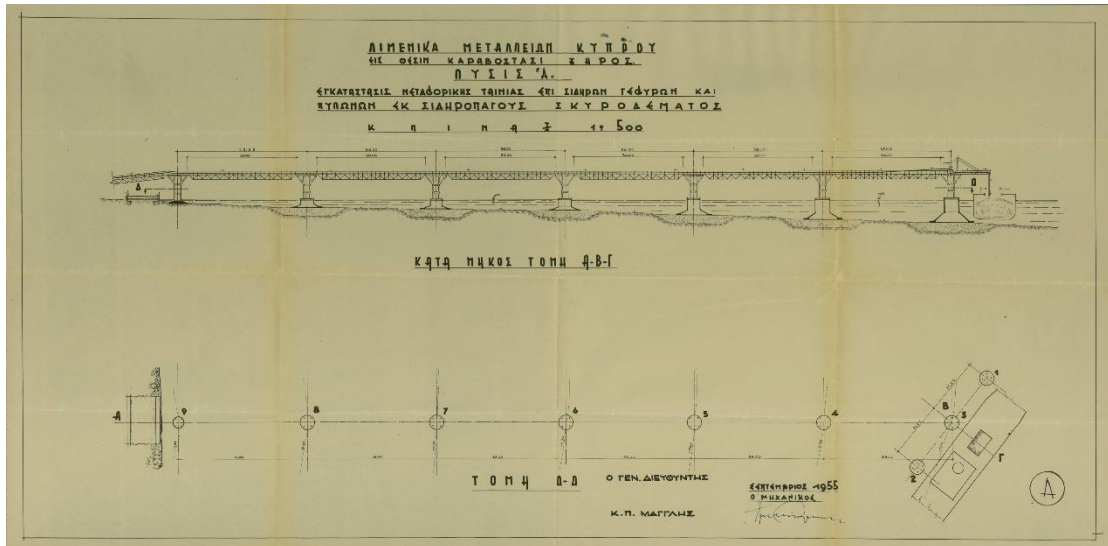
Εικ. 4.8. Σχέδια της αποβάθρας φόρτωσης στο Καραβοστάσι, 1955 (Κρατικό Αρχείο, SA1 1213/1956).
