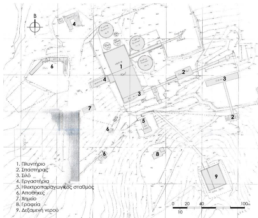
Εικ. 4.3.* Τοπογραφικό διάγραμμα των εγκαταστάσεων του εργοστασίου θραύσης και εμπλουτισμού των μεταλλευμάτων στο Μιτσερό (αρχείο ΕΜΕ).
