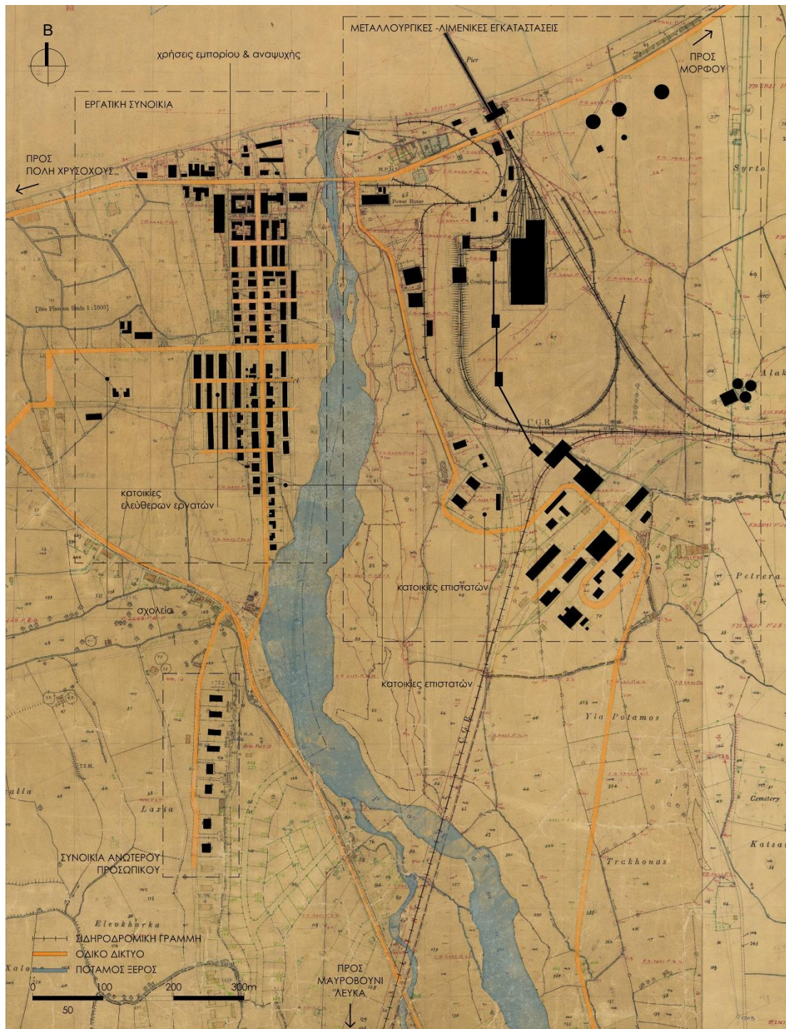
Εικ. 2.61.* Τοπογραφικό σχέδιο του οικισμού του Ξερού (υπόβαθρο: Τμ. Κτηματολογίου και Χωρομετρίας, αποσπάσματα τοπογραφικών σχεδίων 1958Ε2, 1959W2, 2802Ε1, 2803W1, original, κλ. 1:2.500, 1928-1931).
