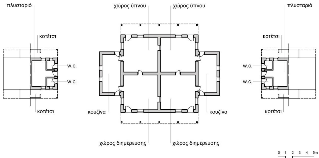
Εικ. 4.21. Κάτοψη του τυπικού κτηρίου των τεσσάρων κατοικιών και των βοηθητικών του κτηρίων του οικισμού των Πλατειών της ΕΜΕ μετά το μετασχηματισμό του σε κτήριο δυο κατοικιών (σχέδιο από τον συγγραφέα).
