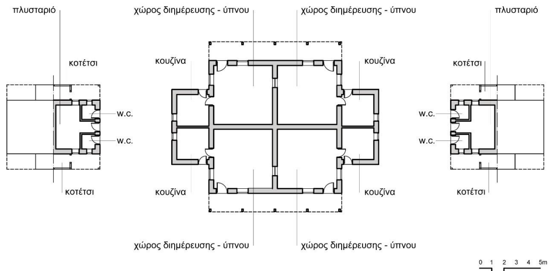
Εικ. 4.20. Κάτοψη του τυπικού κτηρίου των τεσσάρων κατοικιών και των βοηθητικών κτηρίων τουαλετών, πλυσταριών και κοτετσιών του οικισμού των Πλατειών της ΕΜΕ (σχέδιο από τον συγγραφέα).
