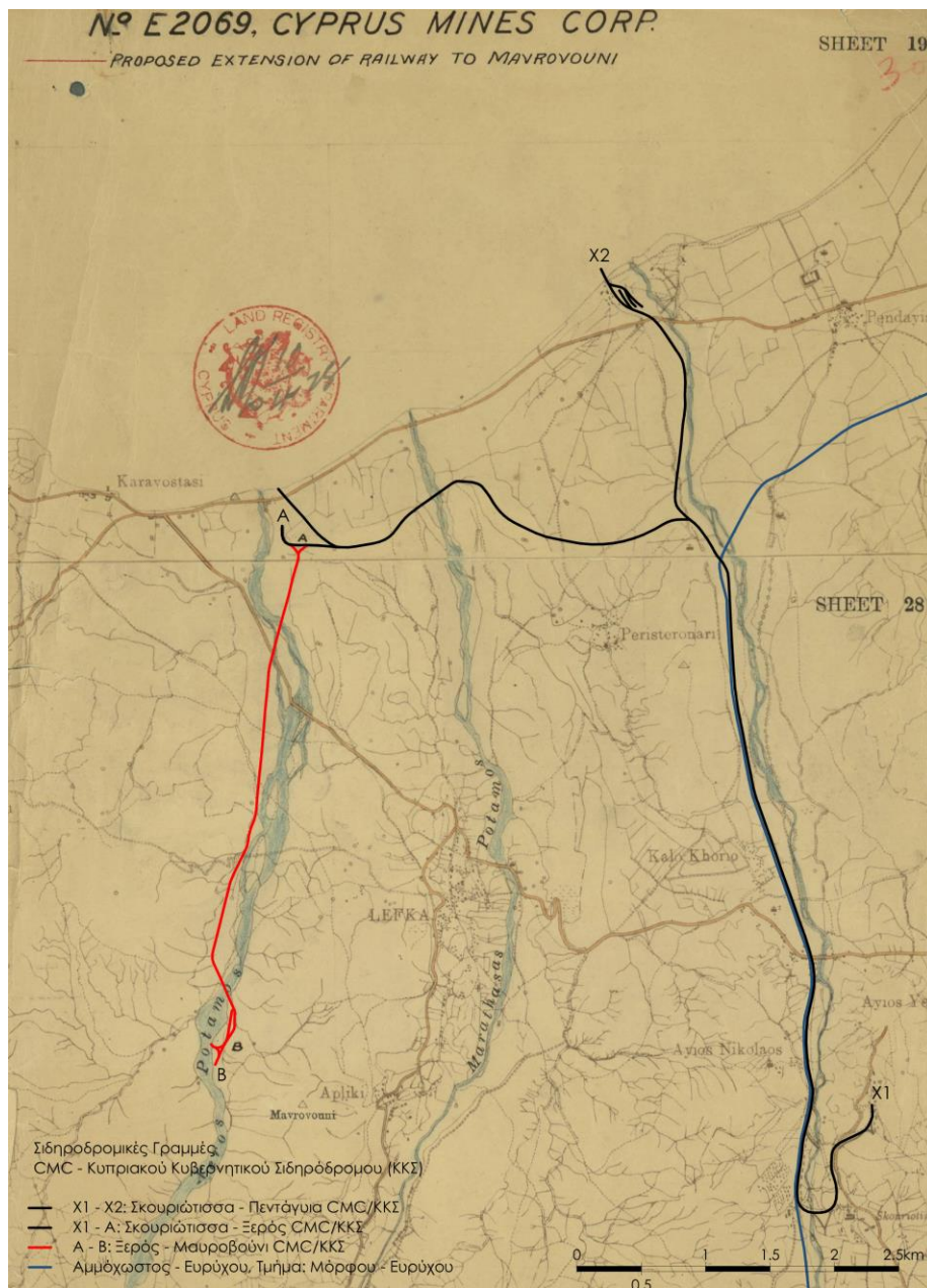
Εικ. 2.18.* Το σιδηροδρομικό δίκτυο της CMC σε τοπογραφικό σχέδιο της προτεινόμενης επέκτασής του δικτύου της εταιρείας από τον Ξερό στο Μαυροβούνι, 1928 (Κρατικό Αρχείο, CW/2817).
