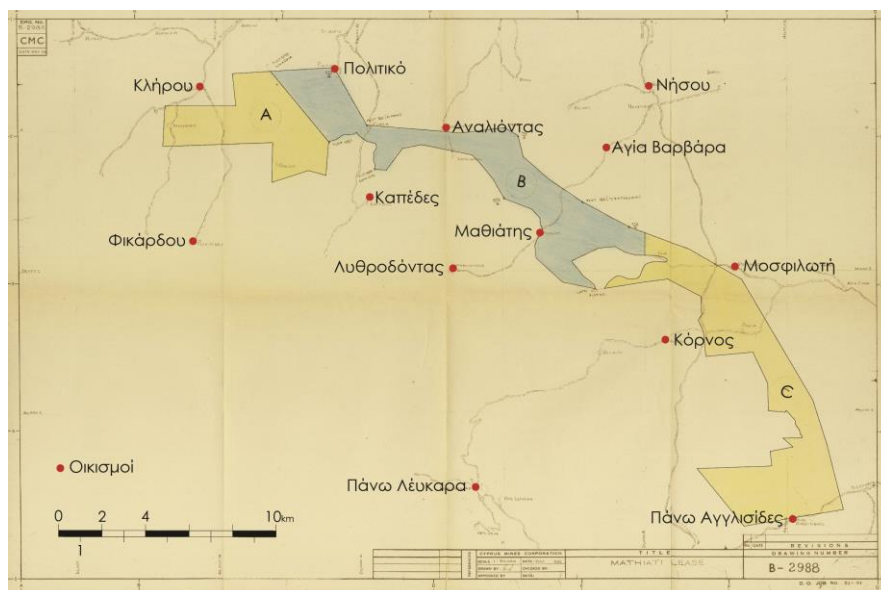
Εικ. 2.13.* Τοπογραφικό διάγραμμα της μεταλλευτικής μισθώσης Μαθιάτη της CMC, 1956 (Κρατικό Αρχείο, SA1 1157/1949/2).
