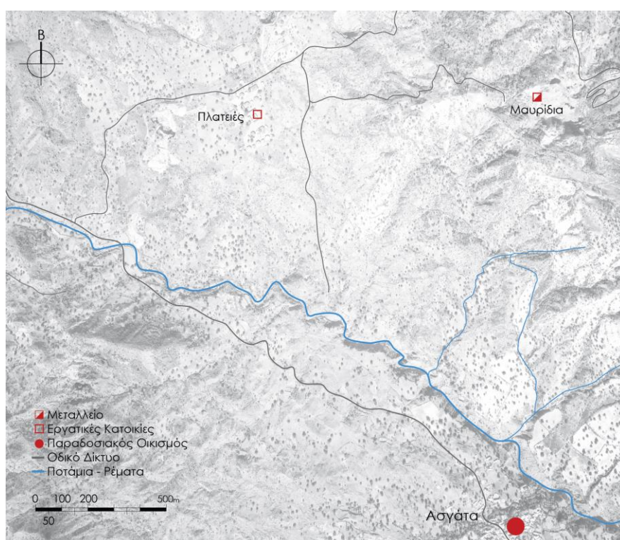
Εικ. 2.32.* Οι μεσοπολεμικές εγκαταστάσεις της ΑΕΕΧΠΛ στη μεταλλευτική μίσθωση Ασγάτας – Καλαβασού (υπόβαθρο: Τμ. Κτηματολογίου και Χωρομετρίας, απόσπασμα αεροφωτογραφίας, 1963).
