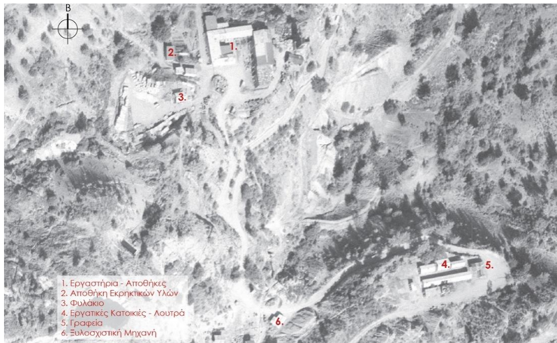
Εικ. 2.33.* Οι μεσοπολεμικές εγκαταστάσεις της ΑΕΕΧΠΛ στα Μαυρίδια (υπόβαθρο: Τμ. Κτηματολογίου και Χωρομετρίας, απόσπασμα αεροφωτογραφίας, 1963).
