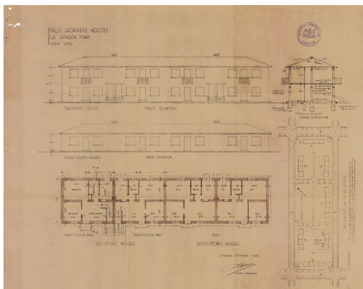
Εικ. 4.52. Σχέδια των προτεινόμενων εργατικών κατοικιών του Δήμου Λεμεσού, 1945 (Αρχείο Δήμου Λεμεσού, ΔΛ1/66).
