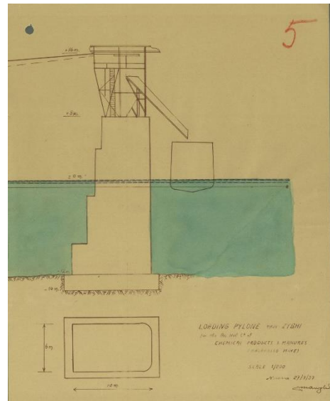
Εικ. 2.50. Σχέδιο του πυλώνα φόρτωσης των μεταλλευμάτων στα πλοία του εναέριου καλωδιωτού μεταφορικού συστήματος της ΑΕΕΧΠΛ στην περιοχή του Βασιλικού, 1937 (Κρατικό Αρχείο, SA1 1137/1937).
