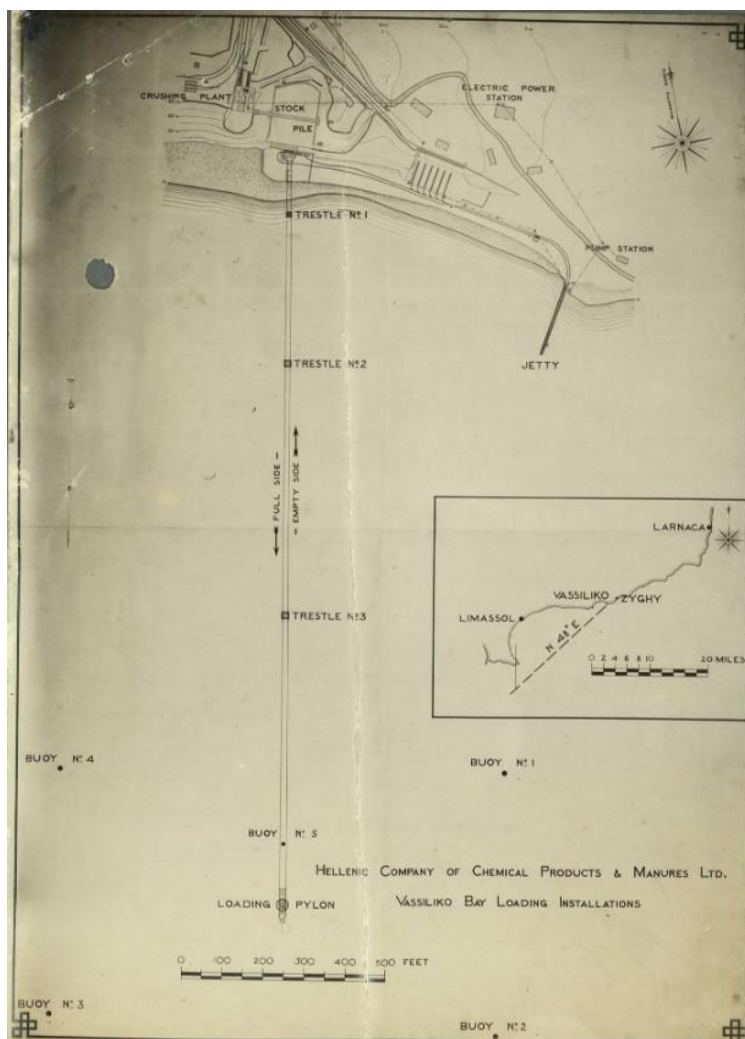
Εικ. 2.34. Σχέδιο των παραγωγικών και λιμενικών εγκαταστάσεων του Βασιλικού, 1946 (Κρατικό Αρχείο, SA1 1091/1937/3).
