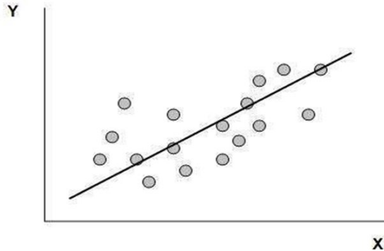
Διάγραμμα 3.1: Ευθεία ελαχίστων τετραγώνων
