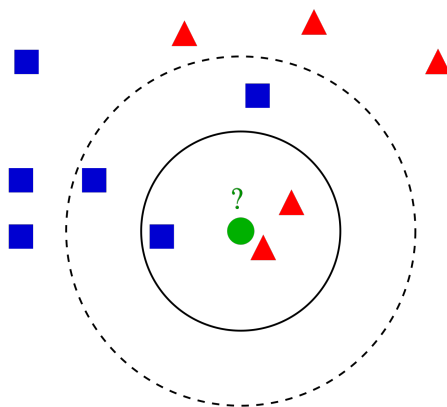
Σχήμα 4.15: Απεικόνιση της λειτουργίας του αλγορίθμου k NN. Ανάλογα με τον καθορισμό του k , το μοντέλο θα ταξινομήσει το δείγμα (πράσινη κουκίδα) στα κόκκινα τρίγωνα ή τα μπλε τετράγωνα [16].
