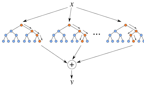
Σχήμα 4.16: Η αρχιτεκτονική και ο τρόπος λειτουργίας του Random Forest Classifier.
