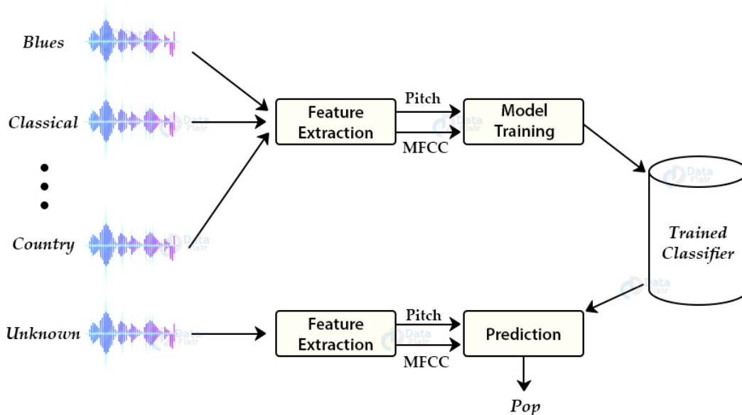
Σχήμα 3.5: Η χρήση μοντέλων μηχανικής μάθησης με σκοπό τη πρόβλεψη μουσικών ειδών και κατηγοριοποίηση κομματιών με βάση αυτά, είναι ένα ιδιαίτερα ενδιαφέρον σκέλος έρευνας [13]. Έχει ουσιαστικό νόημα η χρήση του machine learning ή πρόκειται για ένα πρόβλημα που χρήζει άληθης λύσης;
