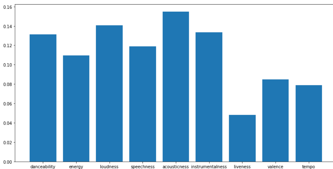
Σχήμα 6.2: Ιστόγραμμα σπουδαιότητας μελωδικών χαρακτηριστικών του κεντρικού dataset, μέσω του κατηγοριοποιητή XGBoost.
