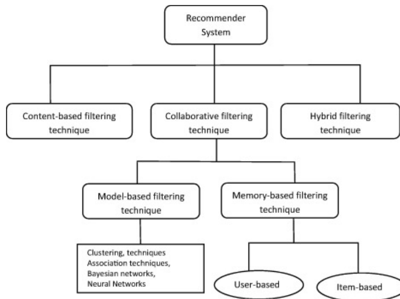
Σχήμα 2.4: Σήμερα, τρεις εκ των προαναφερθεισών κατηγοριών recommenders χαίρουν υιοθέτησης και ενδιαφέροντος. Τα content-based συστήματα, η δημοφιλής collaborative filtering τεχνική και ο φουτουριστικός hybrid συνδυασμός υλοποιήσεων είναι οι κατηγορίες που έχουν ξεχωρίσει [5].
