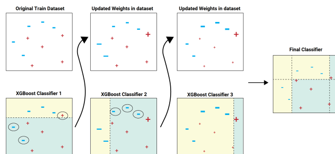
Σχήμα 4.18: Απεικόνιση του τρόπου με τον οποίο δρα ο XGBoost, ενισχύοντας την απόδοση των κλασικών gradient boosting μοντέλων και βελτιώνοντας το τελικό αποτέλεσμα [18].
