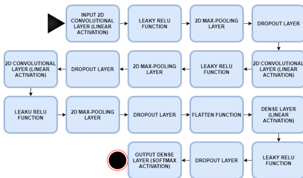
Σχήμα 4.19: Η αποτύπωση της διάταξης των επιπέδων στο δημιουργηθέν 2d convolutional νευρωνικό δίκτυο για το μουσικό σύνολο δεδομένων μας.
