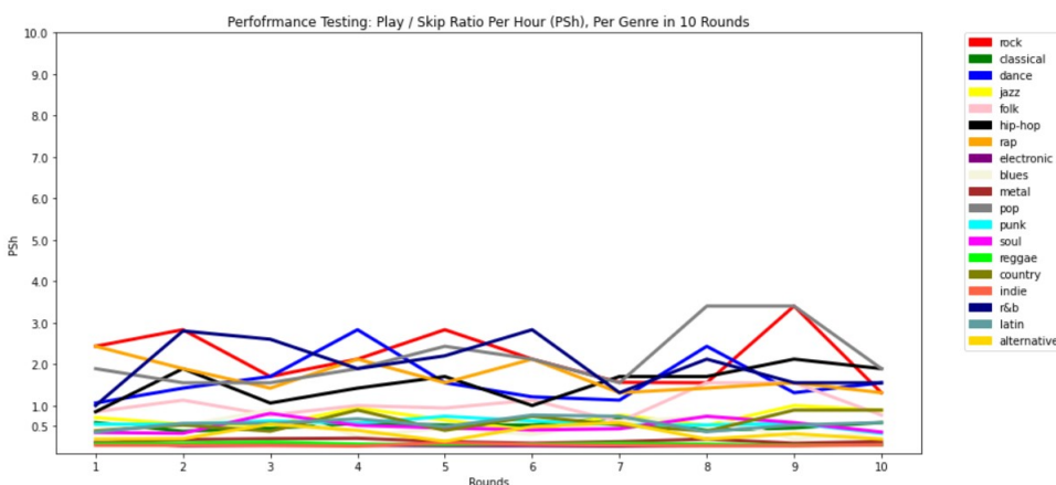
Σχήμα 6.9: Διάγραμμα Play / Skip Ratio Ανά Ώρα (PSh) “μεσαίου” συνόλου.
