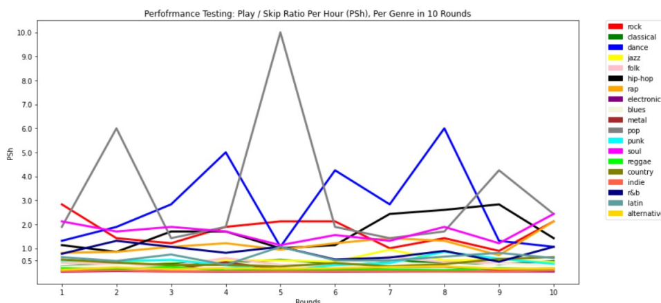
Σχήμα 6.8: Διάγραμμα Play / Skip Ratio Ανά Ώρα (PSh) “μικρού” συνόλου.
