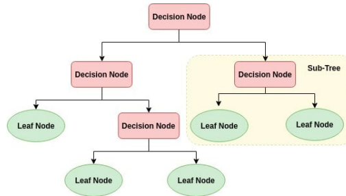
Σχήμα 4.17: Τα δέντρα αποφάσεων και η λειτουργία μέσω της οποίας προχωρούν στην ταξινόμηση των χαρακτηριστικών [17].
