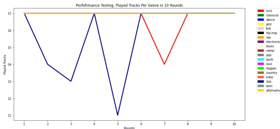
Σχήμα 6.5: Διάγραμμα Συνολικών Αναπαραγωγών “μεσαιού” συνόλου.
