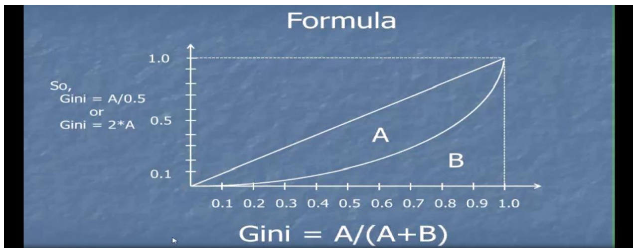
Εικόνα 2.2 . Δείκτης gini
