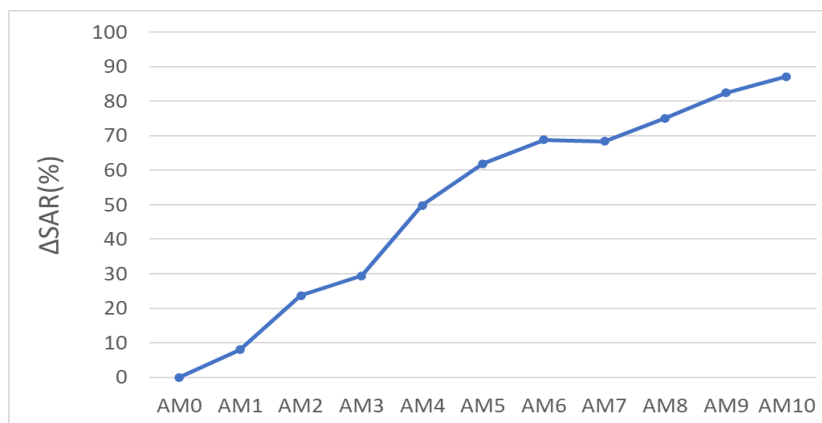
Εικόνα 5.12 Μείωση SAR-HMMPA f=3.6\text{GHz}
