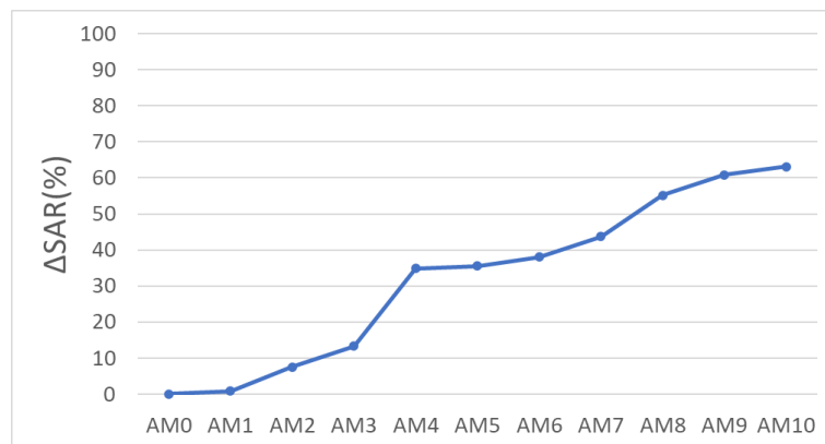
Εικόνα 5.3 Καμπύλη μείωσης SAR-για την HMMPA στα f=2.4\text{GHz}
