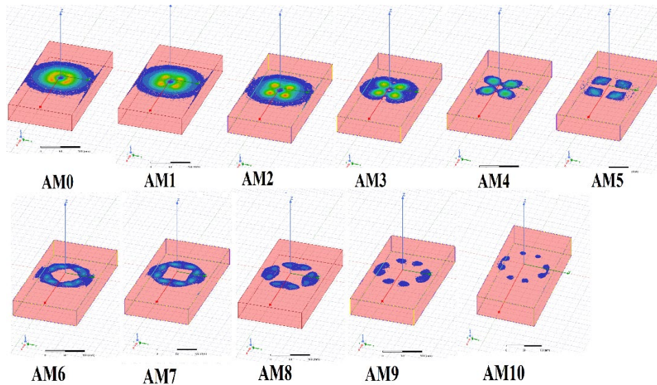
Εικόνα 5.13 Μείωση SAR για την HMPA επάνω στο ομοίωμα στα f=3.6 GHz
