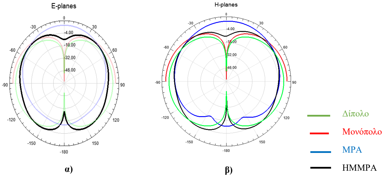
Εικόνα 2.27: Συγκριτικά Διαγράμματα Ακτινοβολίας στον ελεύθερο χώρο α) \varphi=0^\circ β) \varphi=90^\circ
