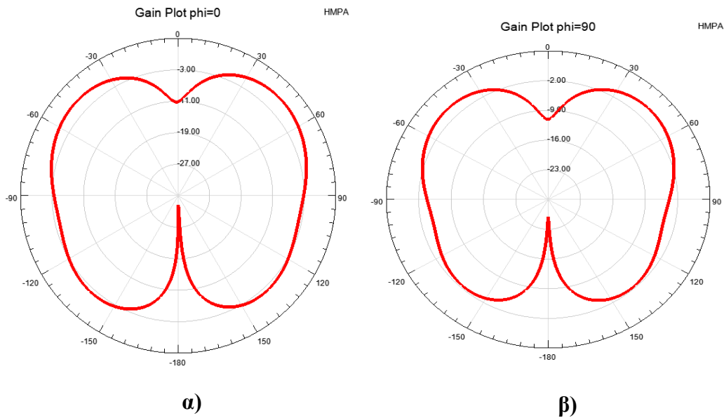
Εικόνα 2.26: Διαγράμματα ακτινοβολίας για ΗΜΜΡΑ στα f=3.6\text{ GHz} α) \varphi=0^\circ β) \varphi=90^\circ
