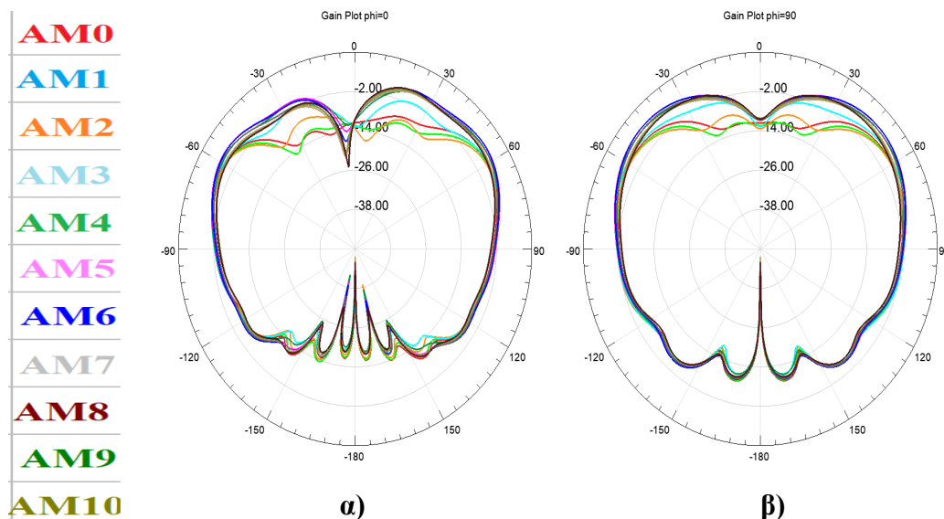
Εικόνα 5.11 Διαγράμματα Ακτινοβολίας για AM1-AM10 με phantom f=3.6\text{GHz} α) \varphi=0^\circ β) \varphi=90^\circ
