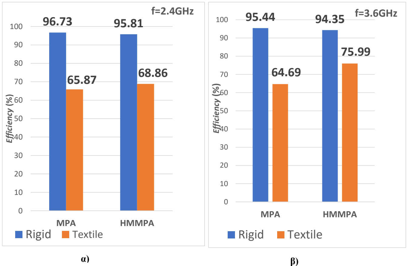
Εικόνα 2.28: Απόδοση Ακτινοβολίας με άκαμπτα και εύκαμπτα υλικά α) f=2.4\text{GHz} β) f=3.6\text{GHz} υψηλότερου συντελεστή απωλειών που έχουν τα εύκαμπτα υλικά. Αντίστοιχα για την συχνότητα f=3.6\text{GHz} , η μείωση στην απόδοση ακτινοβολίας για την κεραία MPA είναι 30.75%, αντίστοιχα με την συχνότητα f=2.4\text{GHz} , ενώ για την HMMPA είναι λιγότερο, κοντά στο 18.6%.
