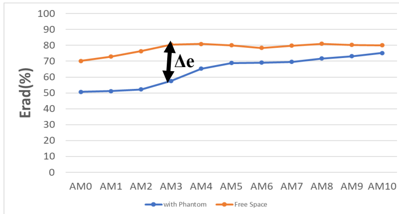
Εικόνα 5.5 Απόδοση Ακτινοβολίας στον Ελεύθερο Χώρο και με Ομοίωμα στα f=2.4\text{GHz}
