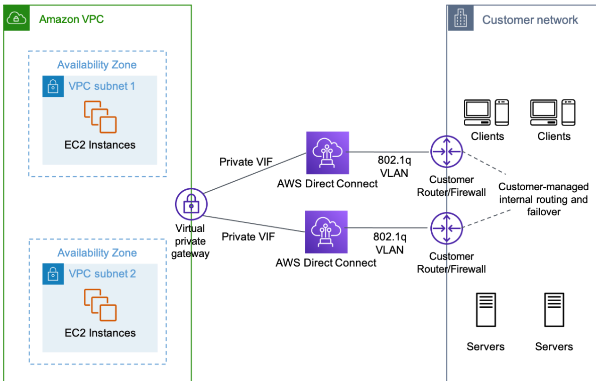
Εικόνα 28 : AWS redundant Direct Connect
